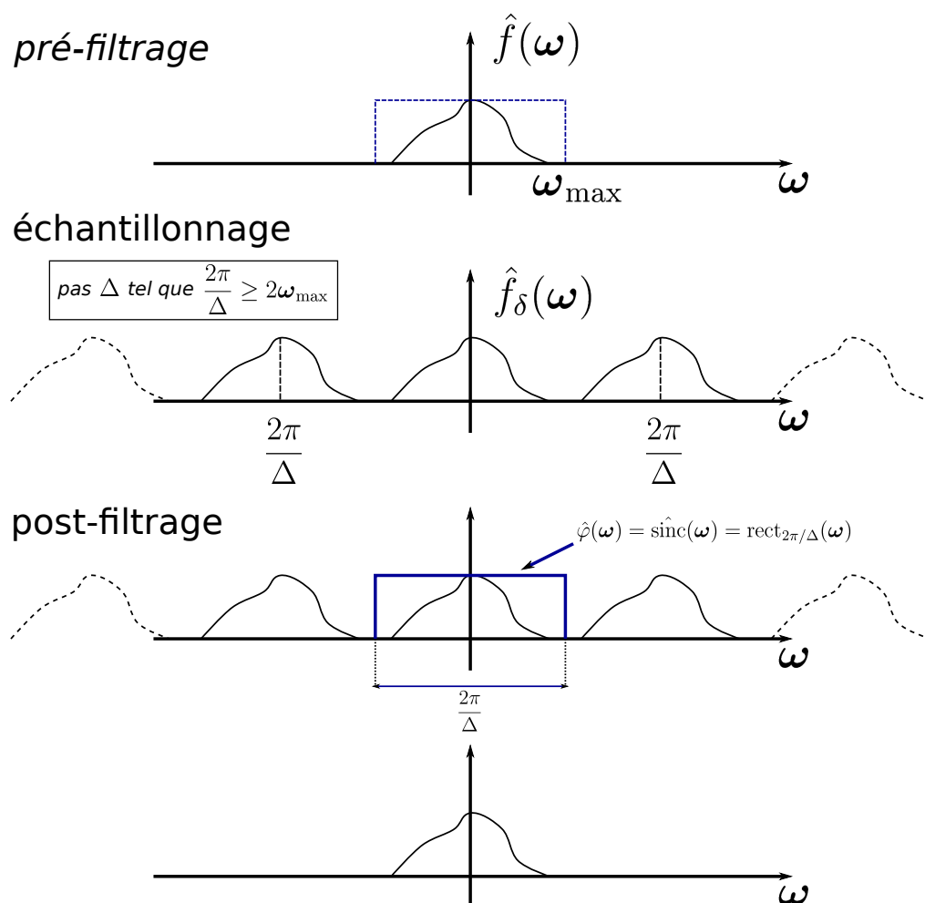
FIGURE 2.3: Schéma d'échantillonnage (tiré de [Unser, 2000]), dans le domaine de Fourier, selon la théorie de Shannon, s'appliquant à une fonction f à support spectral borné (fréquence maximale du spectre \omega_{\max} ). Sa transformée de Fourier est notée \hat{f}(\omega) . On retrouve les trois étapes vues dans la figure 2.2. Le pas d'échantillonnage \Delta est choisi tel que la fréquence d'échantillonnage \frac{2\pi}{\Delta} soit supérieure au double de la fréquence de Nyquist 2\omega_{\max} . L'étape d'échantillonnage revient à une périodisation du spectre. Le post-filtrage \hat{\varphi}(\omega) permet de retrouver le spectre initial. Dans la théorie de Shannon, ce filtre est idéal, c'est la fonction sinus cardinal \text{sinc}(x) dont la transformée de Fourier est la fonction porte \text{rect}_{2\pi/\Delta}(\omega) de largeur \frac{2\pi}{\Delta} qui permet la récupération parfaite du signal.
