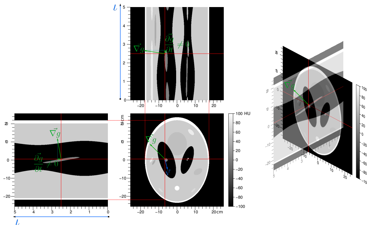
FIGURE 3.18: Illustration du gradient spatio-temporel global \vec{\nabla}g en un point du fantôme dynamique de Shepp-Logan, simulé dans le cas n° 1. La tranche temporelle en \nu = 2,5 s est représentée au centre. Les schémas périphériques montrent les différentes coupes 2-D dans la direction temporelle, i.e. des tranches spatio-temporelles (la direction temporelle est indiquée). Chacune de ces coupes est localisée sur la tranche centrale. On met ainsi en évidence la notion de frontière spatio-temporelle de l'objet, indiquant une corrélation entre les tranches.
