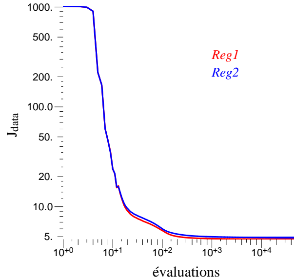
FIGURE 3.40: Convergence du terme d'attache aux données J_{\text{data}} (cf. équation 3.28), en fonction du nombre d'évaluations, de deux reconstructions régularisées respectivement avec Reg1 (en rouge) et Reg2 (en bleu), pour les mêmes poids \mu_{\text{space}} et \mu_{\text{time}} .
