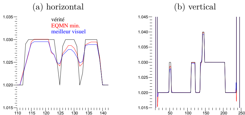
FIGURE 1.36: Visualisation des profils de coupes horizontale (a) et verticale (b), identifiés sur la figure 1.21(b), pris sur les reconstructions de la figure 1.30, la reconstruction donnant l'erreur EQMN minimale dans la ROI (rouge), et la reconstruction de meilleure qualité visuelle empirique (bleu). Le profil de référence est de couleur noire.
