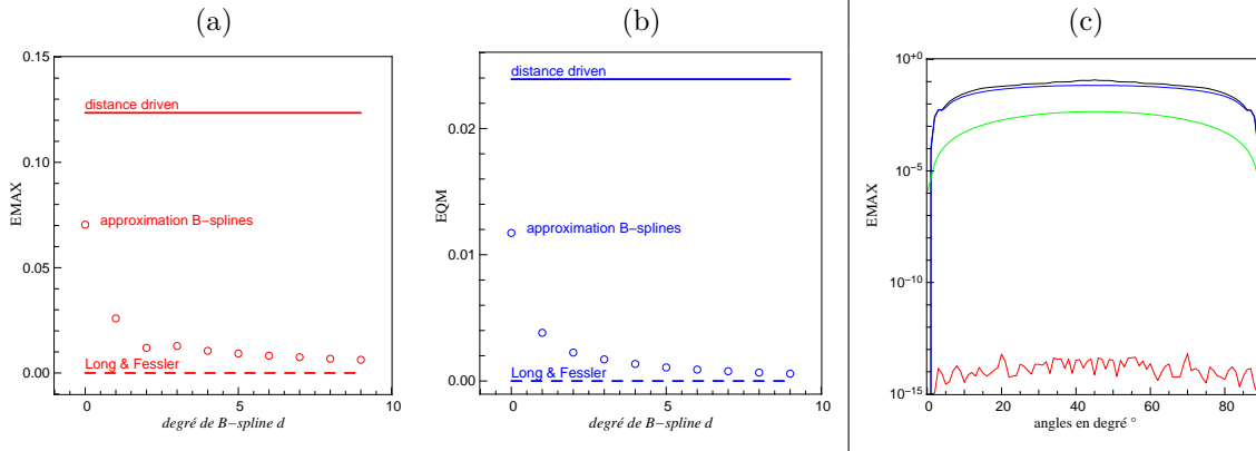
FIGURE 2.35: Évolution de l'erreur maximale EMAX (a) et de l'erreur quadratique moyenne EQM (b) en fonction du degré d de B-spline utilisé pour notre modèle, comparé à celles des modèles distance driven (en trait plein sur chaque graphe) et L&F (en trait pointillé sur chaque graphe). La projection est réalisée pour un détecteur incliné à 45^\circ par rapport au plan horizontal. En (c) : erreur d'approximation maximale, en propagation parallèle, en fonction de l'inclinaison du détecteur, allant de 0^\circ à 90^\circ , pour le modèle distance driven (noir), le modèle L&F (rouge), notre modèle avec indicatrice de voxel (bleu) et avec B-spline cubique (vert).
