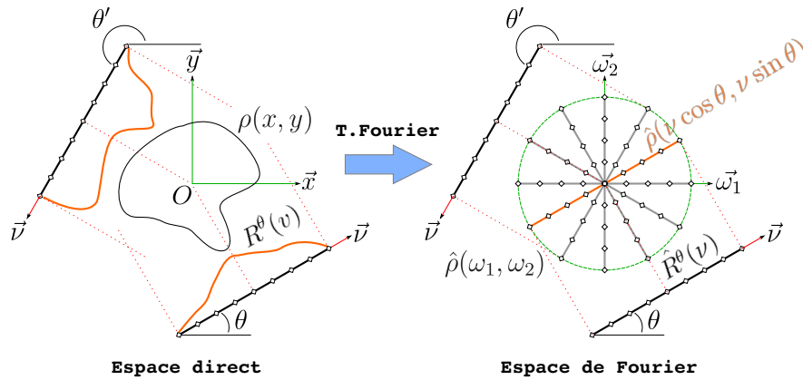
FIGURE 2.23: Illustration du théorème coupe-projection lié à la transformée de Radon 2-D standard, i.e. en géométrie standard et propagation parallèle. La transformée de Fourier \hat{R}^\theta(\nu) de la projection de Radon d'un objet 2-D sur un détecteur linéaire incliné d'un angle \theta est égale à la coupe 1-D, suivant cette même inclinaison et passant par l'origine, dans la transformée de Fourier 2-D de l'objet \hat{f}(\omega_1, \omega_2) .
