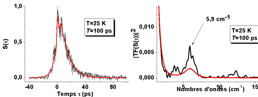
FIGURE 4.22 – Signal d'écho de photons stimulés de W(CO)_6/CH_4 à 25 K. - Pour ce signal, T=100 ps. Le signal expérimental est en noir, le modèle est en rouge. A droite : module au carré de la transformée de Fourier du signal d'écho. Voir le texte pour les paramètres du modèle.
