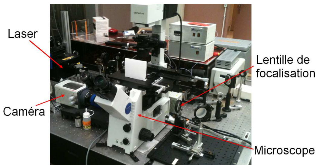
FIGURE 3.12.: Montage de microscopie à onde évanescente.
