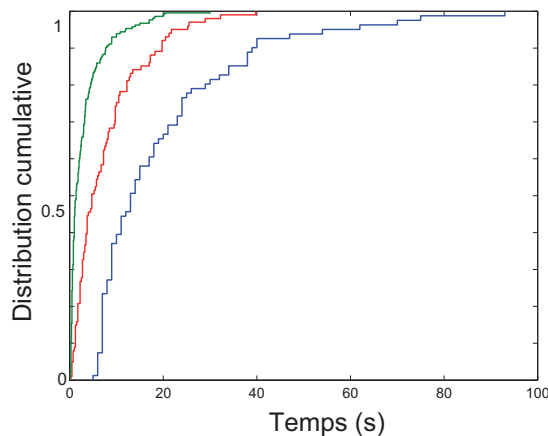
FIGURE 3.29.: Rallongement du temps de photoblanchiment par illumination stroboscopique. Fonctions cumulatives des temps de photoblanchiment aux cadences 10 images/s (vert), 2.5 images/s (rouge) et 1 image/s (bleu).
