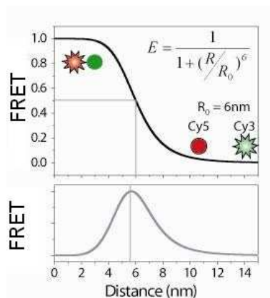
FIGURE 3.38.: Efficacité du FRET pour le couple Cy3 et Cy5 en fonction de la distance entre les fluorophores. Extrait de [Sel07].
