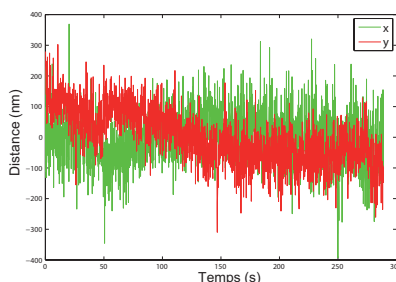
FIGURE 4.1.: Suivi de la position d'un Qdot en fonction du temps. L'écart type des déplacements calculés est égal à 96 nm sur chaque axe. L'erreur sur la position du QDot est égale à 2 nm.
