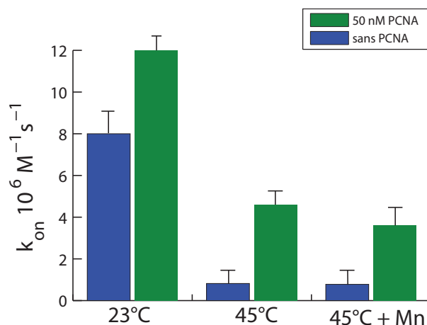
FIGURE 5.4.: Taux d'association de NucS avec le substrat 5bf5 en fonction de la température et de la concentration en \text{Mn}^{2+} .
