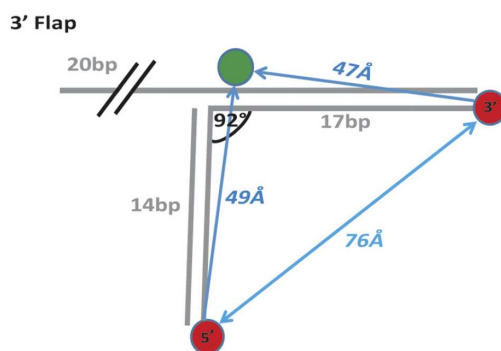
FIGURE 5.18.: Mesure de FRET du complexe NucS-ADN-PCNA dans le cas d'un flap 3'. NucS est montrée en vert et les deux extrémités du substrat en rouge. Le modèle de pliage à la jonction implique la présence de NucS en amont du flap. Extrait de [Cre12].
