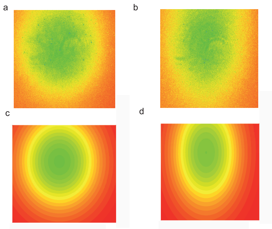
FIGURE 3.19.: Profil d'intensité du laser. a) en épifluorescence. b) en onde évanescente. c) l'ajustement 2D aboutit à un diamètre de 37.2 \pm 0.4 \mu\text{m} et une ellipticité de 0.09. d) l'ajustement 2D aboutit à un diamètre à mi-hauteur de 78.4 \pm 0.7 \mu\text{m} pour une ellipticité de 0.38.
