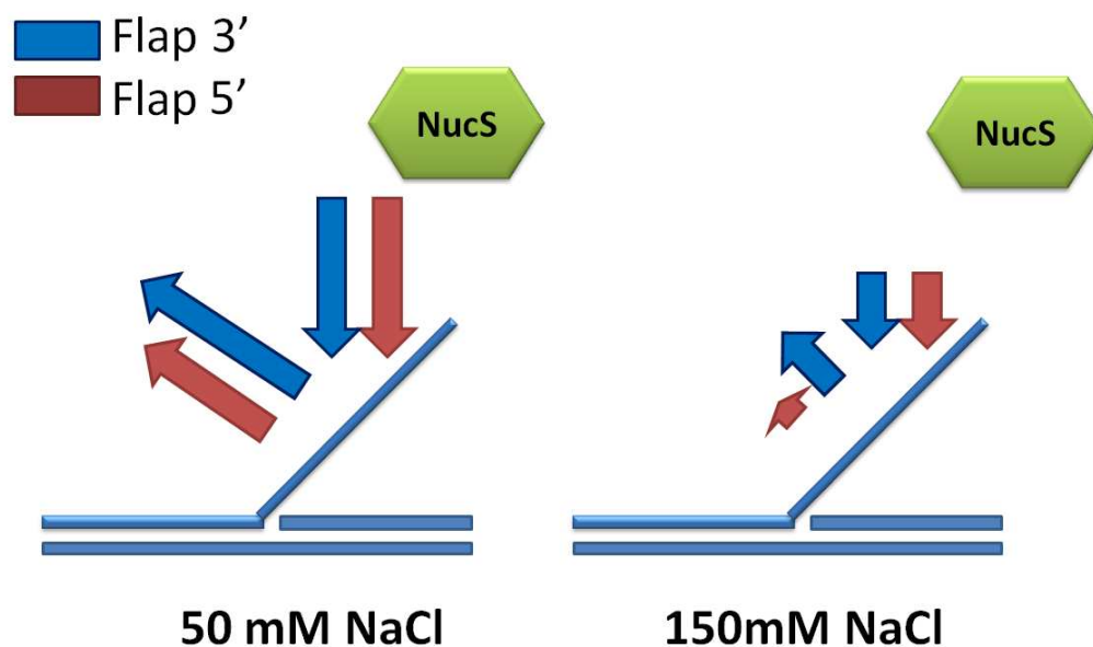
FIGURE 4.11.: Cinétique d'association et de dissociation de NucS avec le flap 3' et 5'. La longueur de la flèche est indicative de la valeur du taux d'association et de dissociation.
