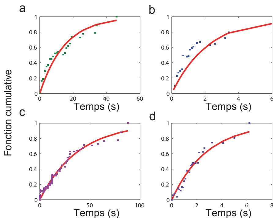
FIGURE 4.9.: Distribution des probabilités de dissociation du complexe NucS-ADN. a. et b. Flap 3' à 150 mM et 50 mM de NaCl, respectivement. c. et d. Flap 5' à 150 mM et 50 mM de NaCl, respectivement.
