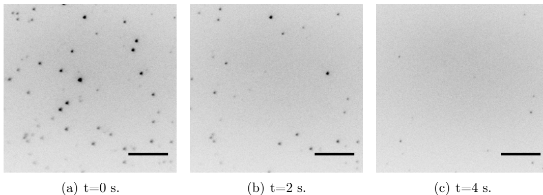
FIGURE 3.22.: Photoblanchiment du Fluorophore Alexa 488. Observation en microscopie à onde évanescente de molécules uniques d'Alexa 488. P=400 \text{ W/cm}^2 , échelle= 10 \text{ }\mu\text{m} .
