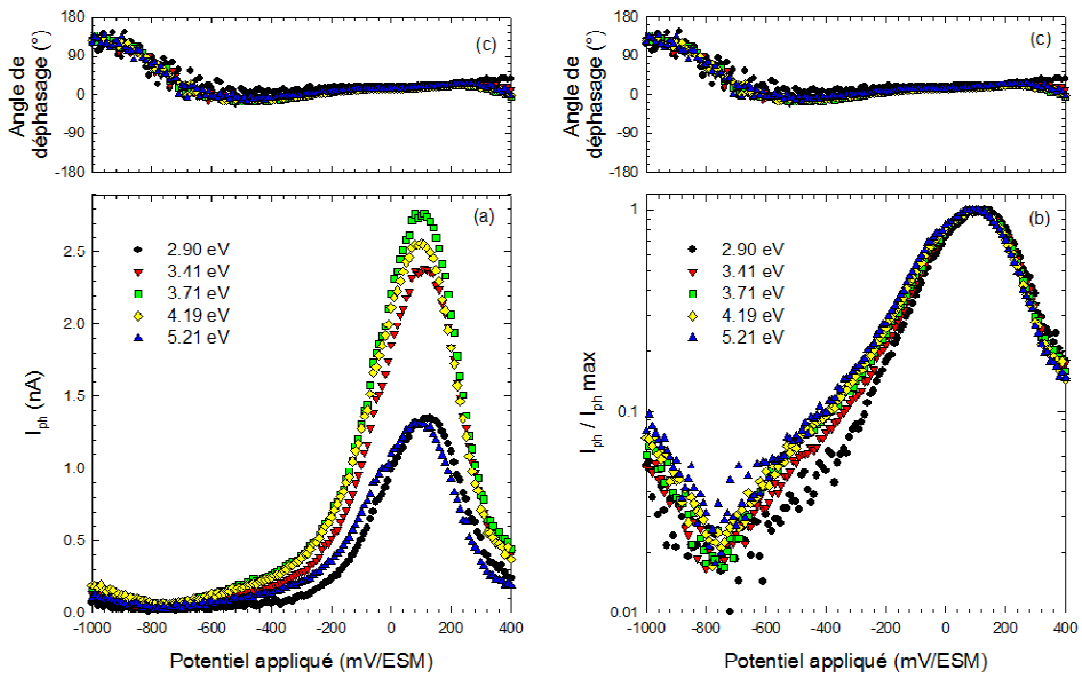
Figure III.9 : Photocaractéristiques en potentiel aux hautes énergies, 2,90 \leq E \leq 5,21 eV, de l'alliage 600, de polissage 1\text{ }\mu\text{m} diamant, oxydé en eau primaire simulée (autoclave en titane pendant 500 heures) à P(\text{H}_2) = 0,3 bar.
