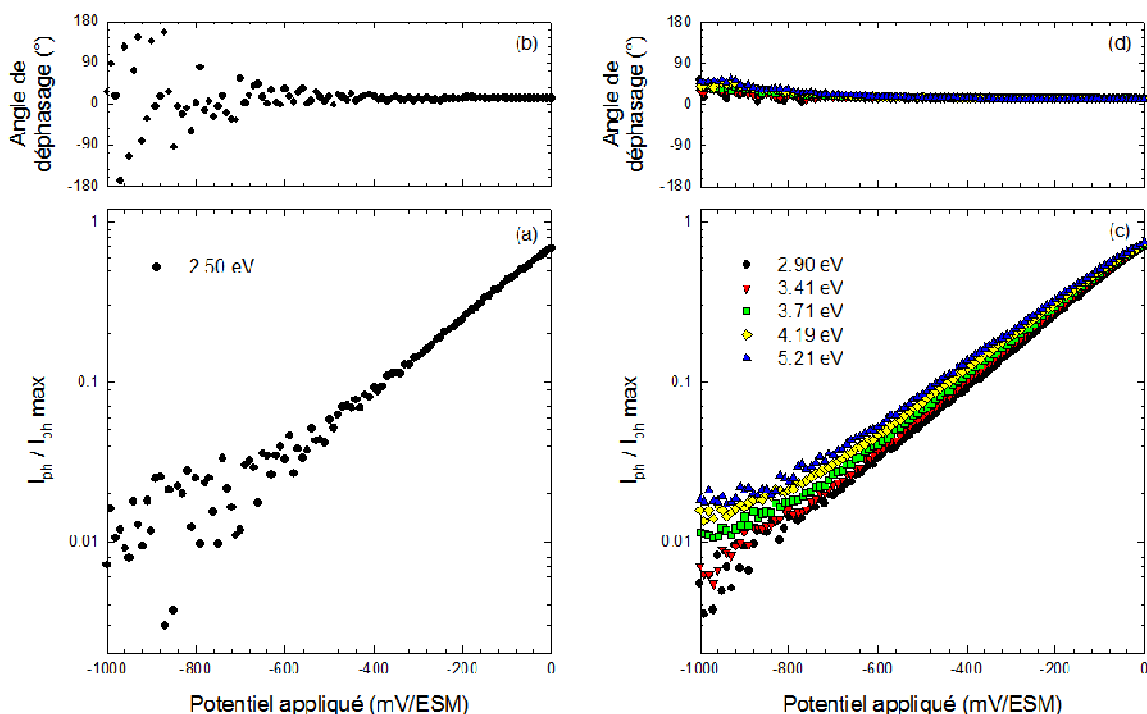
Figure III.19 : Photocaractéristiques en potentiel de l'alliage 600, de polissage 1 \mu m diamant, oxydé en eau primaire simulée (autoclave en titane pendant 500 heures) à P(H_2) < 0,01 bar.
