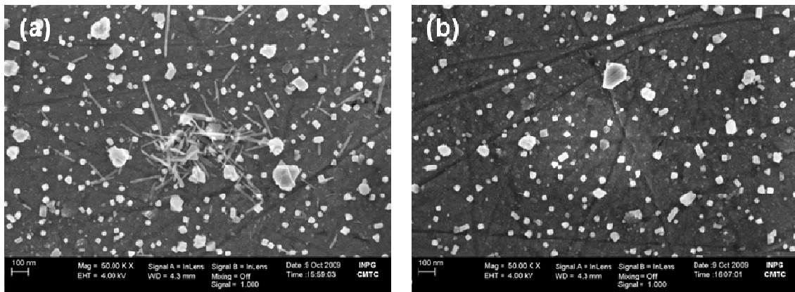
Figure II.10 : Observations au MEB-FEG de la couche d'oxydes formée sur l'alliage 600 (coulée WF675), de polissage 1\ \mu\text{m} diamant, oxydé en eau primaire simulée (autoclave en titane pendant 500 heures) à P(H_2) = 6,5 bar.
