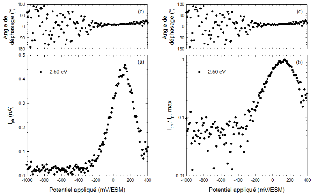
Figure III.8 : Photocaractéristiques en potentiel à basse énergie, E = 2,50 eV, de l'alliage 600, de polissage 1\text{ }\mu\text{m} diamant, oxydé en eau primaire simulée (autoclave en titane pendant 500 heures) à P(\text{H}_2) = 0,3 bar.
