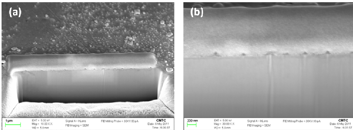
Figure II.17 : Observations au MEB-FEG d'une coupe transverse, préparée par FIB, de l'alliage 600, de polissage 1\ \mu\text{m} diamant, oxydé en eau primaire simulée (autoclave en titane pendant 500 heures) à P(\text{H}_2) = 6,5\ \text{bar} .
