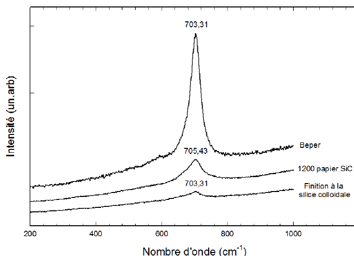
Figure II.23 : Spectres Raman obtenus pour les couches d'oxydes formées sur l'alliage 600, oxydé en eau primaire simulée (autoclave en titane pendant 500 heures) à P(\text{H}_2) = 0,3 \text{ bar} avec différents états de surface.
