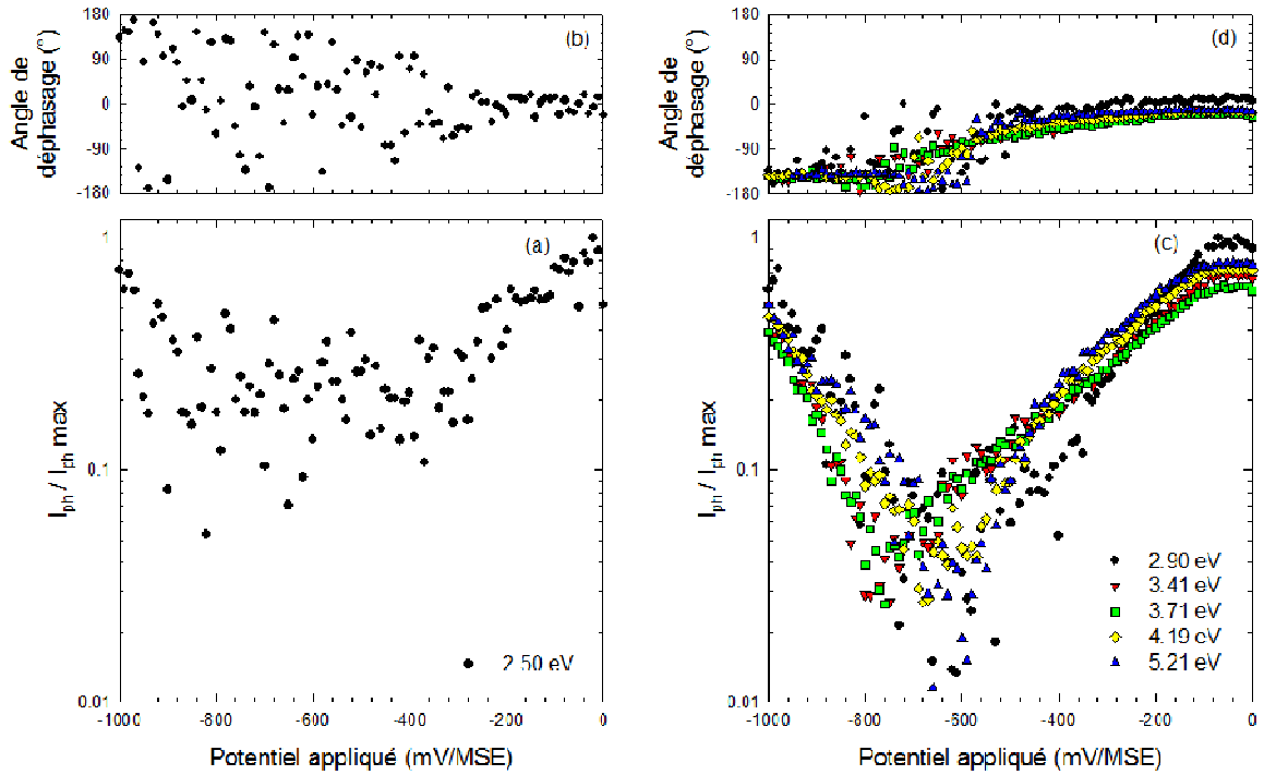
Figure III.22 : Photocaractéristiques en potentiel de l'alliage 690, de polissage 1 \mu\text{m} diamant, oxydé en eau primaire simulée (autoclave en titane pendant 500 heures) à P(\text{H}_2) = 6,5 \text{ bar} .
