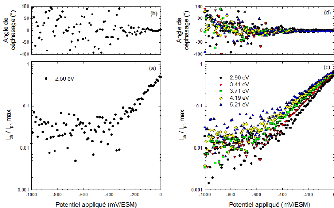
Figure III.35: Photocaractéristiques en potentiel de l'alliage 600, de polissage 1\ \mu\text{m} diamant, oxydé en eau primaire simulée (autoclave en acier inoxydable) à P(\text{H}_2) = 0,3\ \text{bar} pendant 4500 heures.
