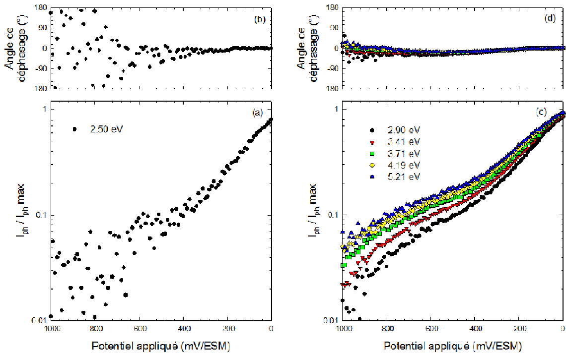
Figure III.23 : Photocaractéristiques en potentiel de l'alliage 690, de polissage 1 \mu\text{m} diamant, oxydé en eau primaire simulée (autoclave en titane pendant 500 heures) à P(\text{H}_2) < 0,01 \text{ bar} .
