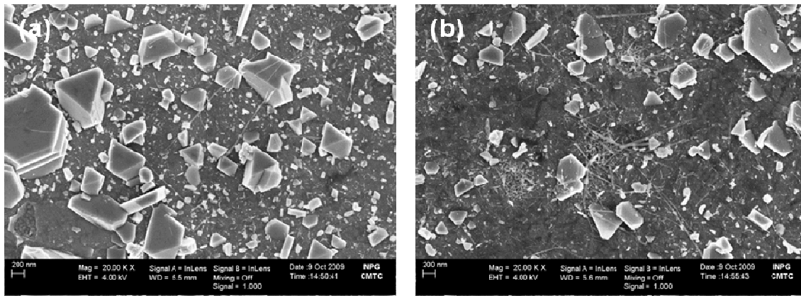
Figure II.9 : Observations au MEB-FEG de la couche d'oxydes formée sur l'alliage 600 (coulée WF675), de polissage 1\ \mu\text{m} diamant, oxydé en eau primaire simulée (autoclave en titane pendant 500 heures) à P(H_2) < 0,01 bar.
