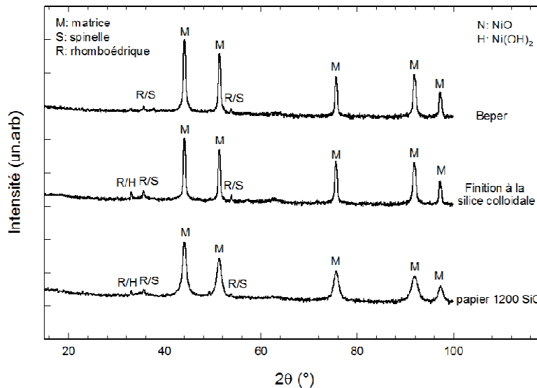
Figure II.20 : Diffractogrammes des rayons X en mode rasant obtenus pour les couches d'oxydes formées sur l'alliage 600, oxydé en eau primaire simulée (autoclave en titane pendant 500 heures) à P(H_2) = 0,3 bar avec différents états de surface.
