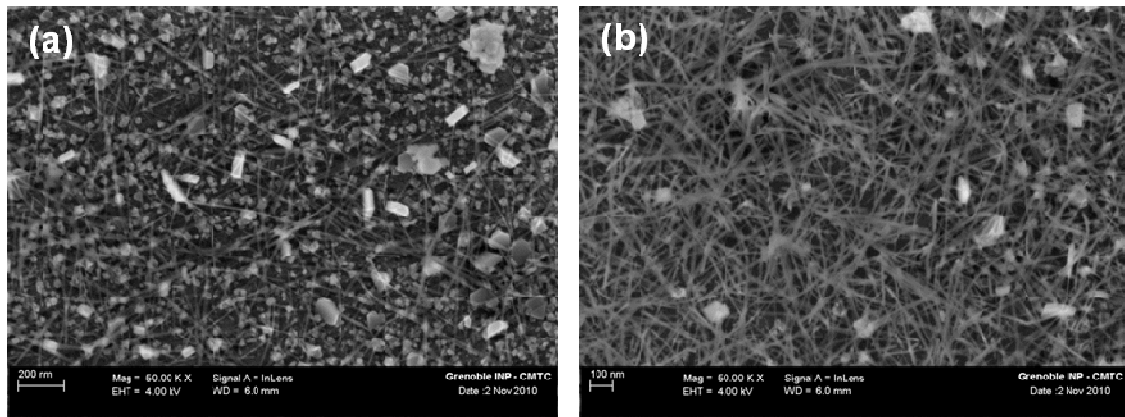
Figure II.13 : Observations au MEB-FEG de la couche d'oxydes formée sur l'alliage 600, de polissage 1 \mu\text{m} diamant avec finition à la silice colloïdale, oxydé en eau primaire simulée (autoclave en titane pendant 500 heures) à P(H_2) = 0,3 bar.
