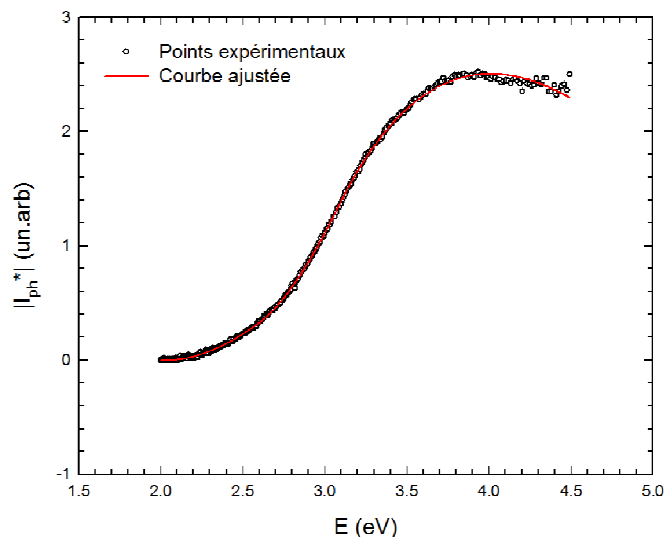
Figure III.46 : Exemple d'ajustement du photocourant, obtenu à -300 mV/ESM, pour l'alliage 600, de polissage 1\ \mu\text{m} diamant, oxydé en eau primaire simulée (autoclave en titane pendant 500 heures) à P(\text{H}_2) = 0,3 bar.
