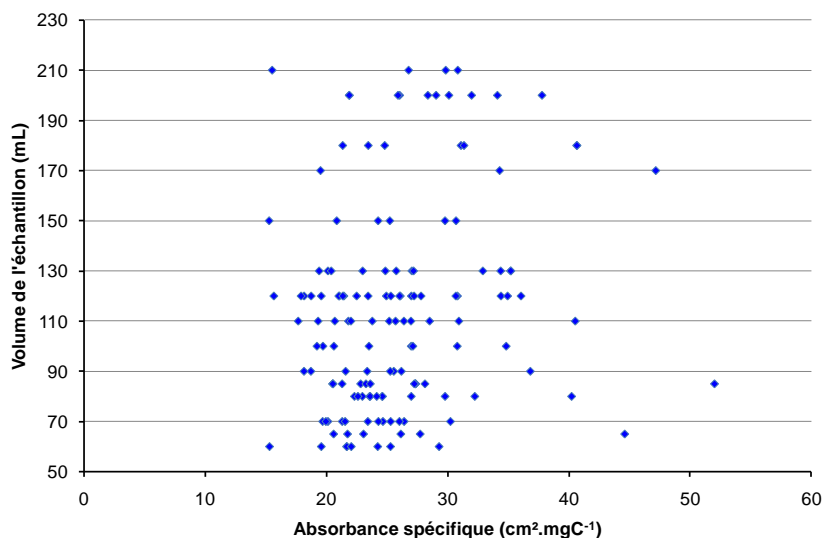
Figure 60 : Indépendance de l'absorbance spécifique (cm 2 .mgC -1 ) vis à vis du volume d'échantillon injecté (mL).
