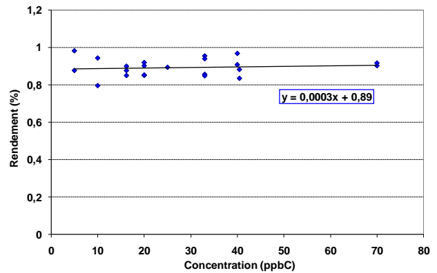
Figure 24 : Les rendements d'extraction en fonction de la concentration en acide fulvique injectée.
