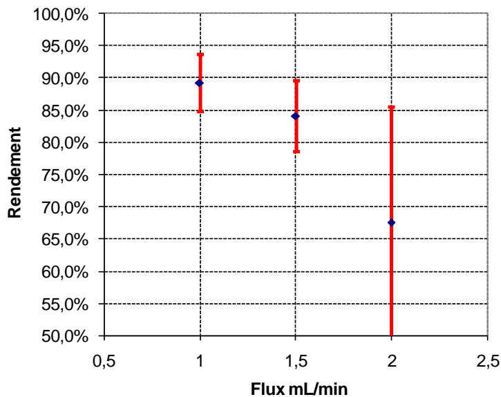
Figure 25 : Evolution du rendement d'extraction en fonction du flux d'échantillon à travers la résine.
