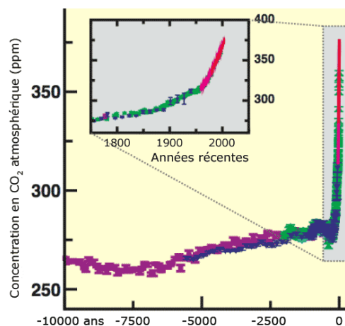
Figure 42 : Evolution de la concentration atmosphérique globale en CO 2 (ppm).
