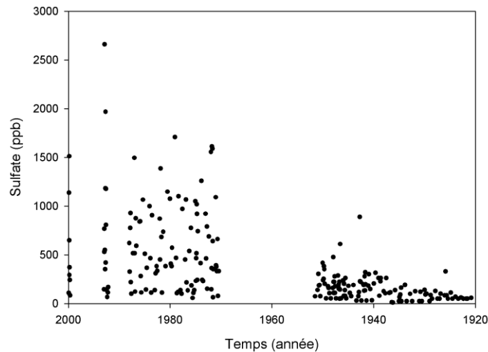
Figure 28 : Evolution de la concentration en sulfate (ppb) dans la carotte de glace du col du Dôme au cours du XX ème siècle (mesures correspondant aux échantillons d'HULIS WS de la Figure 27).
