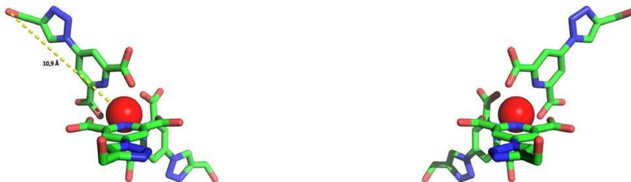
Figure 4.3 – Les deux formes énantiomères du [\text{Ln}(\text{HMTDPA})_3]^{3-}
