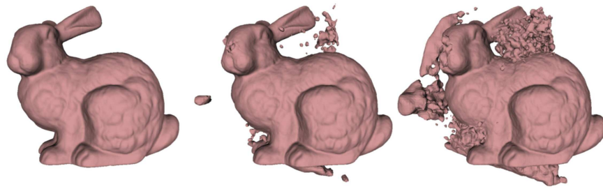
(b) Poisson
