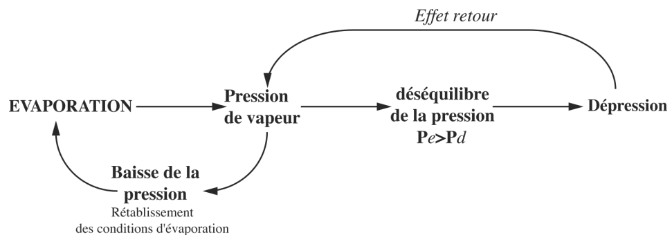
Figure 25. Les deux effets simultanés de la dépression
