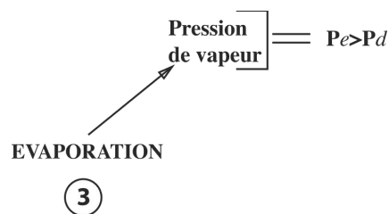
Figure 23. L'évaporation produit une pression de vapeur
