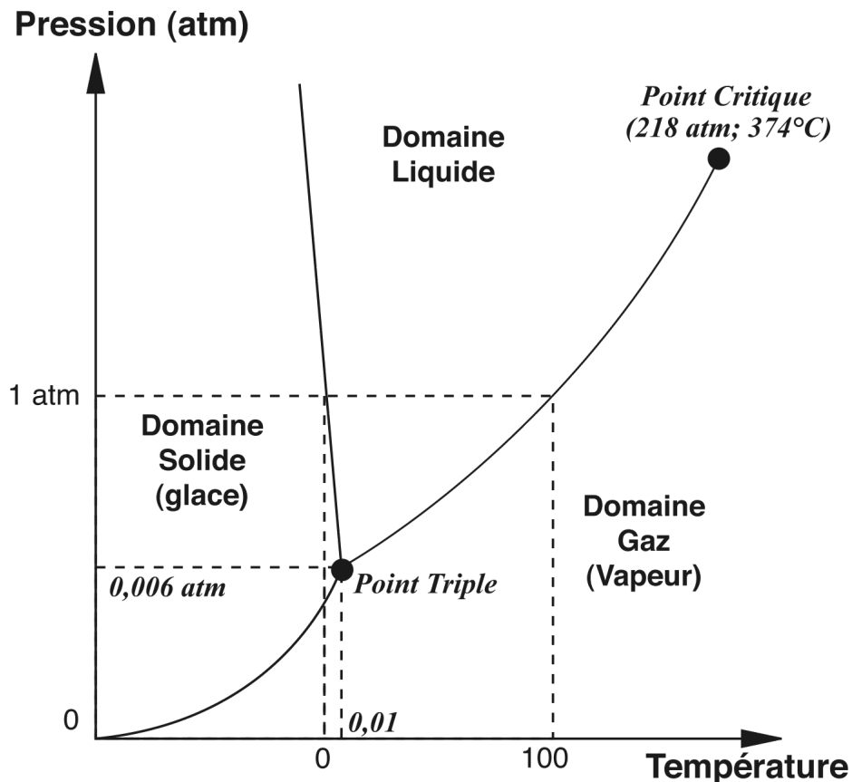
Figure 6. Diagramme des changements de phases de l'eau
