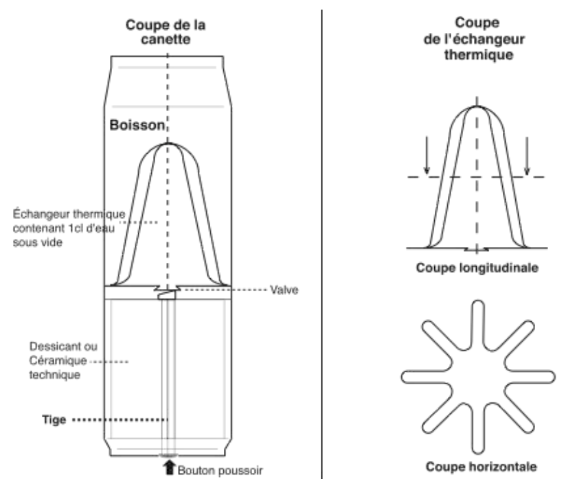
Figure 2. Schéma de la canette
