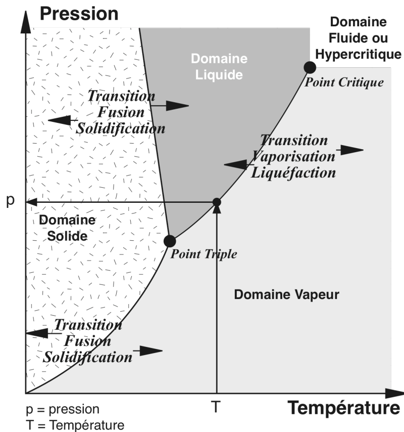
Figure 5. Diagramme général des changements de phases
