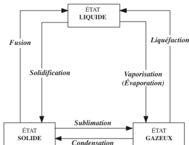
Figure 4. Schéma des six changements de phase
