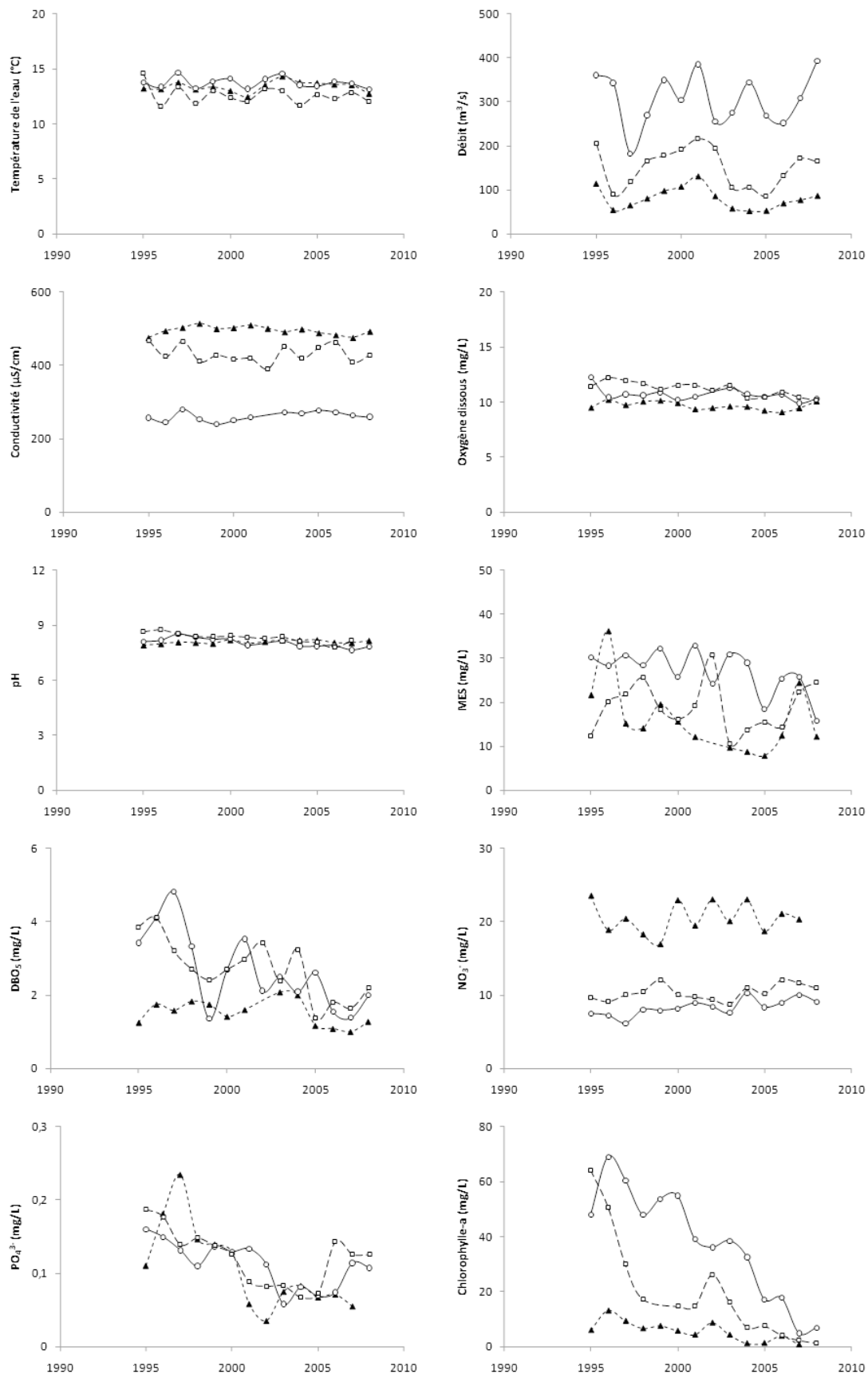
Annexe 10 : Evolutions moyennes annuelles des 10 paramètres abiotiques mesurés sur la Loire à Dampierre (cercles), sur la Seine à Nogent (triangles noirs), et sur la Meuse à Chooz (carrés) entre 1995 et 2008.
