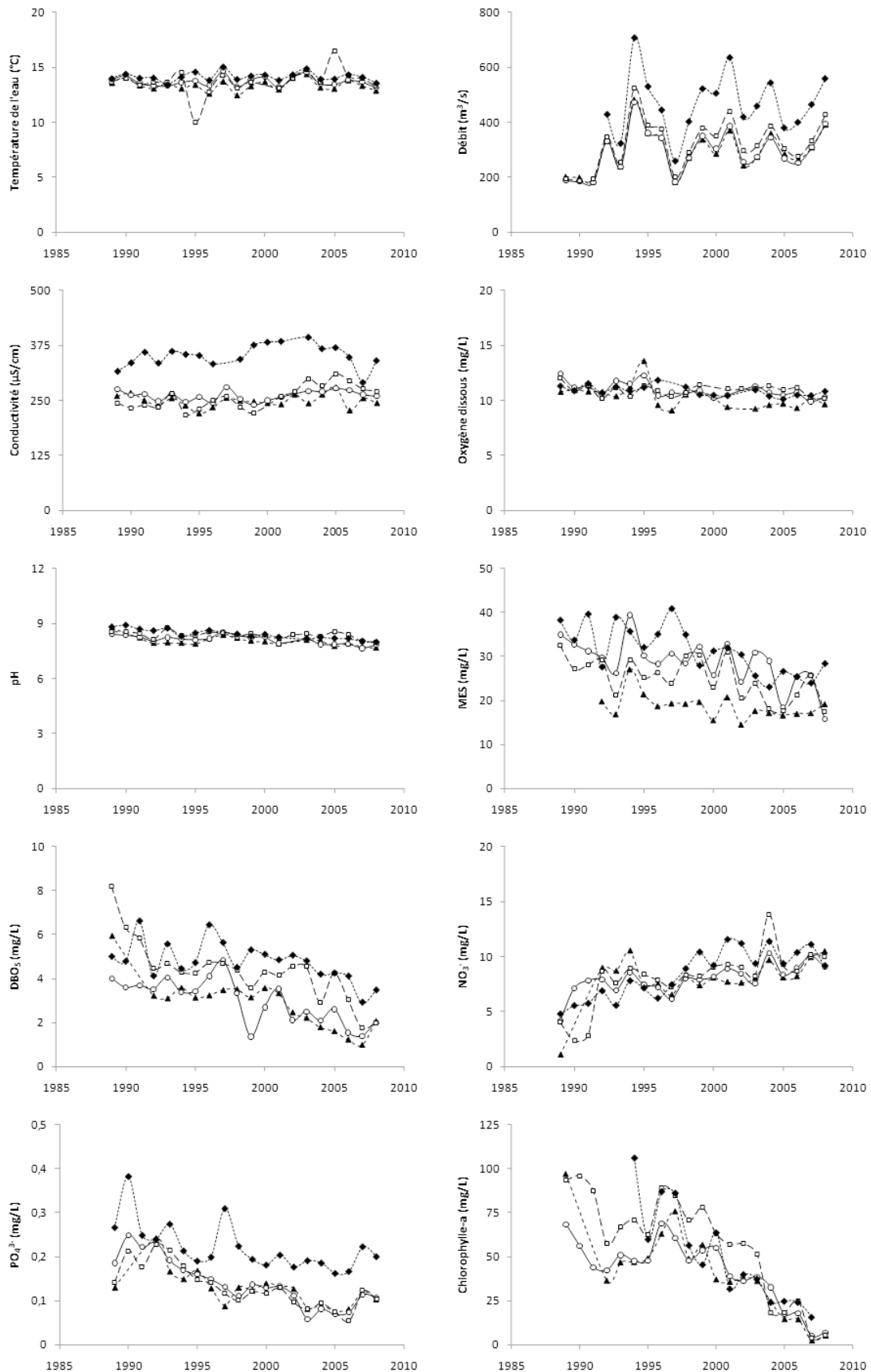
Annexe 9 : Evolutions moyennes annuelles des 10 paramètres abiotiques mesurés sur la Loire à Belleville (triangles noirs), Dampierre (cercles), Saint-Laurent (carrés) et Chinon (losanges noirs) entre 1989 et 2008.
