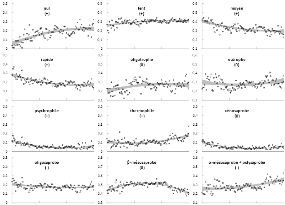
Figure 39 (suite) : Evolution temporelle des modalités des quatre traits écologiques.
