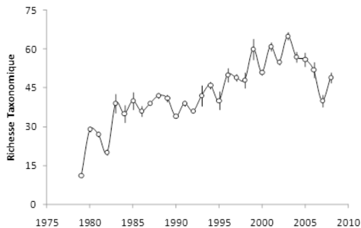
Figure 27 : Evolution long-terme de la richesse taxonomique globale (courbe noire) et saisonnière (barres d'erreur standard) à Dampierre.
