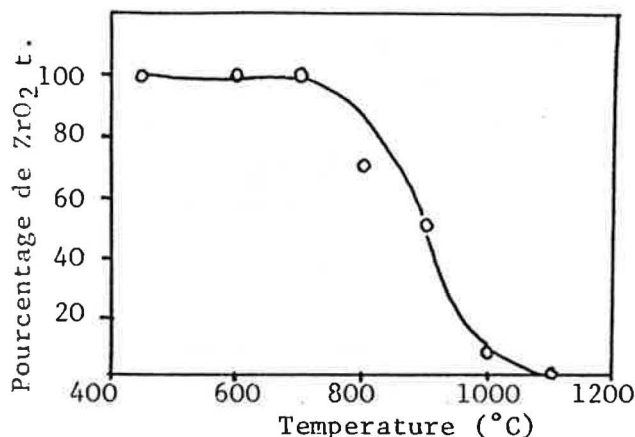
Figure IV - 7 . Evolution en fonction de la température de la teneur en ZrO_2 tétragonale (7)
