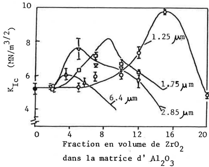
Figure VI.2 - Relation entre \sigma_F et K_{Ic} et la quantité et taille de particules de \text{ZrO}_2 dispersées (4)
