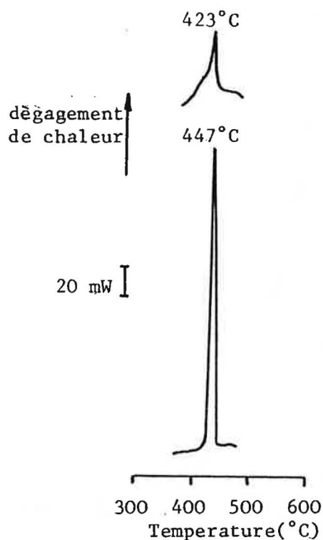
Figure V-4. Calorimétrie différentielle du <gel> après précipitation (a) et après le 6ème lavage (b)
