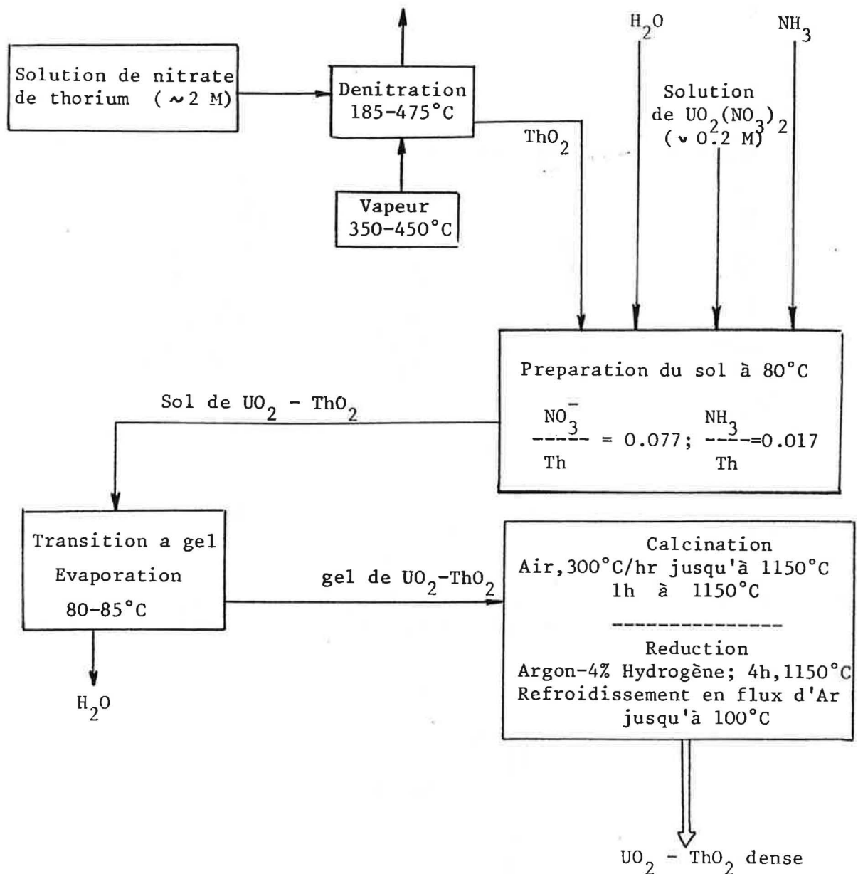
Figure VI-12. Schéma du procédé sol-gel d' Oak Ridge (9).
