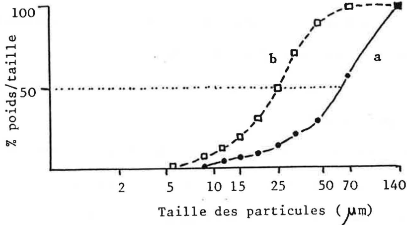
Figure VI - 18 . Distributions dimensionnelles des poudres: a) obtenue à partir d'un sol de viscosité de 400 cP; b) obtenue à partir d'un sol de viscosité de 40 cP
