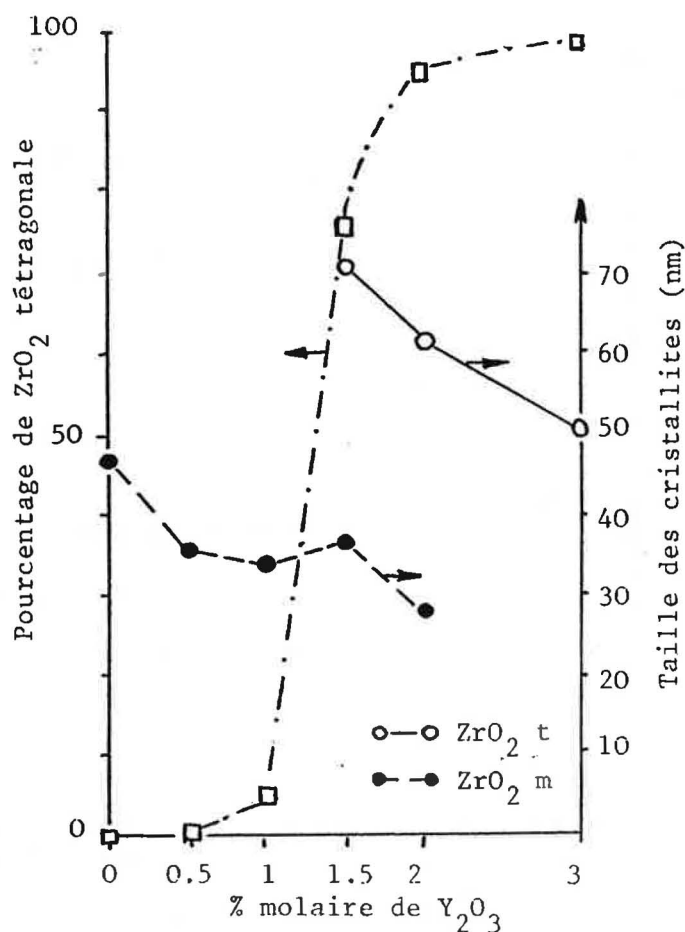
Figure V -12 . Influence d'un traitement thermique prolongé sur la pourcentage de zircone tétragonale et sur la taille moyenne des cristallite de zircone tétragonale et monoclinique
