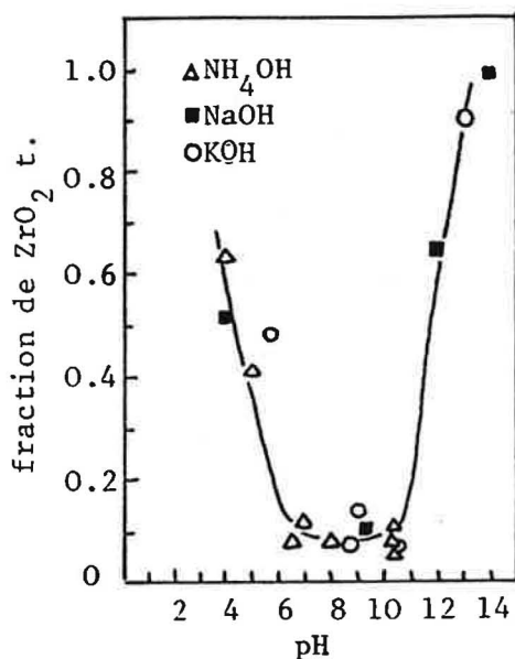
Figure IV - 5 . Proportion de zircone tétragonale obtenue à partir de gels précipités à différents pH (6)
