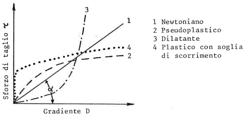
Figura III . 2 - Tipologia di comportamento reologico
