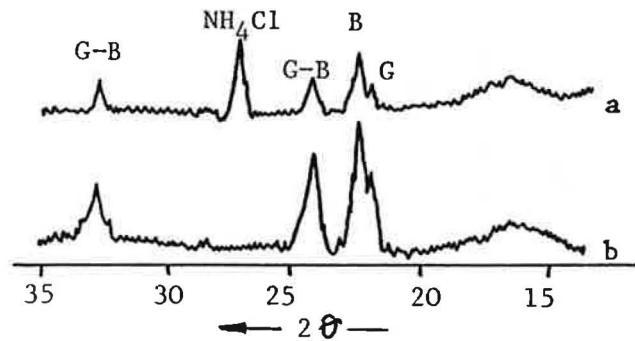
Figure VI-6 . Diagramme au Rayons X du gel ( Al_2O_3 + 15 % en poids de ZrO_2 ) séché à 105^\circ C : a) après précipitation ; b) après 7 lavages (G=gibbsite; B=bayerite)
