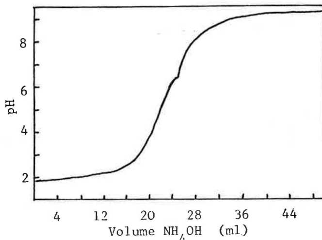
Figure IV - 3 . Courbe pH vs. volume d'agent de précipitation pour un gel ZrO_2 - Y_2O_3 (5)
