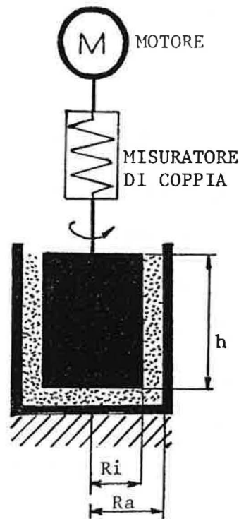
Figura III . 3 - Schema di viscosimetro a cilindri coassiali
