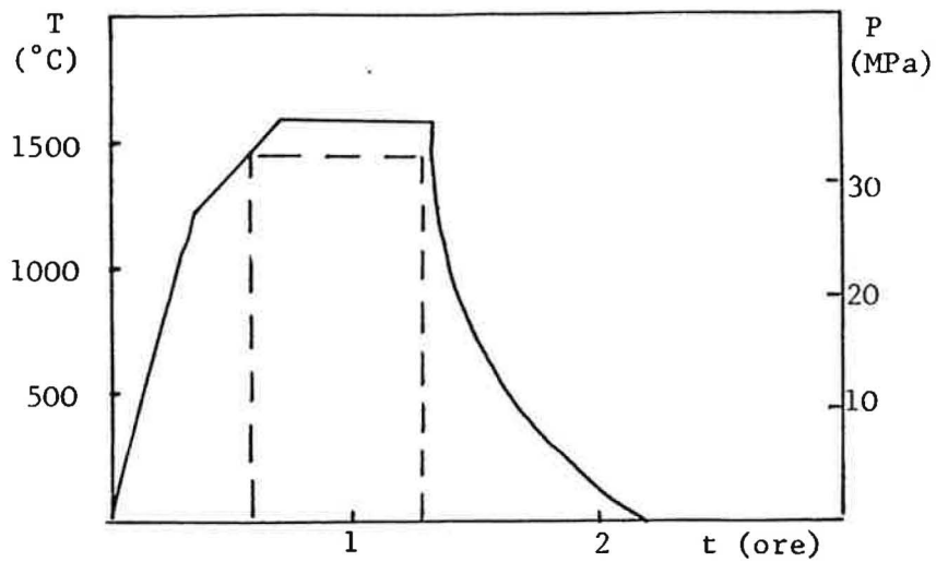
Figura III - 9. Ciclo di temperatura e pressione per la pressatura a caldo
