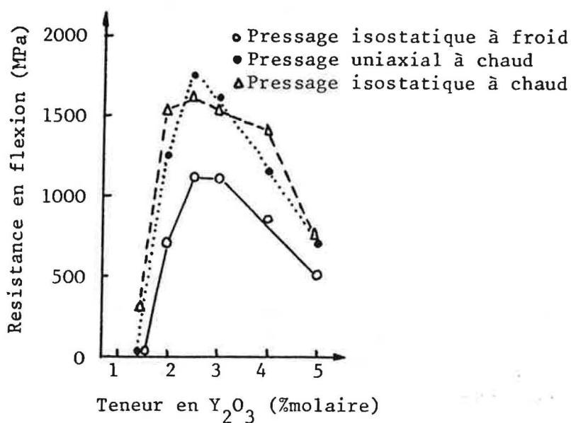
Figure II - 15 . Relation entre \sigma_F et la teneur en Y 2 O 3 des zircons yttriés (32)
