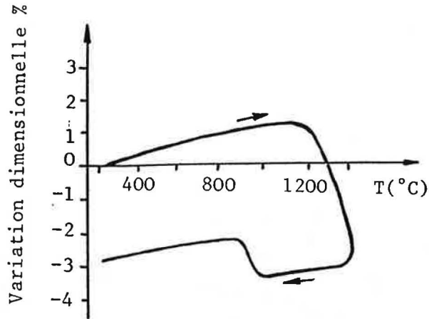
Figure II - 5 . Courbe dilatometrique d'une zircone industrielle non stabilisée (7)
