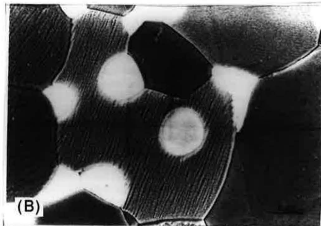
Figure II - 21. Micrographie d'un composite Al_2O_3 - 8% vol. ZrO_2 : on peut distinguer des particules de zircone à l'intérieur (intra-granulaires) et aux joints (intergranulaires) des grains de la matrice (10)
