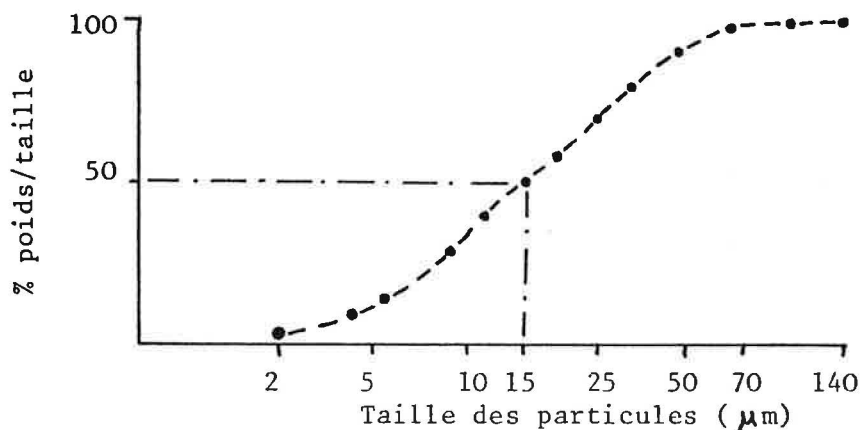
Figure VI-9 . Distribution dimensionnelle, obtenue par granulometrie laser, de la poudre d' \text{Al}_2\text{O}_3 + 15 % en poids de \text{ZrO}_2 obtenue par atomisation.
