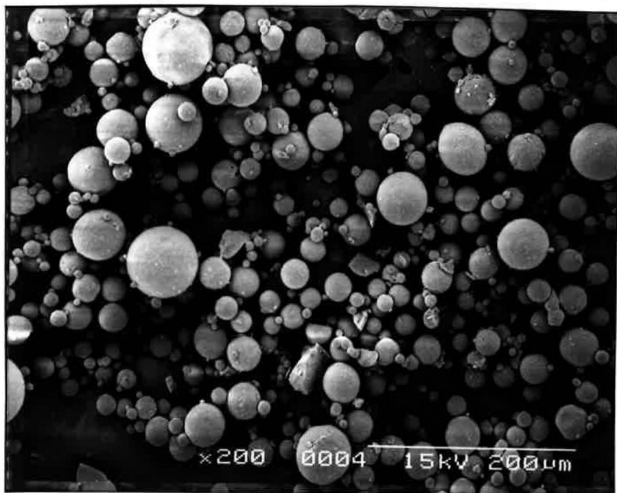
Figure VI - 19 . Micrographies au MEB des poudres obtenues à partir de sols à différente viscosité a) 400 cP; b) 40 cP
