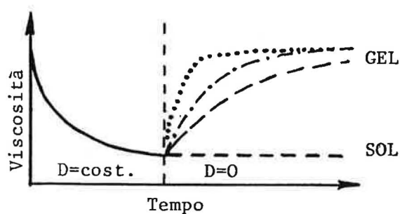
Figura III . 4 - Curva viscosità - tempo di fluidi tixotropici
