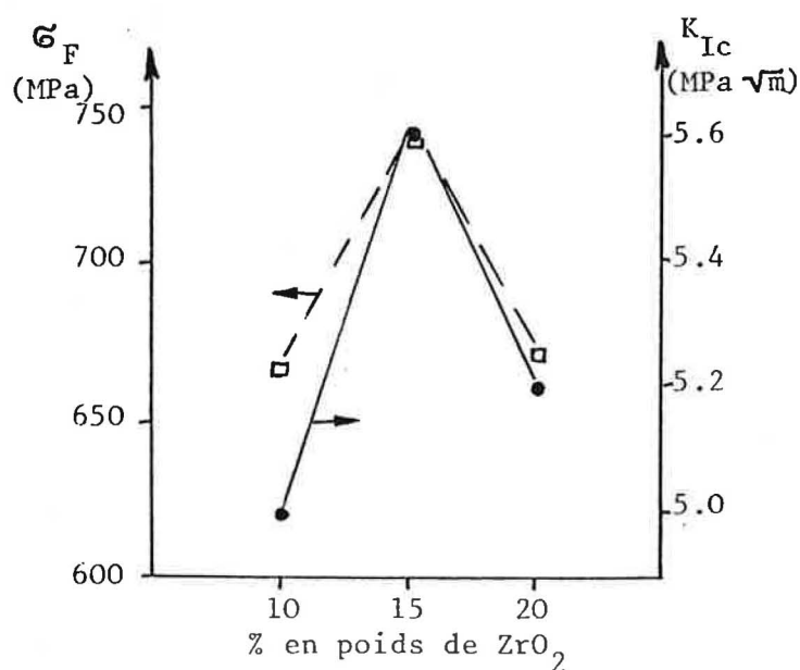
Figure VI . 11 - Variation de \sigma_F et K_{Ic} en fonction de la teneur en ZrO 2
