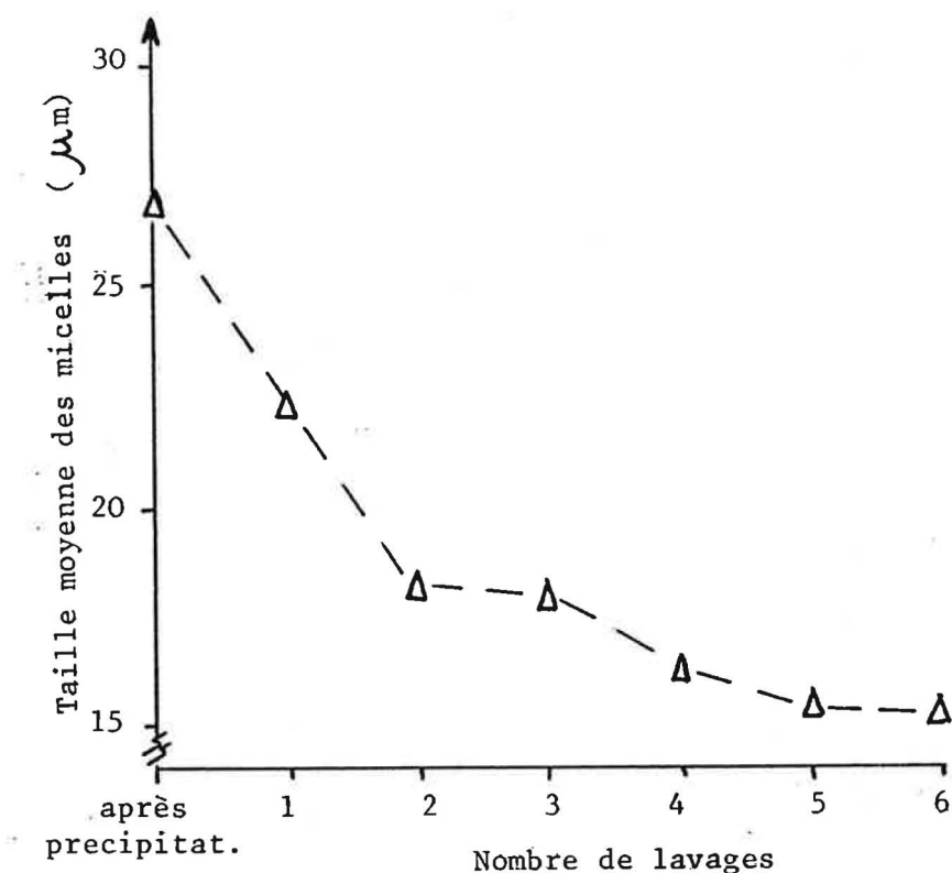
Figure V-2 . Variation de la taille des micelles du gel pendant les lavages, évaluée par granulometrie laser
