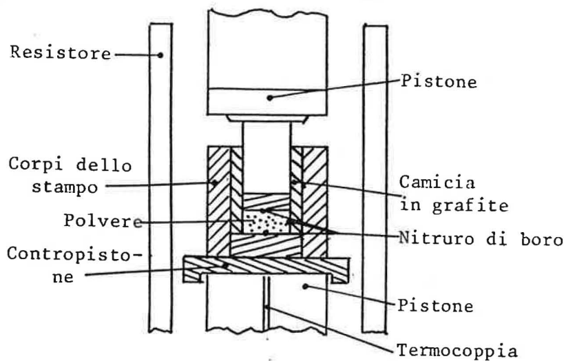
Figura III - 8. Stampo posizionato nel fornello di sinterizzazione
