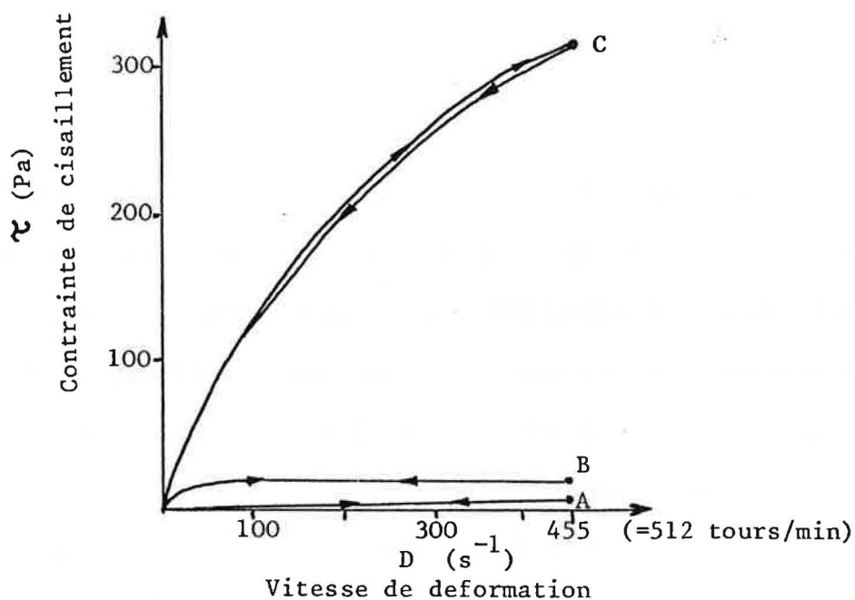
Figure VI-16 . Courbes \tau vs. D de: a) sol après peptisation b) sol après concentration jusqu'à [Al^{3+}] \approx 2M c) sol après concentration jusqu'à [Al^{3+}] \approx 5M
