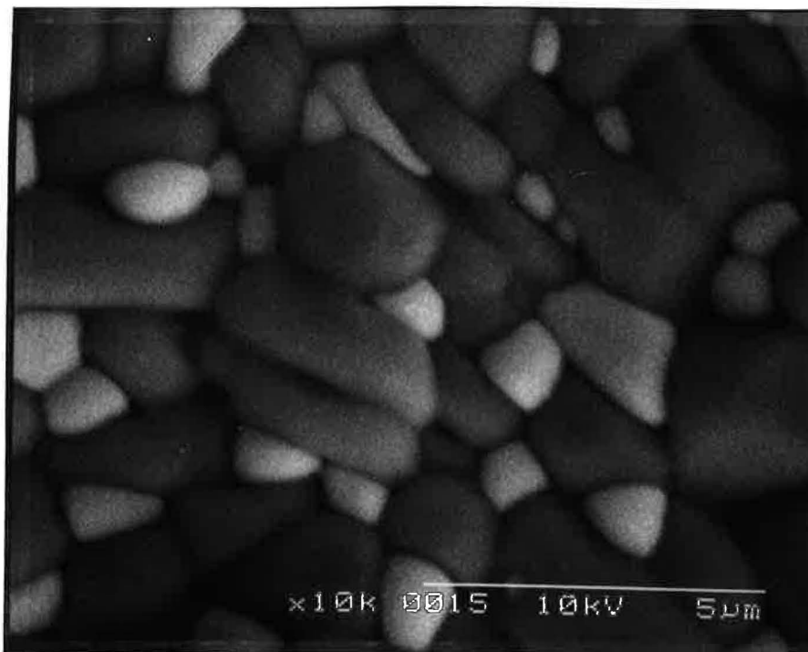
Figure VI -26 . Image au MEB en électrons retrodiffusés du composite alumine + 15% en poids de zirconie: a) obtenu à partir de la poudre atomisée b) obtenu à partir de microsphères
