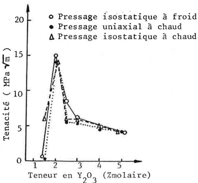
Figure II - 16. Relation entre K_{IC} et la teneur en Y 2 O 3 des zircons yttriés (32)
