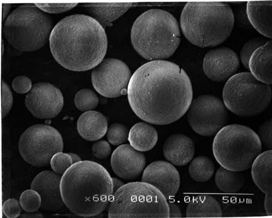
Figure VI - 21 . Micrographie au MEB de la poudre d' \text{Al}_2\text{O}_3 - \text{ZrO}_2 (15 % en poids) traité 30 minutes à 1200^\circ\text{C} , utilisée pour le frittage
