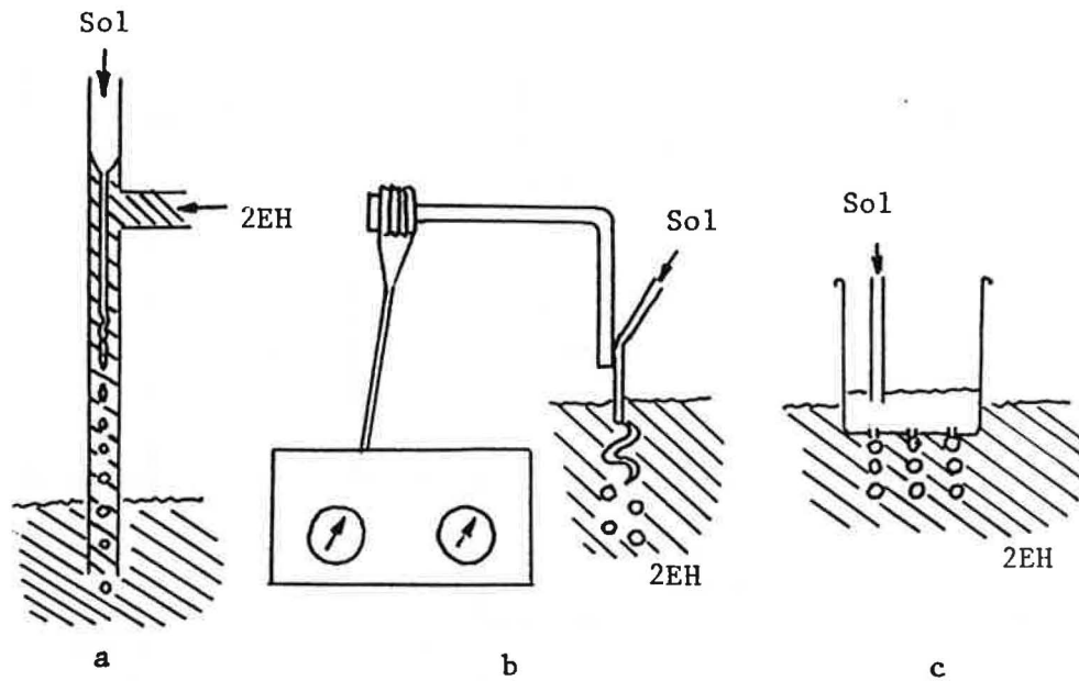
a) tuyère à deux liquides
