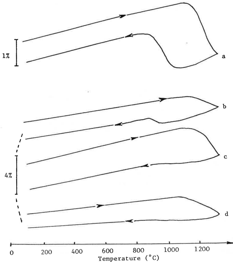
Figure V - 14. Courbes de dilatométrie des poudres traitées à 1200°C, pendant 1 heure: a) ZrO_2 pure b) ZrO_2 + 1.5% molaire Y_2O_3 c) ZrO_2 + 2% molaire Y_2O_3 d) ZrO_2 + 3% molaire Y_2O_3
