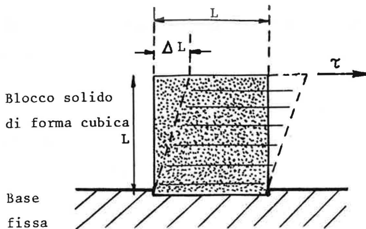
Figura III.1 - Deformazione di un fluido soggetto ad uno sforzo di taglio
