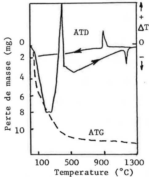
Figure IV - 2 . Analyse thermique (ATD-TG) d'un gel précipité à pH = 10 (2)
