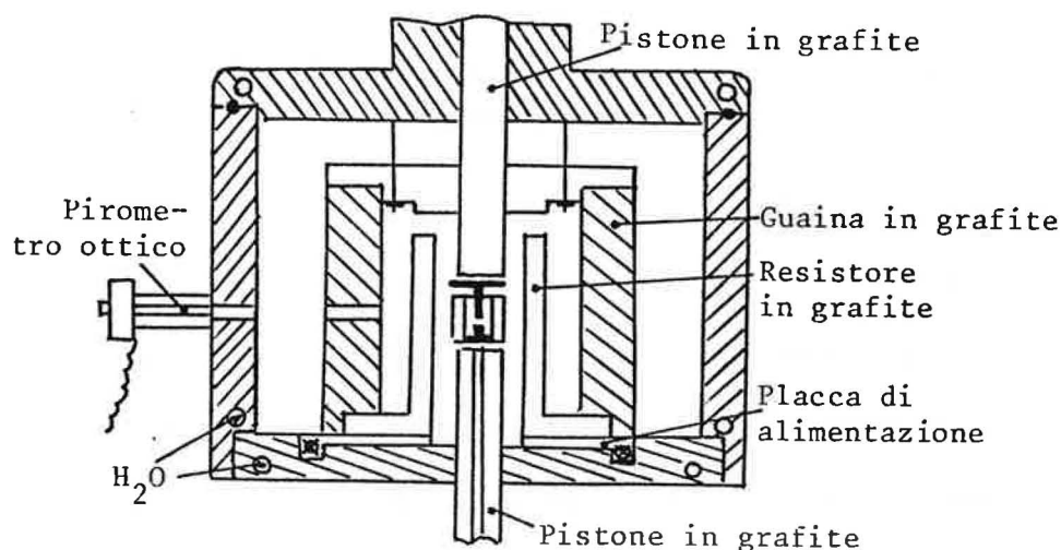
Figura III - 7. Schema del fornello riscaldante per la pressatura a caldo
