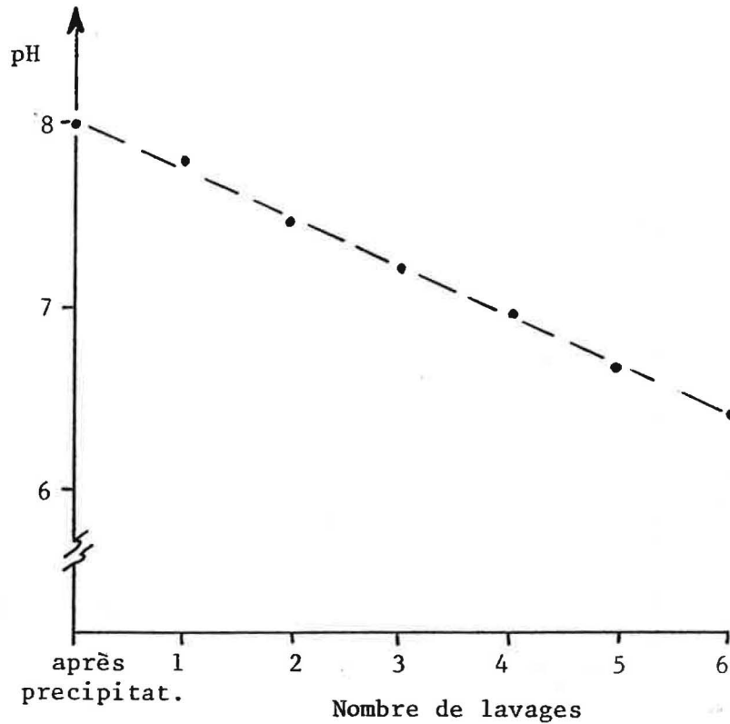
Figure V-1 . Variation du pH de la suspension gélatineuse en fonction du nombre des lavages.
