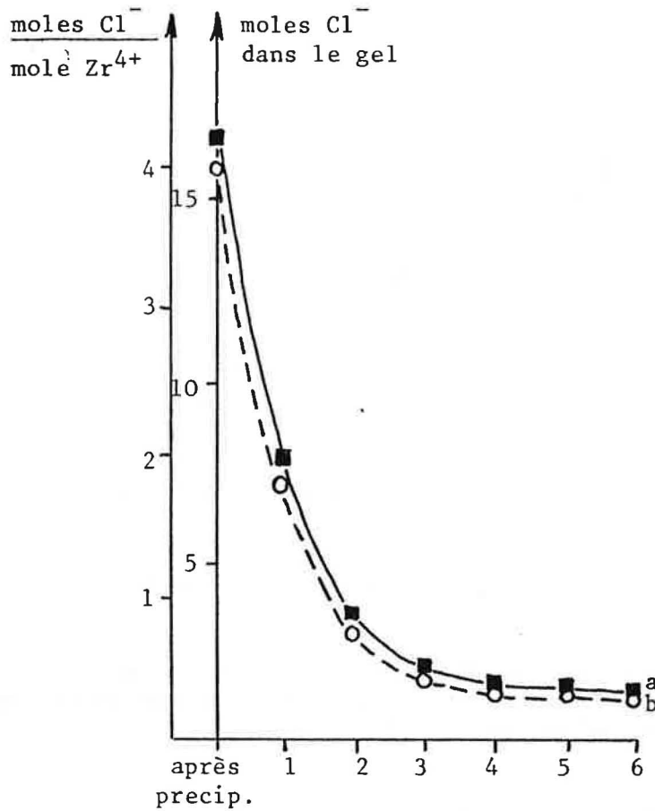
Figure V - 17. Influence du nombre de lavages sur la teneur en ions Cl - du gel (mélange à 2% molaire de Y 2 O 3 ): a) moles Cl - dans le gel b) moles Cl - / mole Zr 4+
