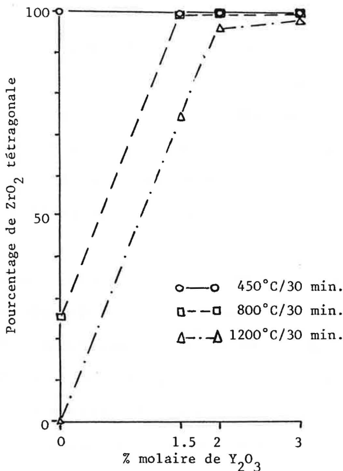
Figure V-18 - Evolution de la pourcentage de zircone tétragonale en fonction de la température
