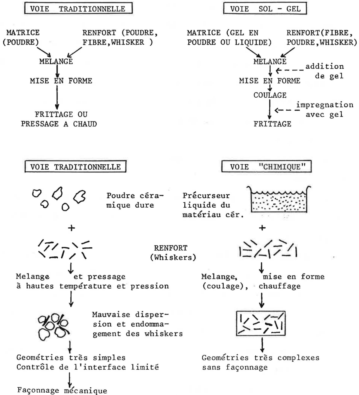
Figure I - 2 . Comparaison entre les procédés de préparation des composites par voie traditionnelle et par voie sol-gel (7)
