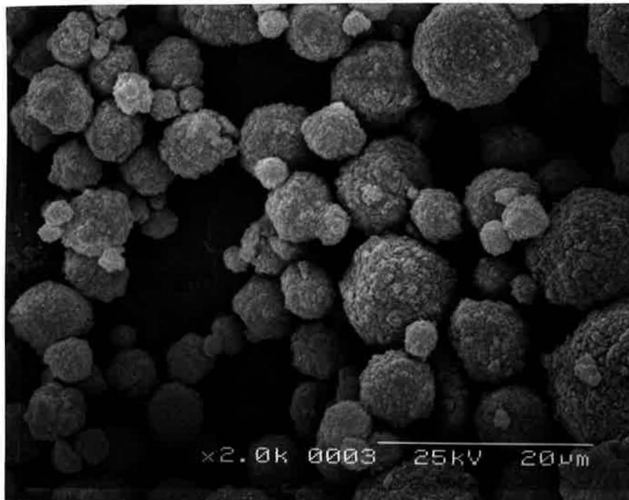
Figure VI-8 . Micrographie MEB de la poudre d' Al_2O_3 + 20 % en poids de zircon obtenue par atomisation.
