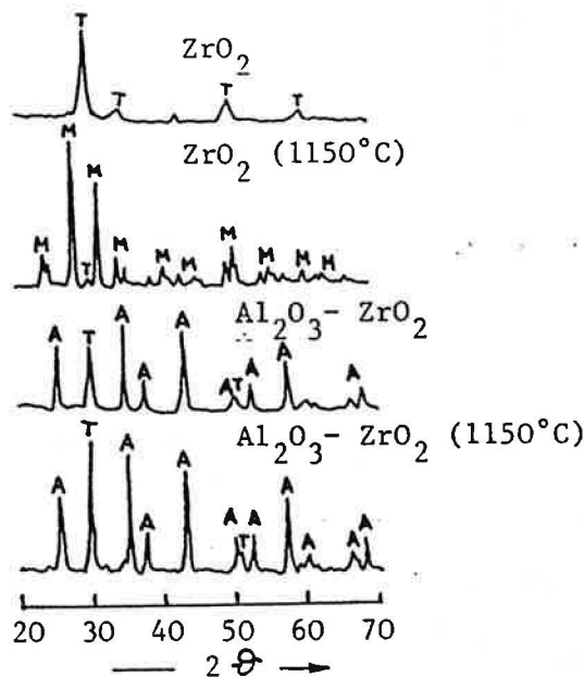
Figure II - 23. Diagrammes de diffraction des Rayons X des poudres obtenues par "EDS", avant et après le traitement thermique à 1150°C pendant 3 h (41)
