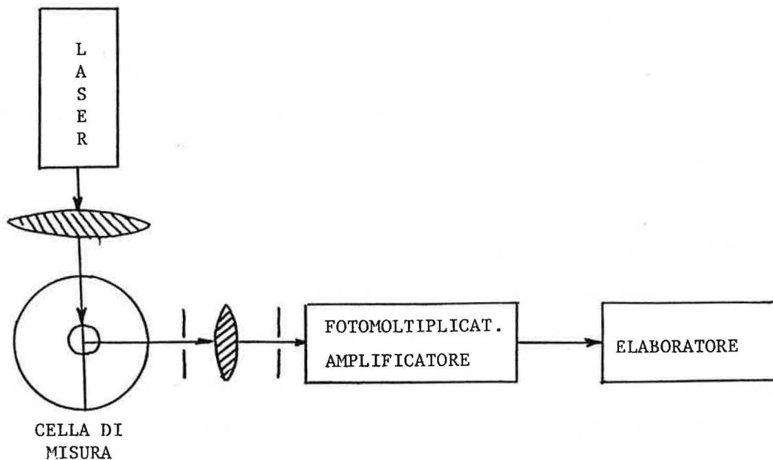
Figura III - 6 . Schema di funzionamento di un microgranulometro laser
