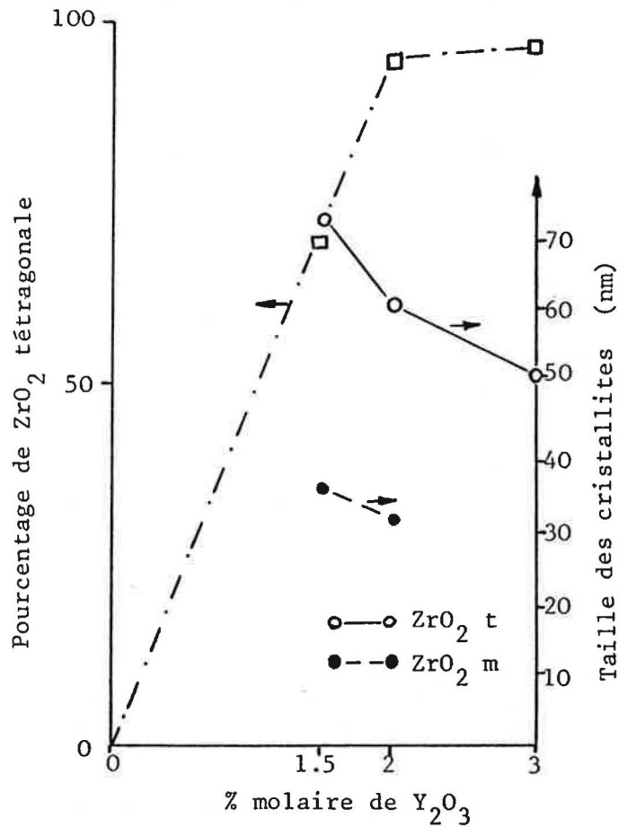
Figure V-20. Influence d'un traitement thermique prolongée sur la taille des cristallites et sur le pourcentage de ZrO_2 tétragonale
