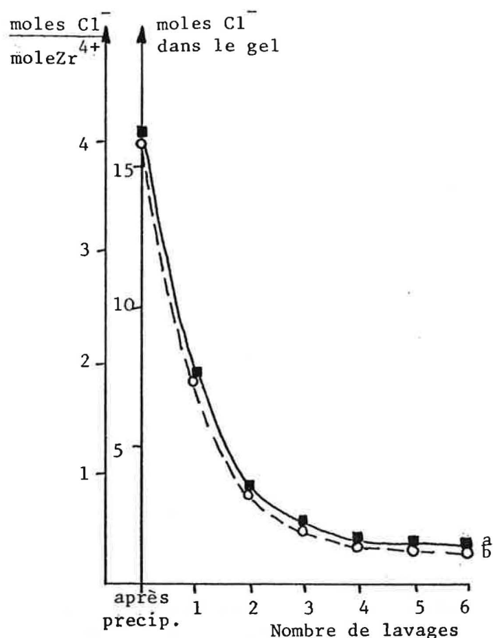
Figure V-3 . Variation de la quantité des ions chlorures dans le gel en fonction du nombre de lavages: a) moles Cl - dans le gel b) moles Cl - /mole Zr 4+
