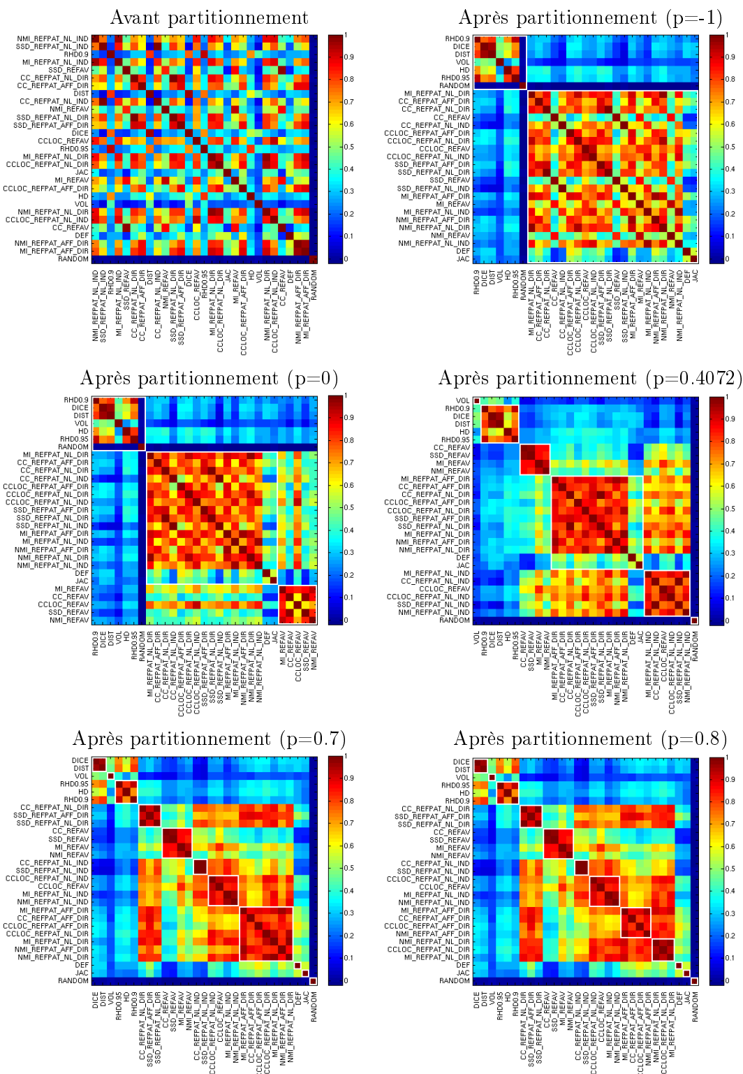
FIG. 6.7 – Coefficient de Spearman moyen pour chaque couple de méthodes de sélection d’atlas (méthodes automatiques ou de référence appliquées ici de façon globale) avant partitionnement (en haut à gauche), et après partitionnement pour différentes valeurs d’auto-similarité : p = -1, 0, 0.4072 (valeur médiane des valeurs de similarité données en entrée), 0.7 et 0.8. Les sous-groupes sont représentés par des carrés blancs.
