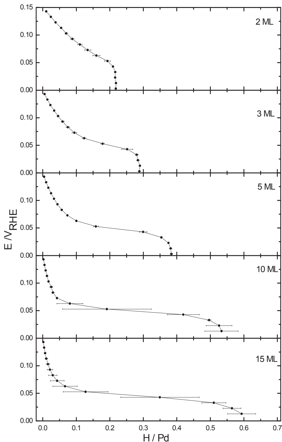
Figure I.6: Isothermes d'insertion électrochimiques pour les films Pd_{xMC}/Au(111) , 0,1 \text{ M } H_2SO_4 .
