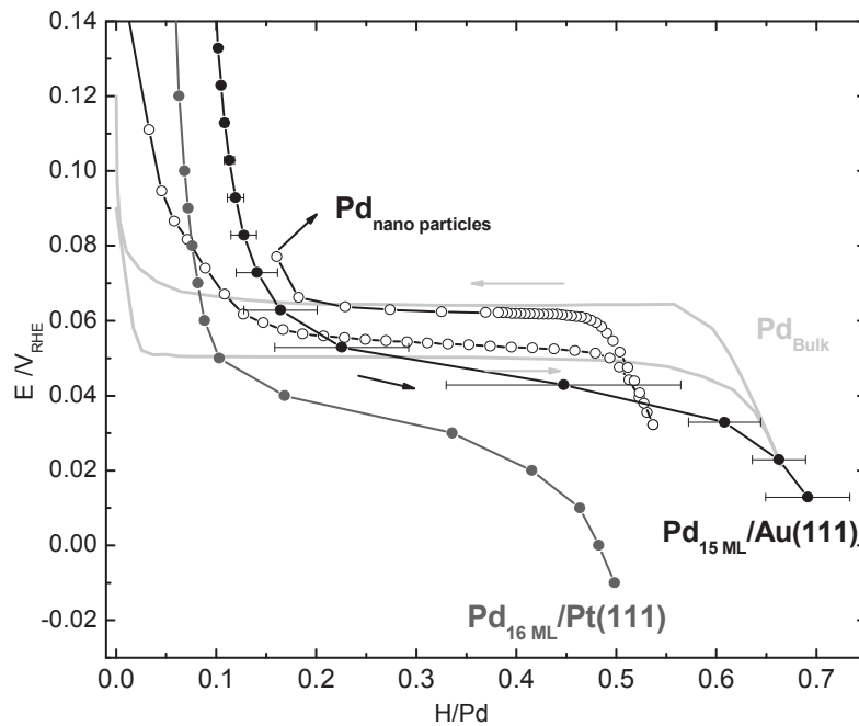
Figure I.9: Isotherme de H dans Pd massif, des nanoparticules de Pd non-supportées (taille moyenne 3,6 nm) [7, 43] et des nanofilms de Pd : Pd 15ML /Au(111) et Pd 16ML /Pt(111) b .
