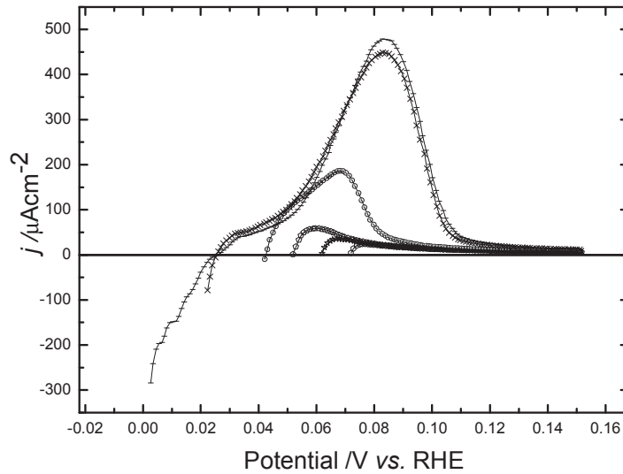
Figure I.3: Calcul de l'isotherme d'absorption : balayages positifs mesurés pour Pd 15 MC/Au(111), 10 mV·s -1 .
