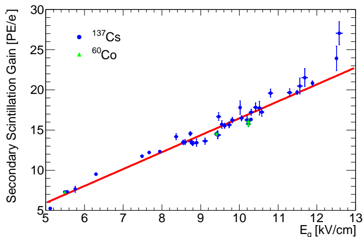
FIG. 2.15: Le gain de scintillation secondaire de XENON100 en fonction du champ électrique dans la zone d'amplification, avec une hauteur de gaz de 2.9 mm choisie comme référence. Extrait de [60].
