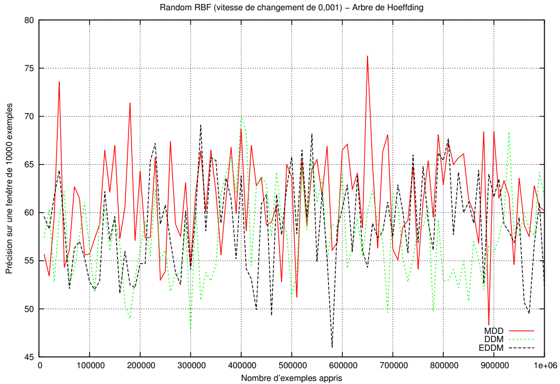
FIGURE 5.16 – Précision sur une fenêtre de taille 10000 sur les différentes méthodes de détection (Arbre de Hoeffding avec le jeu de données Random RBF en mouvement).
