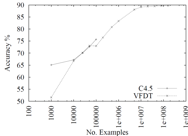
FIGURE 2.2 – Comparaison de C4.5 avec VFDT (extraite de [DH00]).
