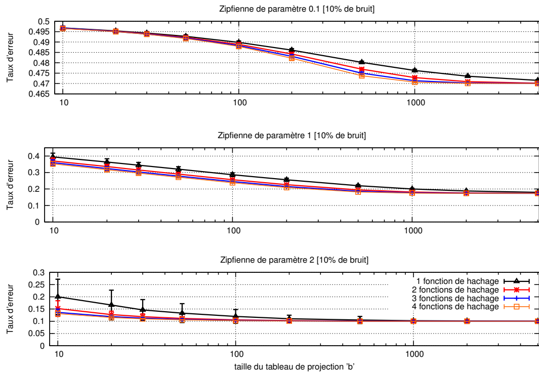
FIGURE 3.16 – Comparaison des moyennes des taux d’erreurs pour le résumé CMSCClass après 1 millions d’insertion avec 'b' allant de 10 à 5000 après ajout de 10% de bruit.
