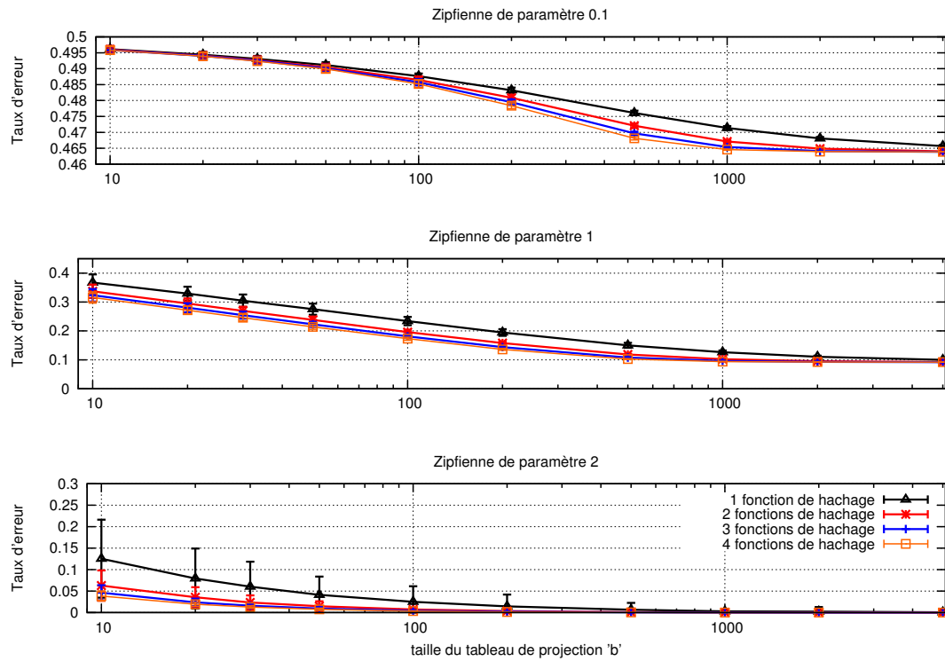
FIGURE 3.15 – Comparaison des moyennes des taux d’erreurs pour le résumé CMSCClass après 1 millions d’insertion avec 'b' allant de 10 à 5000.
