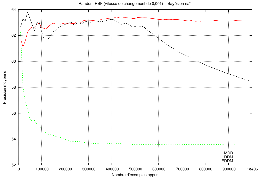
FIGURE 5.12 – Précision moyenne sur les différentes méthodes de détection (classifieur bayésien naïf avec le jeu de données Random RBF en mouvement).
