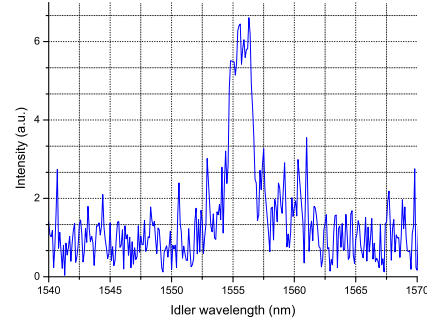
FIGURE 4.3: Spectre de fluorescence paramétrique autour de 1550 nm. La période d'inversion du signe du coefficient est de 7 \mu\text{m} et la longueur d'onde de pompe est de 532 nm. En raison d'une plage de détection limitée, seule la plus haute longueur d'onde (idler) est visible.
