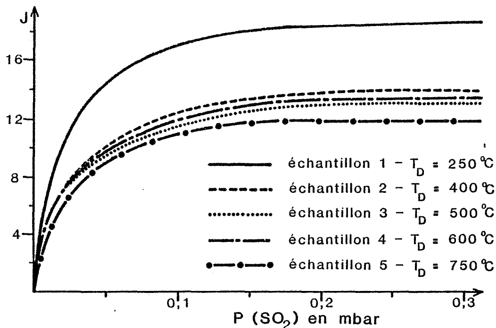
Chaleur dégagée au cours de l'adsorption de \text{SO}_2 à 250^\circ\text{C} en fonction du prétraitement de NiO
