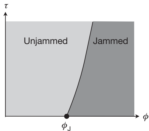
FIGURE 1.2 – Diagramme de phase du jamming proposé par Liu and Nagel (1998) pour un assemblage de grains non frottants et non soumis à une agitation thermique (extrait de Bi et al. (2011)).
