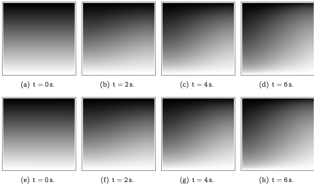
FIGURE 2.5 – Haut : séquence I_s(x,t) obtenue par simulation du modèle complet. Bas : séquence I_s^L(x,t) obtenue par projection de I_s(x,t) sur la base \Psi .
