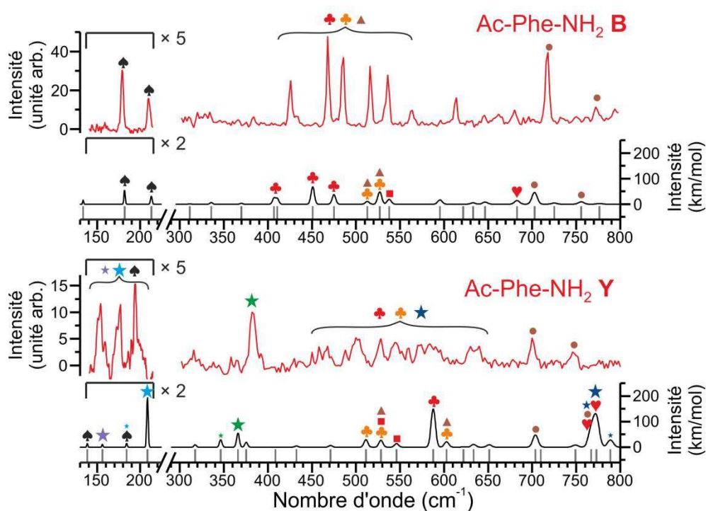
Fig. B.3.2.a – Comparaison des spectres de double résonance IR-UV des conformères B (isolé) et Y (monosolvés) de Ac-Phe-NH 2 (en rouge) et des spectres harmoniques RI-B97-D non corrigés (en noir). Les significations des symboles des modes de vibration sont indiquées dans la Figure B.3.3.a de l'annexe B.
