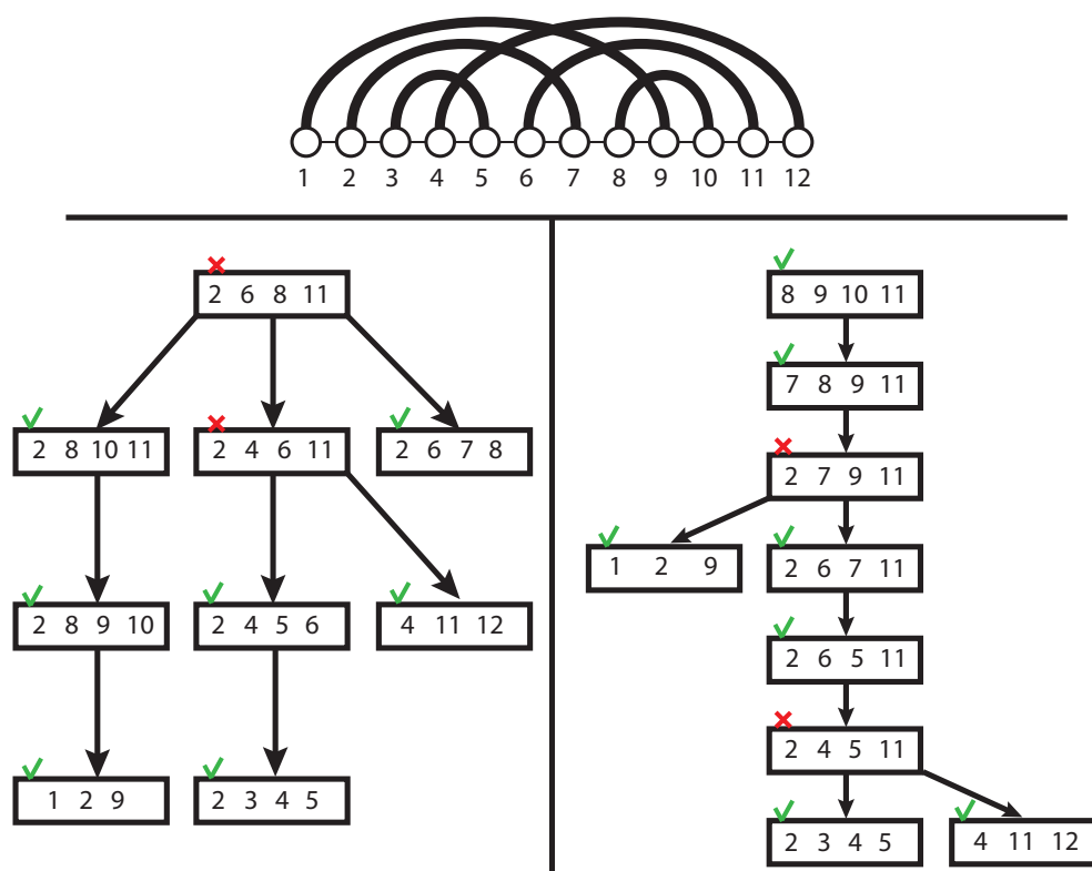
FIGURE 4.25 – Décompositions arborescentes issues des heuristiques degré minimum (à gauche) et remplissage minium (à droite) d'un pseudo-nœud standard de degré 3. Les sacs non lissés sont marqués d'une croix (rouge)
