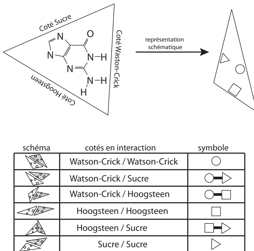
FIGURE 2.5 – Illustration de la nomenclature Léontis-Westhof (interaction en cis uniquement)[35].
