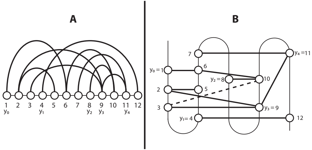
FIGURE 4.14 – A : Une séquence arc-annotée avec un plongement en vagues associé, symbolisé par les pivots (en dessous de la séquence). B : Représentation en vagues de la séquence arc-annotée associée au plongement en vagues de la figure A . Le plongement contient un croisement, par exemple au niveau de l'interaction en pointillés.
