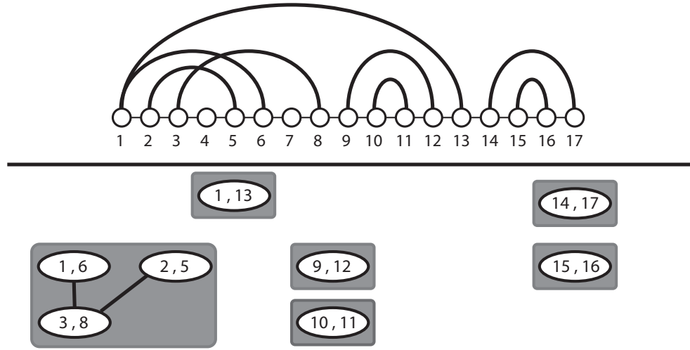
FIGURE 4.9 – Une séquence arc-annotée et son graphe des conflits. Les sommets du graphe des conflits (formes elliptiques) sont regroupés en composantes connexes (cadres grisés).
