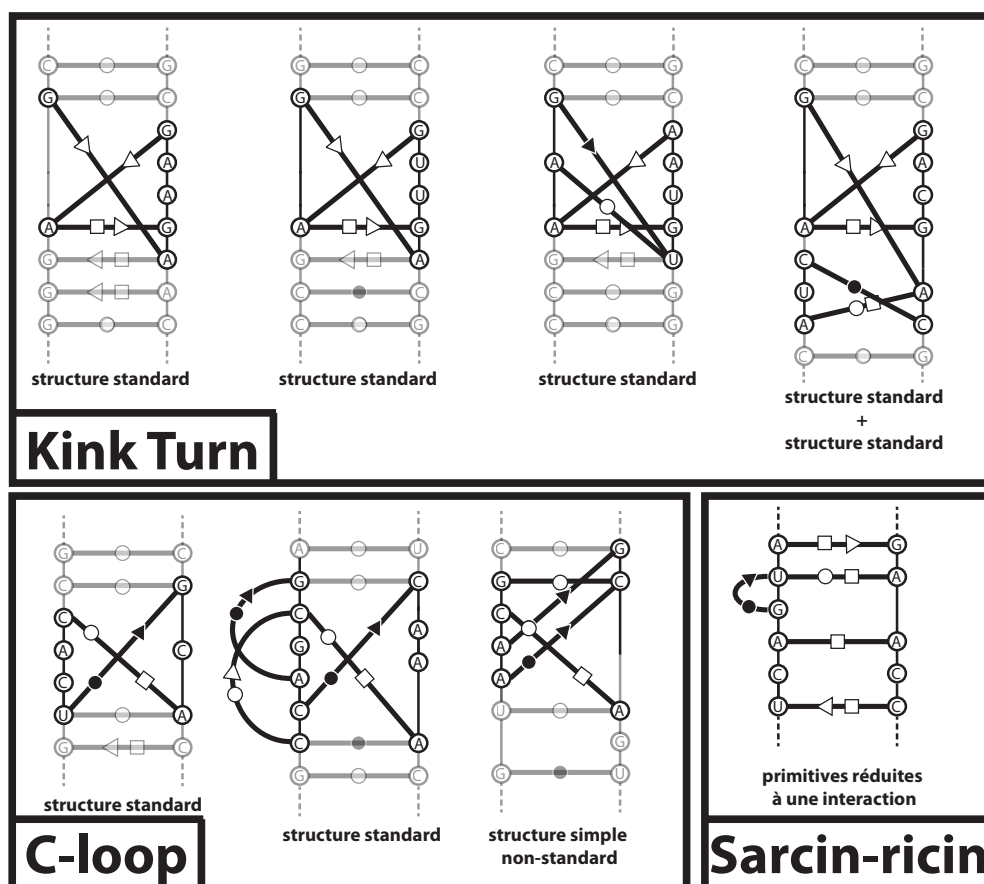
FIGURE 4.26 – Exemple de motifs (Kink Turn, C-loop et sarcin-ricin). Les différentes occurrences représentées (structures grisées+non-grisées) sont toutes combinaisons de structures secondaires et de structures primitives non secondaires (structures non-grisées). Ces structures primitives appartiennent néanmoins à l'une des classes que nous avons définies.
