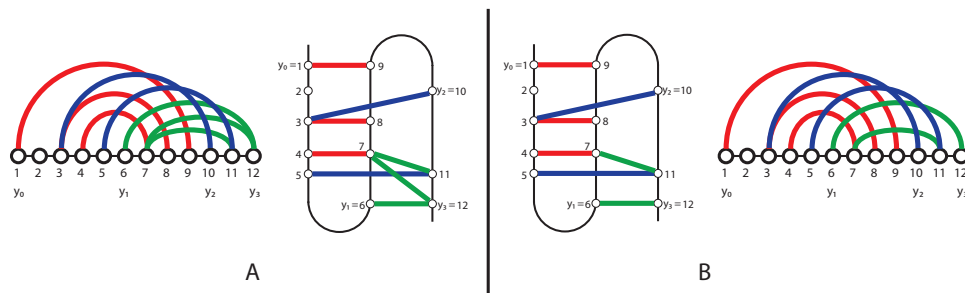
FIGURE 3.13 – À gauche : une triple hélice standard, à droite : une structure qui n'est pas une triple hélice standard.
