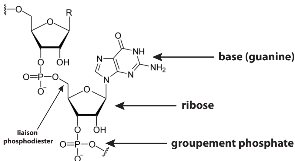
FIGURE 2.2 – Représentation classique d'un nucléotide relié par un liaison phosphodiester à un autre nucléotide.
