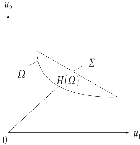
FIG. 4. L'enveloppe convexe H(\Omega) de \Omega dans le cas où r est décroissance et convexe.
