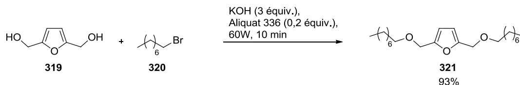
Schéma 91 : synthèse d'éther selon Williamson activée par micro-ondes
