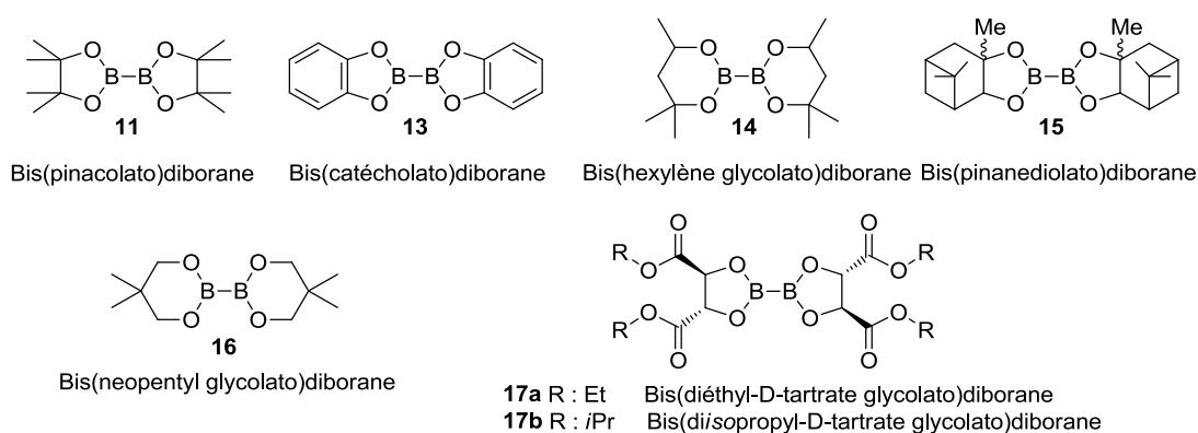
Figure 1 : exemples d'esters de diboranes commerciaux
