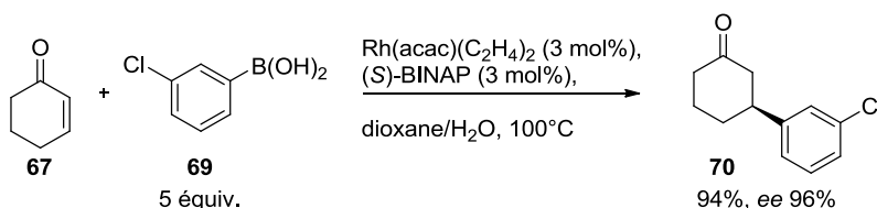
Schéma 30 : addition de type Michael énantiosélective
