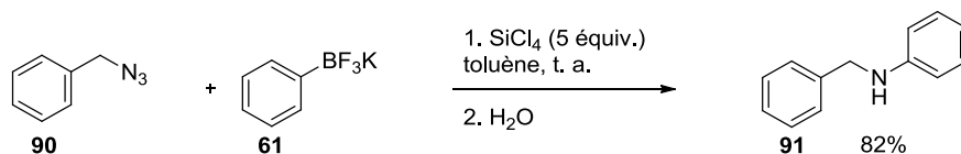
Sch\u00e9ma 38 : utilisation d'azoture pour la formation d'amines secondaires
