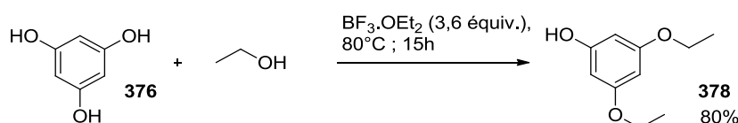
Schéma 121 : disubstitution du phloroglucinol par l'éthanol
