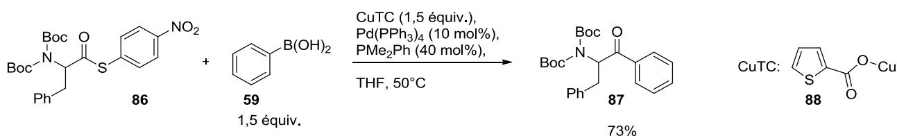
Sch\u00e9ma 36 : acylation de boronique par des thioesters
