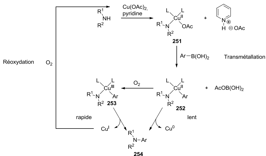
Schéma 72 : mécanisme de la réaction de Chan-Lam
