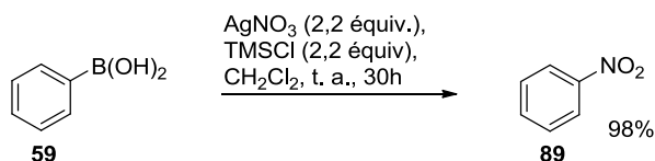
Sch\u00e9ma 37 : nitration \u00e9lectrophile d'acide boronique
