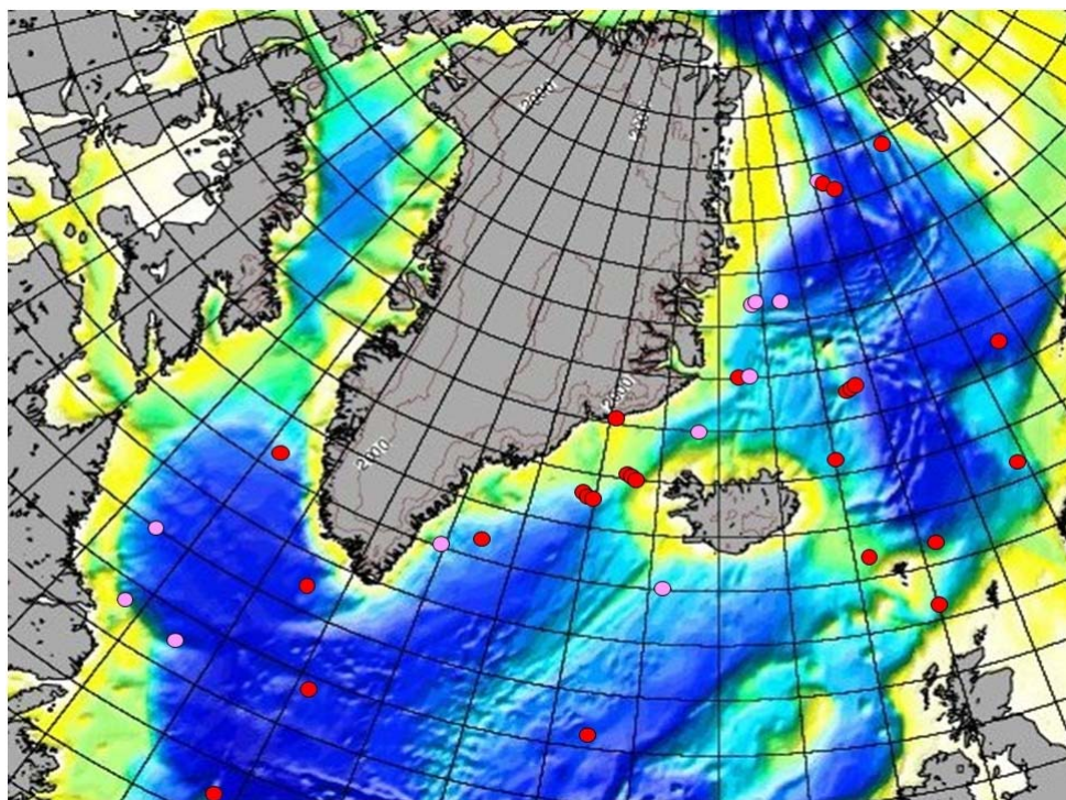
Figure 10: Carte d'échantillonnage du projet Signature.
