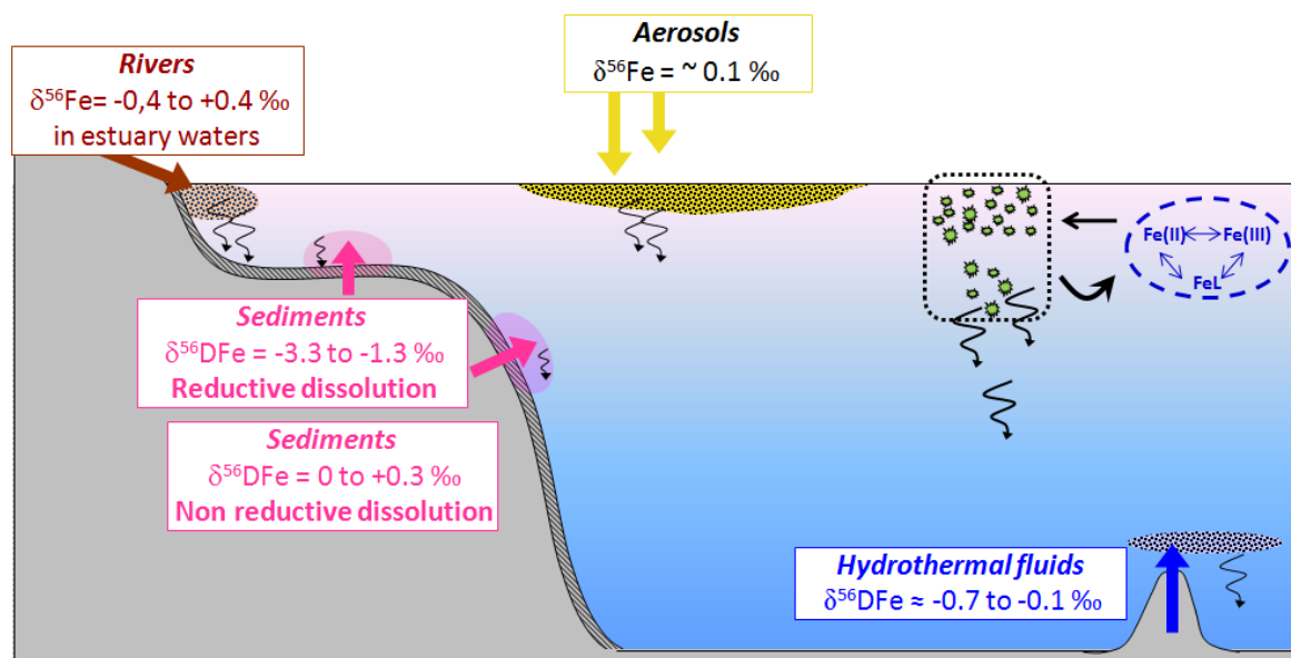
Figure 24: CI de Fe des sources de Fe à l'océan.
