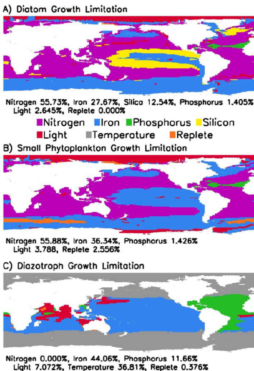
Figure 4: Facteur limitant le plus les taux de croissance pour chaque groupe de phytoplancton pour les mois d'été de chaque hémisphère [Moore et al., 2004].
