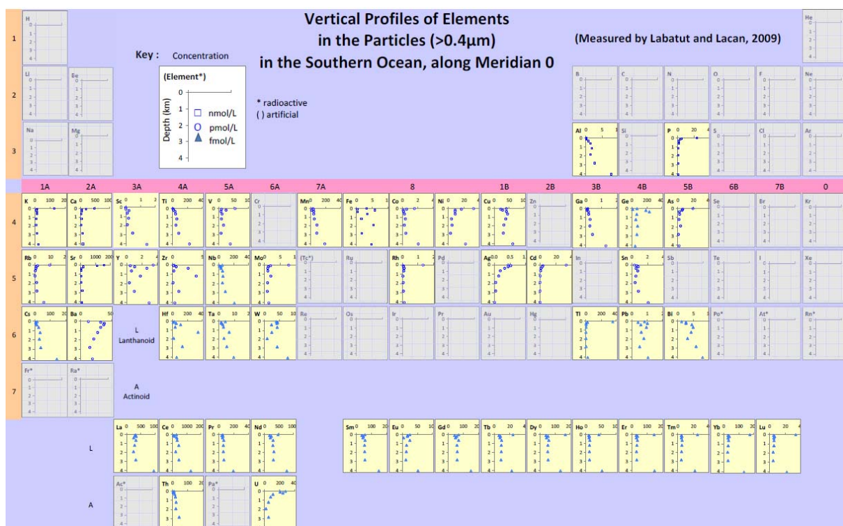
Figure 35: Tableau périodique des éléments dans les particules en suspensions dans l'océan Austral. ATTENTION, il s'agit de données préliminaires, qui ne sont pas toutes validées.
