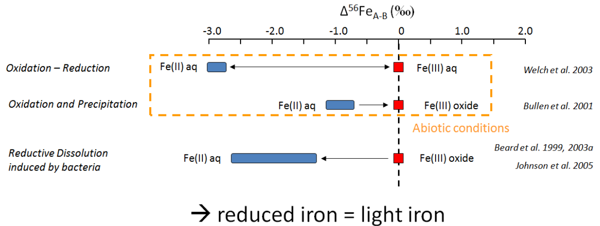
Figure 23: Fractionnement isotopique du Fe lors de processus d'oxydoréduction.
