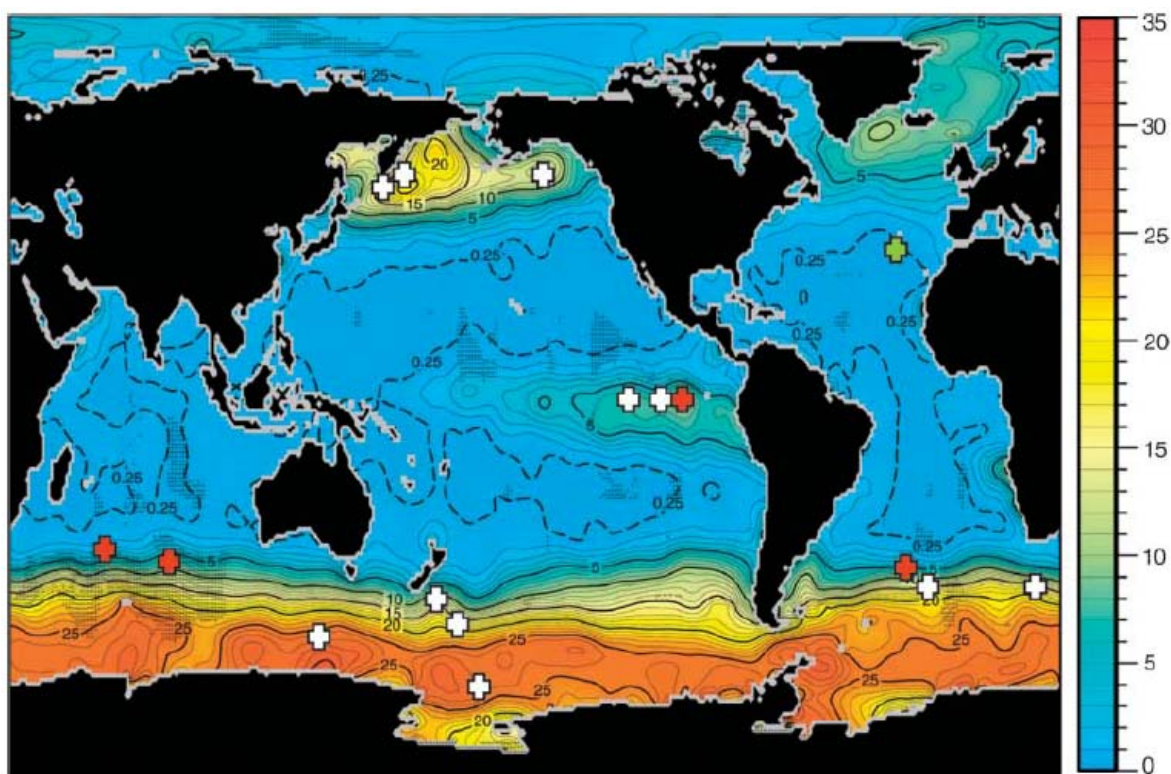
Figure 3: Concentrations de nitrates ( \mu\text{mol/L} ) dans la couche mélangée de surface, en moyenne annuelle, mettant en évidence les régions HNLC.
