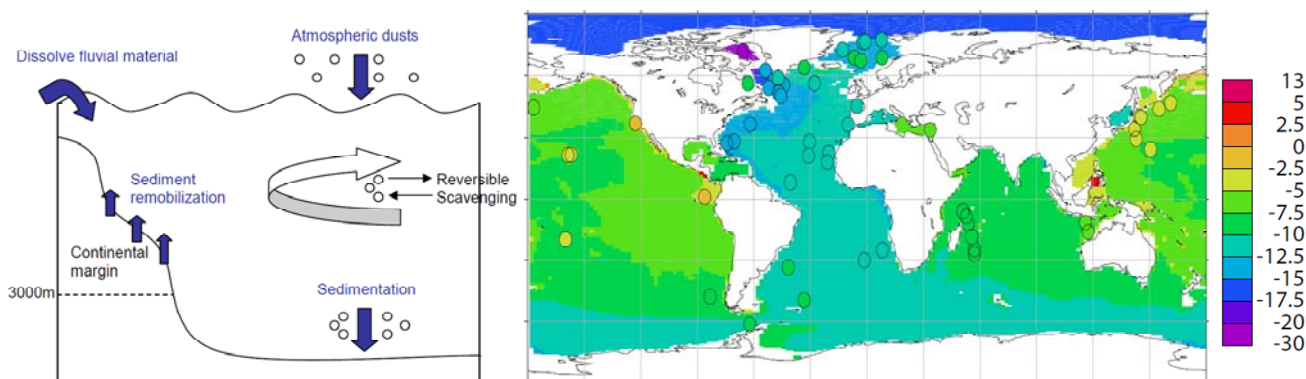
Figure 16: Modélisation couplée physique/biogéochimie du cycle d' \varepsilon_{Nd} [Arsouze et al., 2009].
