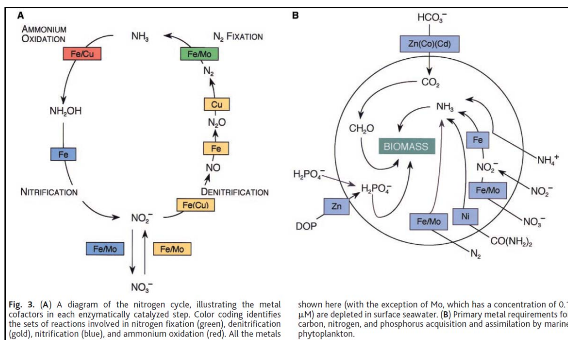
Figure 2: Rôles joués par ces micro-nutritifs lors de l'acquisition et l'assimilation du carbone de l'azote et du phosphore [Morel et Price, 2003].
