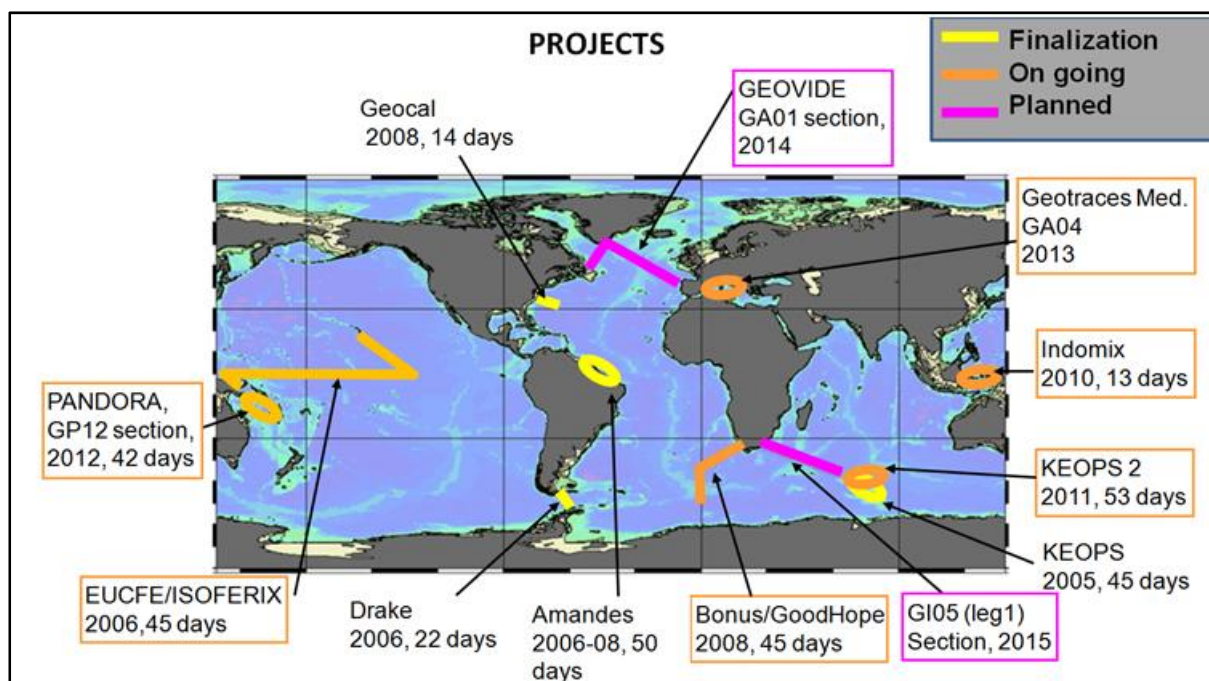
Figure 1: Campagnes en mer de l'équipe GEOMAR, depuis 2005.
