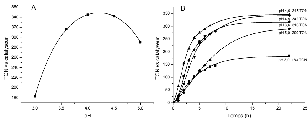
Figure 3 : Activités photocatalytiques en terme de TON Cat en fonction du pH (A) et en fonction du temps à différents pH (B), pour une solution aqueuse contenant PS1 ( 5 \times 10^{-4} M), [Co(CR)Cl 2 ] + ( 0,8 \times 10^{-4} M) et NaHA/H 2 A (1,1 M) après 22 h d'irradiation dans le visible (400-700 nm).
