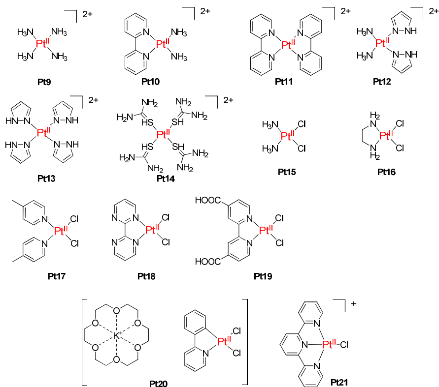
Schéma 8 : Structures des catalyseurs à base de complexes mononucléaires de Pt développés par Sakai et coll.
