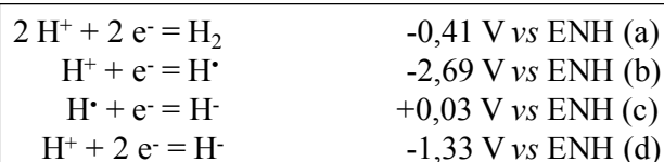
Schéma 2 : Potentiels de réduction à un et deux électrons des protons dans l'eau à \text{pH } 7,0 , 298\text{ K} , pression standard de \text{H}_2 d'une atmosphère, concentration des autres espèces à 1\text{ M} .
