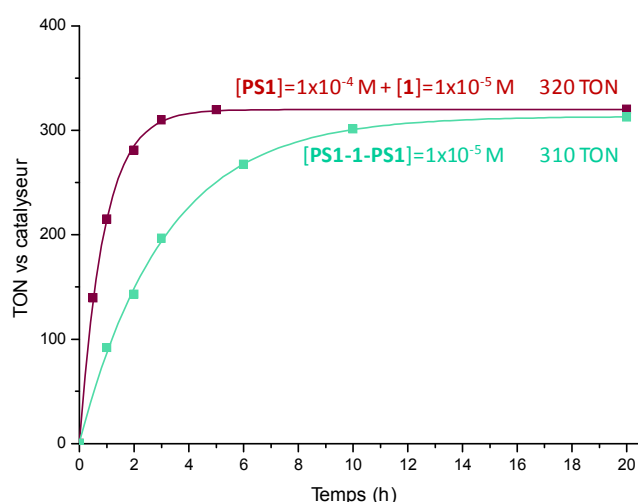
Figure 6 : Production photocatalytique d'hydrogène en fonction du temps en terme de \text{TON}_{\text{Cat}} de solutions aqueuses contenant \text{H}_2\text{A} (0,55 M) et \text{NaHA} (0,55 M) à pH 4,0 sous irradiation visible 400 - 700 nm en présence de : PS1-1-PS1 ( 1 \times 10^{-5} M) et comparaison avec un mélange de complexes [\text{Ru}(\text{bpy})_3]^{2+} ( PS1 ) ( 1 \times 10^{-4} M) et [\text{Rh}(\text{dmbpy})_2\text{Cl}_2]^+ ( 1 ) ( 1 \times 10^{-5} M) (ratio 10/1) (traits pointillés).
