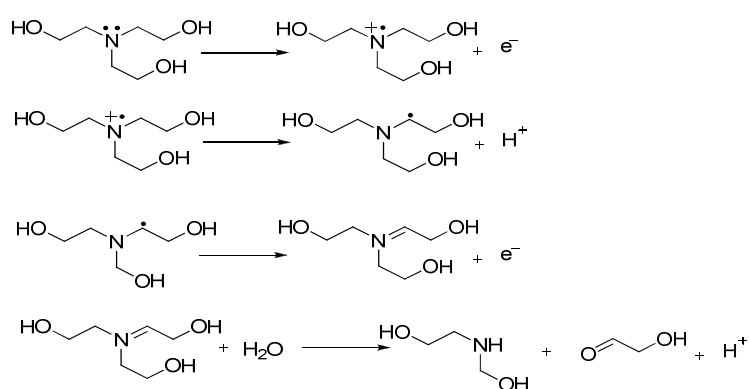
Schéma 3 : Mécanisme d'oxydation irréversible de TEOA
