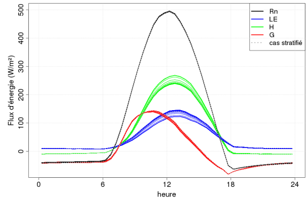
FIGURE 10.14 – Moyenne annuelle du cycle journalier des 4 termes du bilan d'énergie pour chaque pixel : rayonnement net ( Rn ), flux de chaleur latente ( LE ), de chaleur sensible ( H ) et de chaleur dans le sol ( G )
