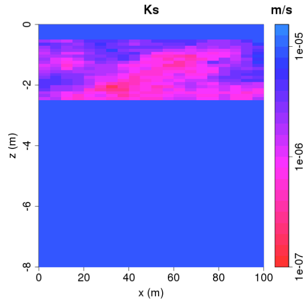
FIGURE 9.2 – Coupe verticale de la conductivité hydraulique à saturation ( K_S )
