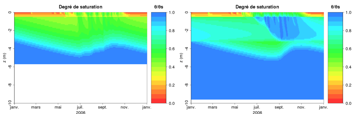
FIGURE 10.9 – Evolution temporelle du degré de saturation pour la configuration en dents de scie pour x = 137,5 m FIGURE 10.10 – Evolution temporelle du degré de saturation pour la configuration en dents de scie pour x = 197,5 m
