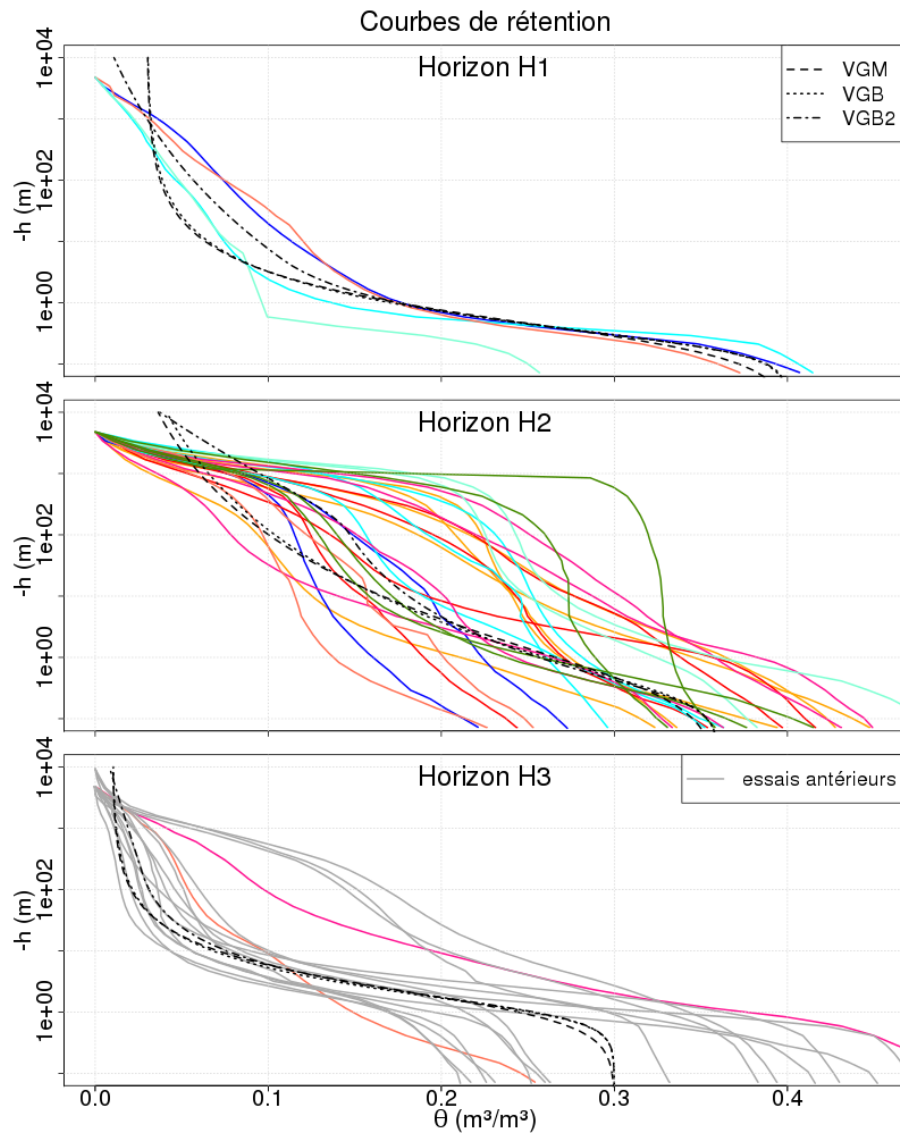
FIGURE 6.7 – Courbes de rétention obtenues par porosimétrie au mercure (cf. figure 6.6) (y compris les essais antérieurs réalisés sur des échantillons entre 2 et 7 m de profondeur, cf. figure 2.4), et courbes des équations de van Genuchten-Mualem (VGM), van Genuchten-Burdine (VGB) et van Genuchten-Burdine modifié dans le sec (VGB2)
