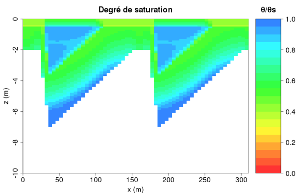
FIGURE 10.17 – Profil de degré de saturation pour une configuration en dents de scie avec un socle moins profond, le 15 octobre (nappe au plus haut)
