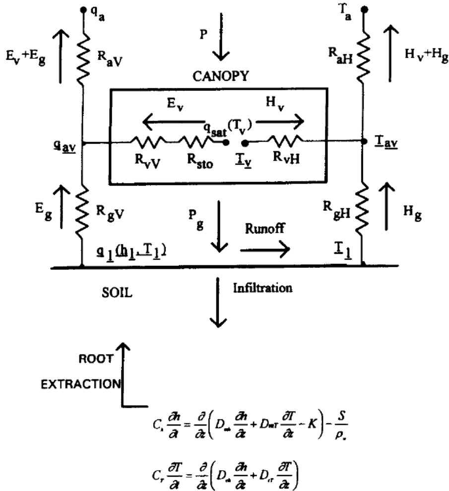
FIGURE 4.1 – Schéma du modèle SiSPAT. D'après Braud et al. (1997).
