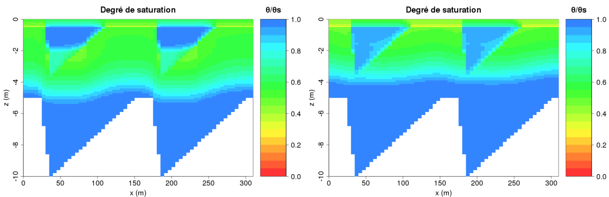
FIGURE 10.6 – Profil de degré de saturation pour la configuration en dents de scie le 2 août (nappe au plus bas) FIGURE 10.7 – Profil de degré de saturation pour la configuration en dents de scie le 15 octobre (nappe au plus haut)
