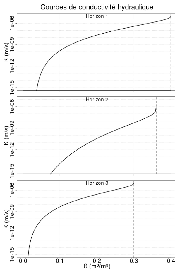
FIGURE 7.2 – Courbes de conductivité hydraulique (équation de van Genuchten-Mualem) pour les 3 horizons
