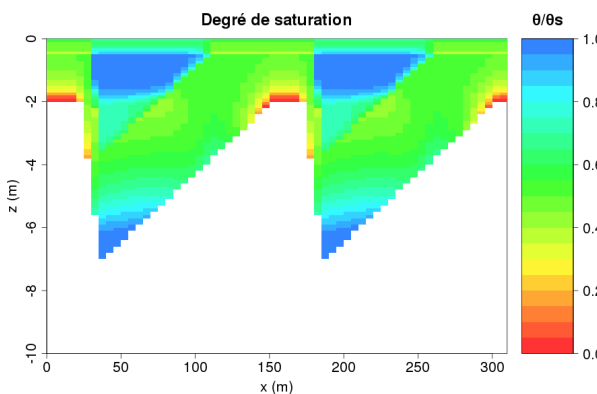
FIGURE 10.16 – Profil de degré de saturation pour une configuration en dents de scie avec un socle moins profond, le 2 août (nappe au plus bas)
