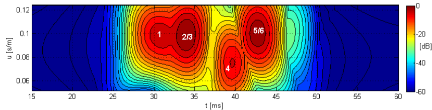
FIGURE 8: Vespagramme synthétique (1) Onde directe (2/3) Réflexions sur les bords droit et gauche (4) Réflexion sur le fond (5/6) Réflexions doubles sur les bords.
