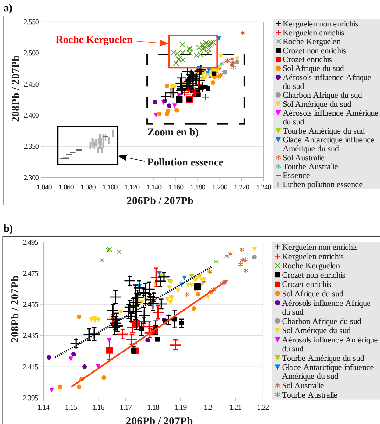
Figure III-2 : Rapports isotopiques ^{208}\text{Pb}/^{207}\text{Pb} en fonction des rapports ^{206}\text{Pb}/^{207}\text{Pb} mesurés aux îles Kerguelen (croix) et de Crozet (carré) : comparaison avec la littérature. Les échantillons enrichis en plomb (pendant l'hiver austral) sont représentés en rouge, les non enrichis en noir. Références : roche Kerguelen [Gautier et al., 1990 ; Weis et al., 1993] ; sol Afrique du sud [Soderberg et Compton, 2007 ; Vallelonga et al., 2010] ; sol Australie [Bollhöfer et al., 2005 ; Lottermoser, 2009 ; Vallelonga et al., 2010] ; sol Amérique du sud [Dejonghe et al., 2002 ; Vallelonga et al. 2010] ; aérosols [Witt et al., 2006] ; tourbes [Kylander et al., 2010] ; charbon Afrique, lichen, essence [Monna et al., 2006] ; glace Antarctique [Vallelonga et al., 2010].
