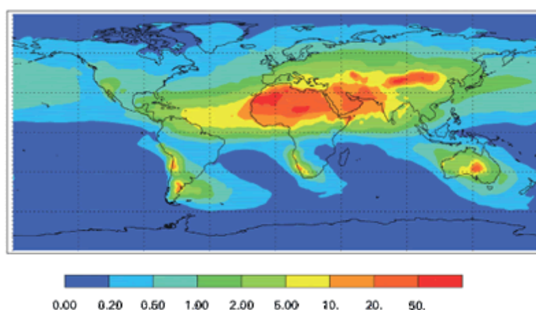
Figure 7: Estimation du dépôt moyen de poussières atmosphériques en g \cdot m^{-2} \cdot an^{-1} [Jickells et al. , 2005].
