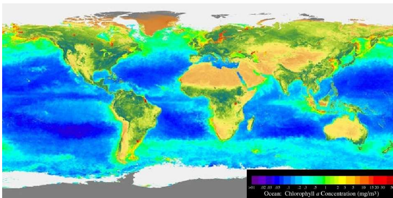
Figure 6: Concentration en pigment dans le phytoplancton (chlorophylle a , en \text{mg}\cdot\text{m}^{-3} ), représentative de la quantité de phytoplancton se trouvant dans les eaux de surfaces océaniques (image satellitaire SeaWiFS, NASA, 2001). La croissance du phytoplancton est limitée dans l'océan austral, en comparaison avec les régions océaniques de l'hémisphère nord situées en hautes latitudes.
