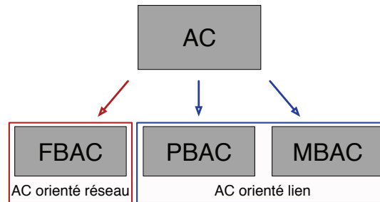
FIGURE 2.2 – Une classification du contrôle d'admission [Statovci-Halimi, 2008].
