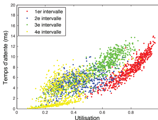
FIGURE 3.3 – Evolution du délai d'attente moyen des paquets dans le buffer du lien en fonction du taux d'utilisation pour un segment de la trace réseau divisé en quatre intervalles de temps de taille identique.
