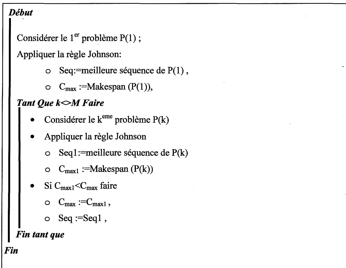
Figure 3. 7. Algorithme de Campbell, Dudek et Smith
