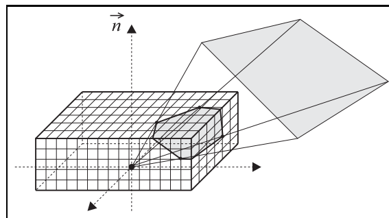
FIG. 3.3 – Méthode de l'hémicube
