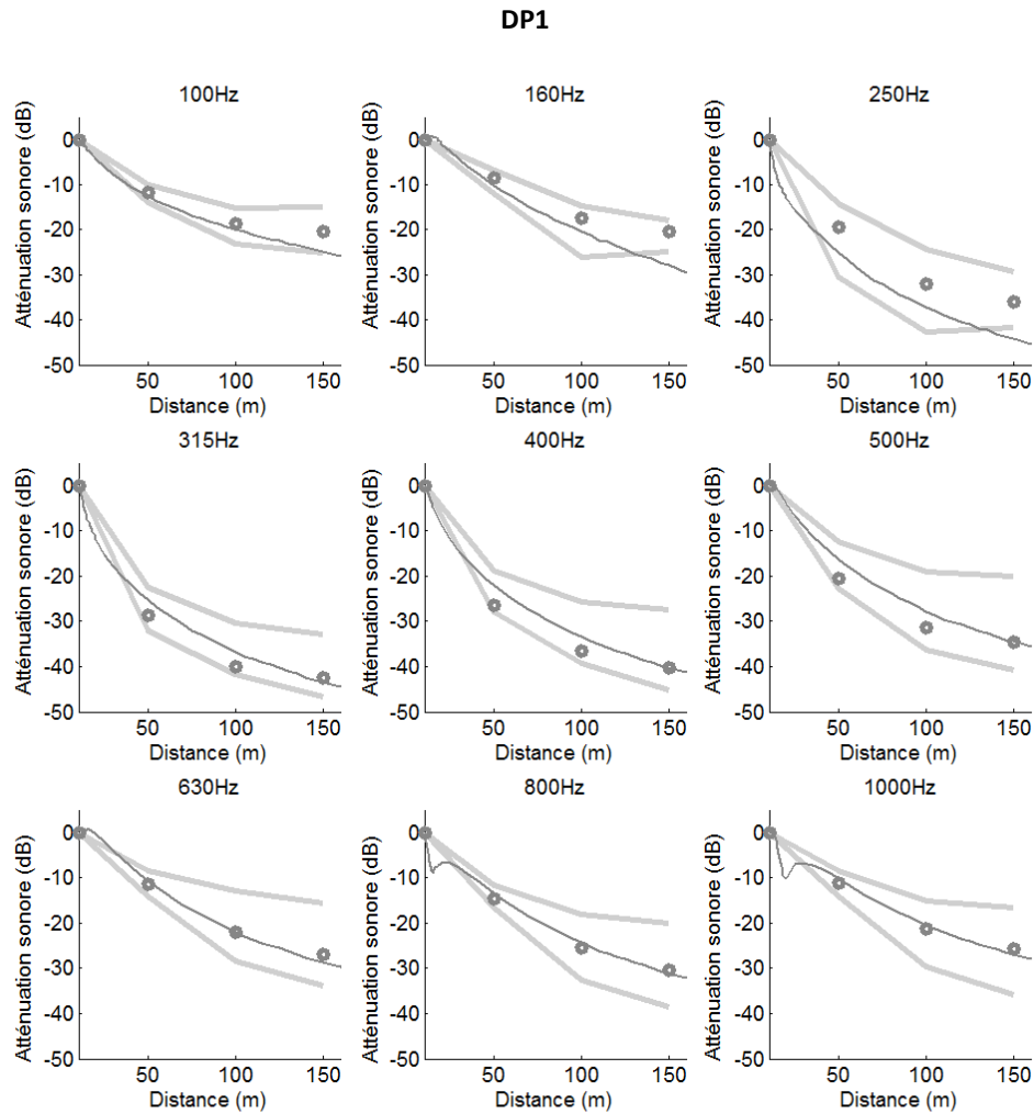
Figure 7.3 : niveaux sonores mesurés (cercles, gris foncé) et simulés (TLM : trait plein, gris foncé) en conditions homogènes selon la direction de propagation 1 avec une résistance de 150 cgs. La dispersion expérimentale des niveaux sonores sur toute la campagne est encadrée par les traits gris clairs.
