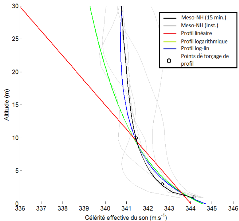
Figure 7.20 : profils moyens (sur les mâts à 50m et 150m de la source) de célérité effective selon DP1, pour le cas INST.
