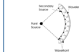
Le principe d'Huygens (1678):
