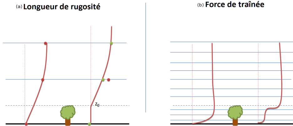
Figure 4.7 : schéma représentant le profil de vent typique en présence de végétation modélisé par la longueur de rugosité z_0 (a), puis par le modèle en force de traînée (b).
