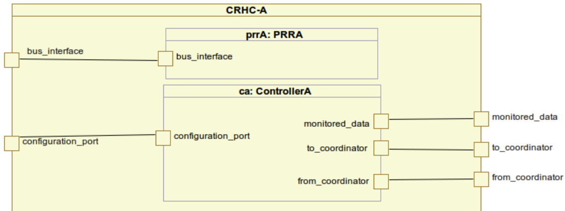
FIG. 5.18 – Modélisation d'un composant matériel reconfigurable contrôlé (CRHC)
