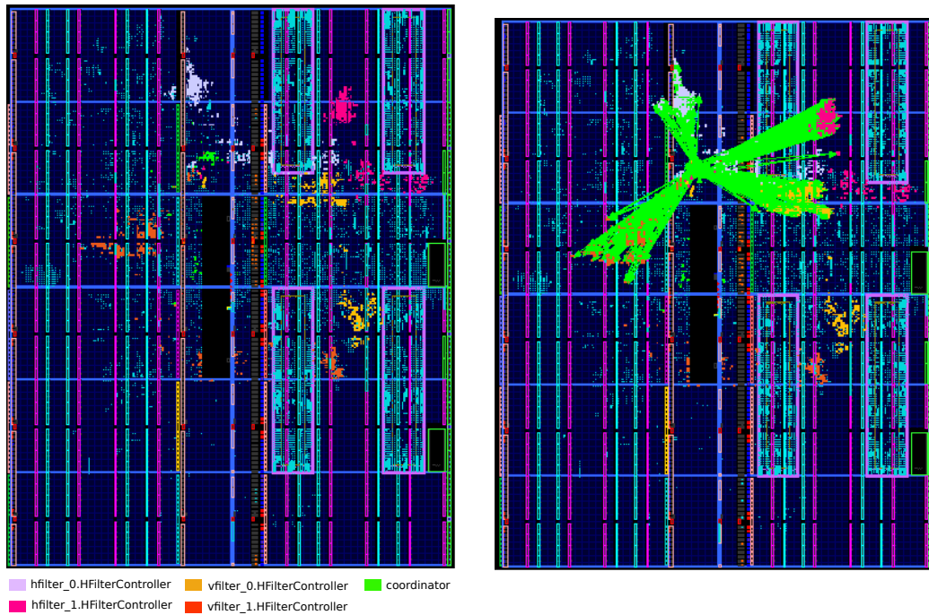
(a) Emplacement du système de contrôle dans le FPGA (b) La communication entre contrôleurs et coordinateur
