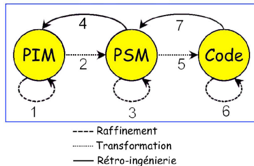
FIG. 3.3 – Les types de transformations de modèles
