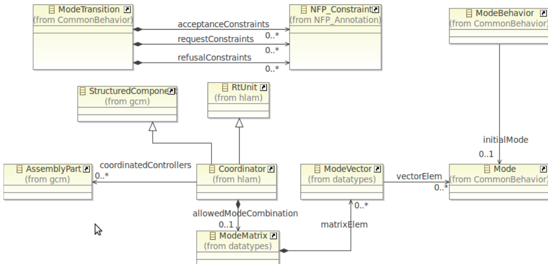
FIG. B.1 – Extension du métamodèle MARTE pour supporter le contrôle semi-distribué
