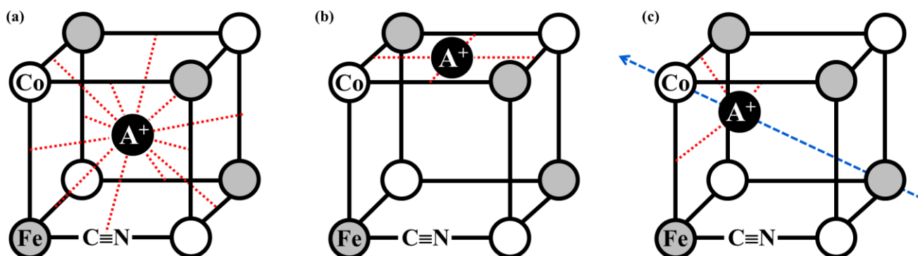
Figure 43 – Différentes positions pour le cation alcalin au sein des ABP A_xCoFe . (a) Cation au centre de l'octant \{Co_4Fe_4\} ; (b) cation au centre des faces \{Co_2Fe_2\} ; (c) cation positionné sur l'axe C_3 (en bleu). Les interactions A^+---CN^- sont représentées par des pointillés rouges. La présence de lacunes en entités \{Fe(CN)_6\} n'est pas représentée dans un souci de clarté.
