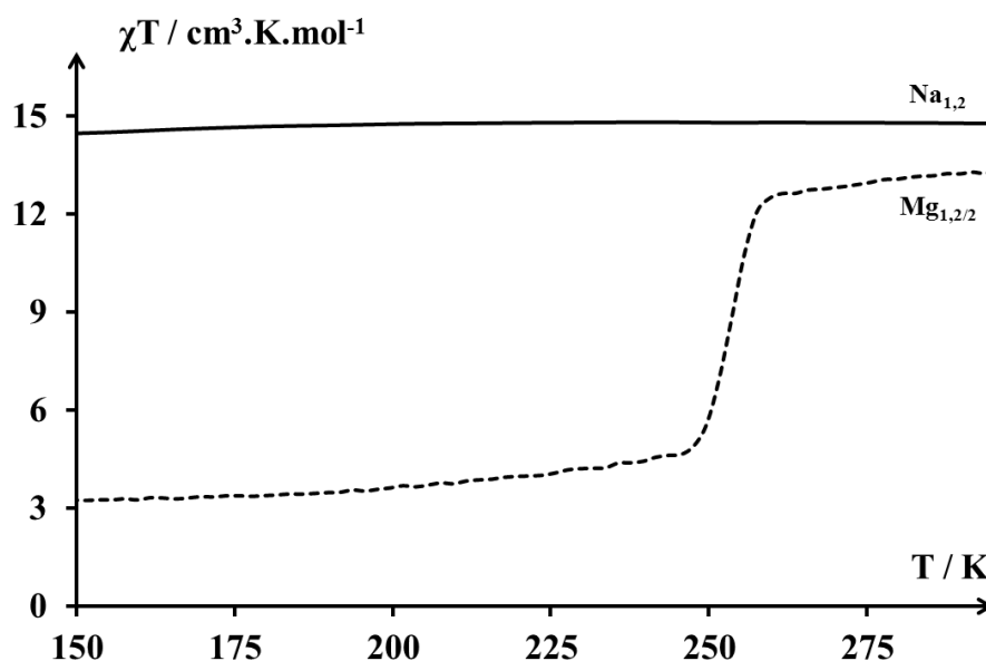
Figure 35 – Évolution du produit de la susceptibilité magnétique et de la température en fonction de la température (lors de la descente en température 300 K \rightarrow 150 K) de l'ABP Mg_{1,2/2}CoFe (trait plein). L'évolution des propriétés magnétique de l'ABP Na_{1,2}CoFe , présentant une transition électronique complète sur la même gamme de température, est donnée à titre de comparaison (trait pointillé).
