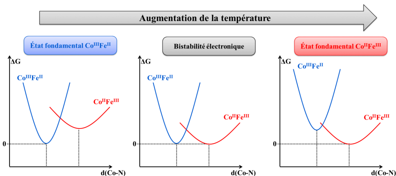
Figure 17 – Stabilisation relative de l'état \text{Co}^{\text{II}}\text{Fe}^{\text{III}} dans les ABP A_x\text{CoFe} lors d'une hausse de la température. Pour chaque température, l'état électronique fondamental est pris comme référence énergétique.
