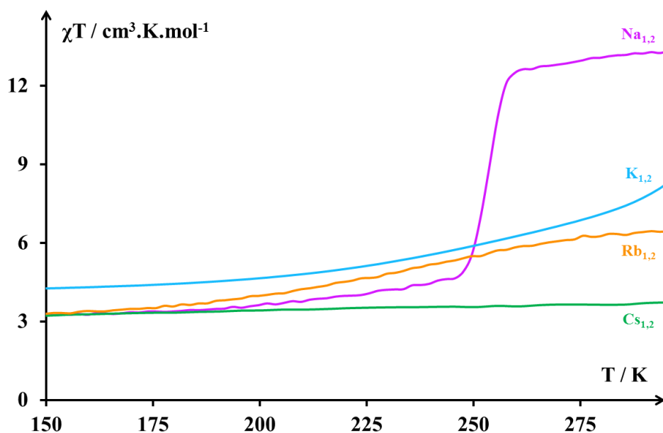
Figure 34 – Évolution du produit de la susceptibilité magnétique et de la température en fonction de la température (lors de la descente en température 300 K \rightarrow 150 K) dans les ABP \text{A}_{1,2}\text{CoFe} . Couleurs : \text{Na}_{1,2}\text{CoFe} (magenta), \text{K}_{1,2}\text{CoFe} (cyan), \text{Rb}_{1,2}\text{CoFe} (vert), \text{Cs}_{1,2}\text{CoFe} (orange).
