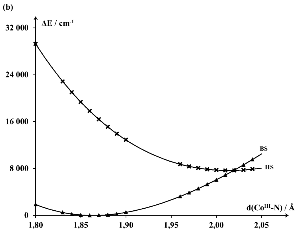
Figure 27 – Évolution de l'énergie relative des états HS (✕) et BS (▲) de plus basse énergie en fonction de la distance d(\text{Co}-\text{N}) dans les monomères [\text{Co}(\text{NCH})_6]^{k+} . Les énergies relatives sont données par rapport à la structure la plus stable. (a) k = 2 ; (b) k = 3 .
