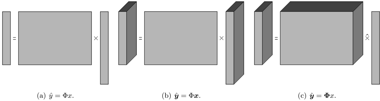
Fig. 2.1 – Comparaisons des modèles univarié/monocanal (a), multicanal (b) et multivarié (c). Dans (c), \hat{x} est considéré comme un produit élément par élément selon la dimension M .
