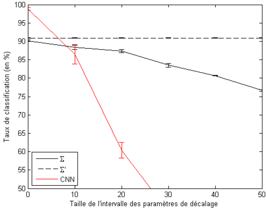
Fig. 6.6 – Taux de classification \bar{\eta}_{consist} sur les vecteurs de caractéristiques extraits des signaux tradatés aléatoirement par les fonctions de groupement \Sigma(\cdot) et \Sigma'(\cdot) , et pour le CNN.
