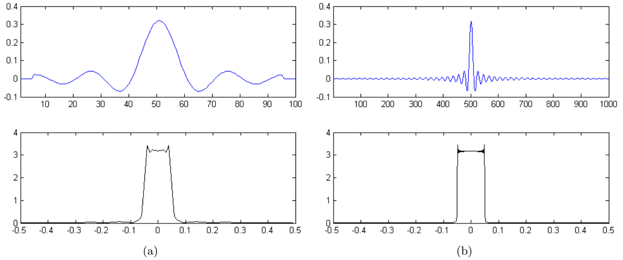
Fig. 1.10 – Noyaux de sinus cardinal (haut) et leurs spectres (bas) pour C = 0.1 , et de longueur N = 100 (a) et N = 1000 (b).
