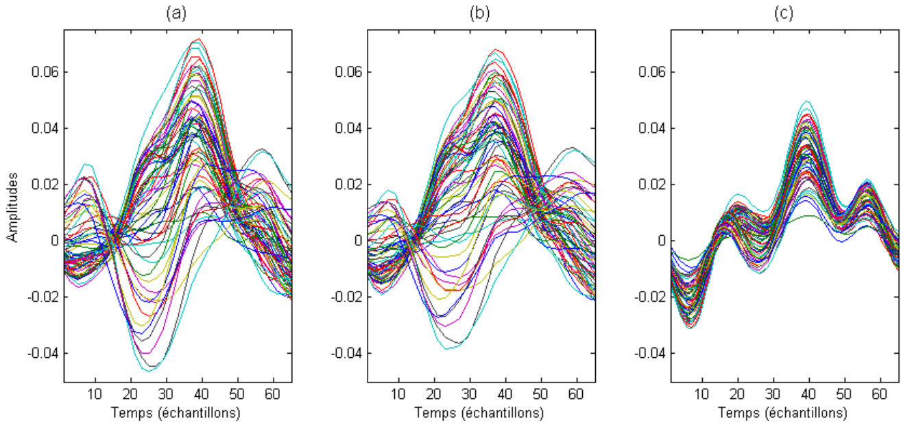
Fig. 2.12 – Motifs temporels multivariés du P300 calculés par grande moyenne (a), par moindres carrés (b) et par apprentissage de dictionnaire multivarié (c). Echantillonnées à 240 Hz, les amplitudes sont données en fonction des échantillons temporels.
