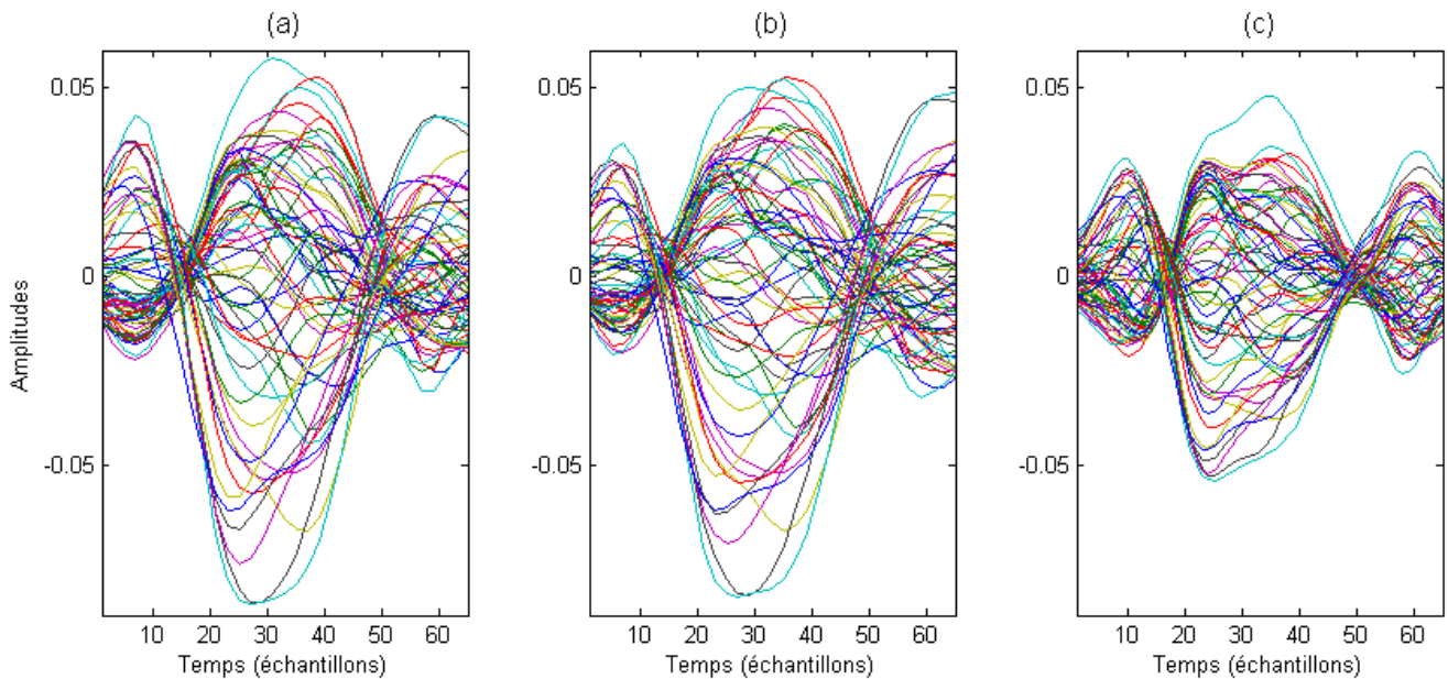
Fig. 2.16 – Motifs temporels multivariés du P300 calculés par grande moyenne (a), par moindres carrés (b) et par apprentissage de dictionnaire multivarié (c), pour la référence d'électrode moyenne.
