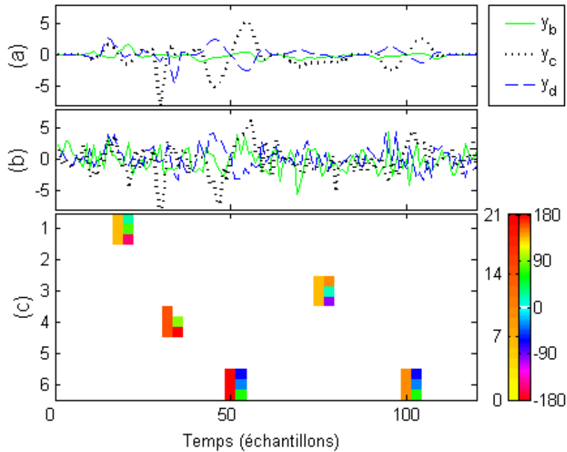
Fig. 3.1 – Signaux quaternioniques original (a) et bruité (b) (première partie imaginaire y_b représentée par un ligne verte pleine ; la seconde partie y_c par une ligne noire pointillée ; et la troisième partie y_d par une ligne traitillée bleue), et le spikegramme associé (c).
