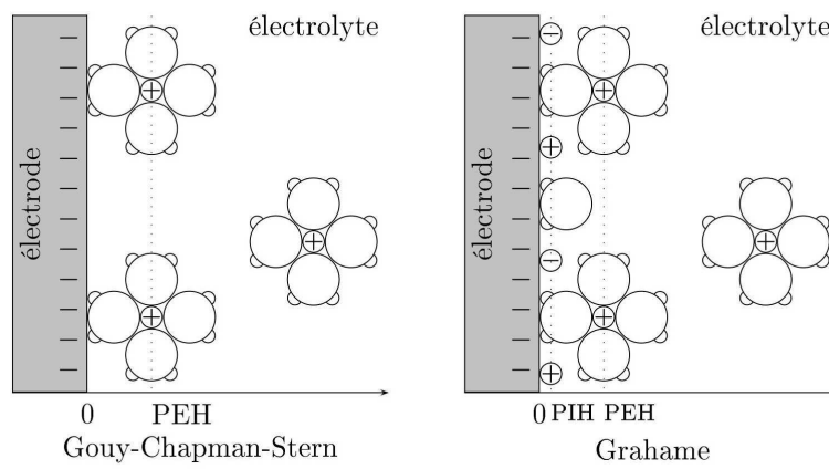
FIGURE 2.6 – Représentation de charges et d'ions selon les modèles de Stern et Grahame. PEH= Plan Externe de Helmholtz, PIH =Plan Interne de Helmholtz. [33]
