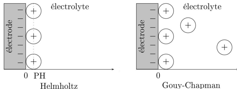
FIGURE 2.5 – Représentation de charges et d'ions selon les modèles de Helmholtz et Gouy-Chapman pour la double couche. PH= Plan de Helmholtz, [33]
