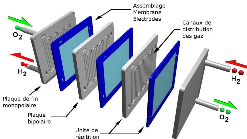
FIGURE 2.1 – Pile à combustible de type PEM alimentée en hydrogène et en oxygène
