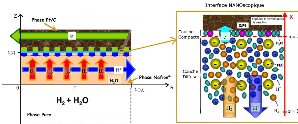
FIGURE 3.2 – À gauche, les échelles microscopiques du modèle d'A. Franco et l'emplacement du modèle nanoscopique en bleu clair, z = e_{NI} . À droite, l'échelle nanoscopique décrivant la double couche électrochimique, où x est la variable d'espace utilisée à cette échelle et L = 1 \text{ nm} représente l'épaisseur de la couche diffuse. Figure extraite de [37].
