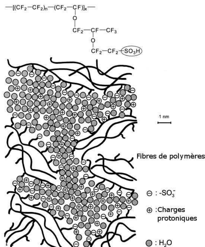
FIGURE 2.4 – Structure chimique de la membrane Nafion : chaque fibre est composée d'une chaîne de polymères organisées de manière que les groupements sulfonates soient disposés à l'extérieur de cœur de la fibre. Figure extraite de [57].
