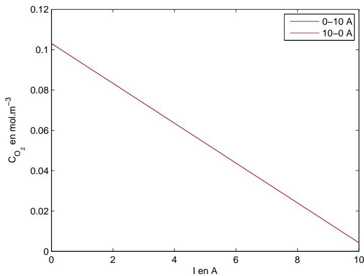
FIGURE 3.10 – Concentration d'oxygène à l'interface cathodique en fonction du courant
