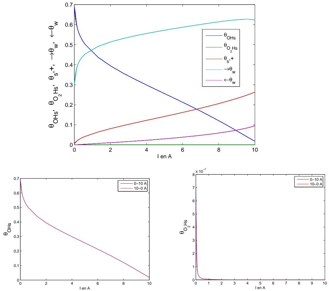
FIGURE 3.12 – Taux de recouvrement à la cathode en fonction du courant. \theta_{O_2Hs} prend des valeurs inférieures à 10^{-6} , invisibles sur la figure.
