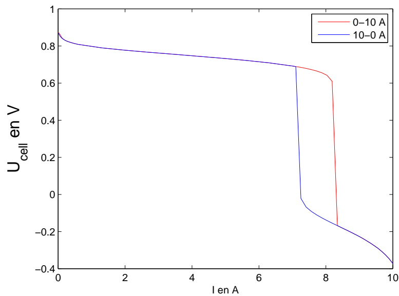
FIGURE 3.6 – Courbe de polarisation de la pile
