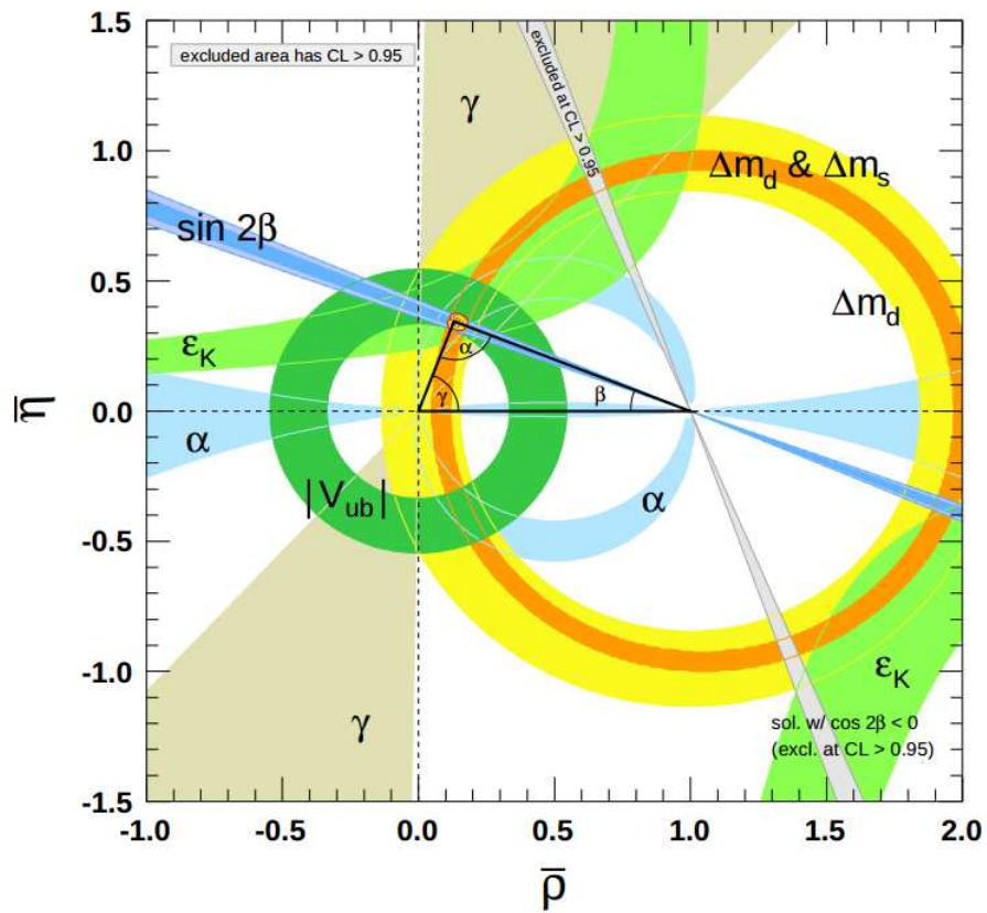
Figure B.2: Contraintes sur les paramètres \bar{\rho} = \rho(1 - \frac{\lambda^2}{2}) et \bar{\eta} = \eta(1 - \frac{\lambda^2}{2}) de la matrice CKM.
