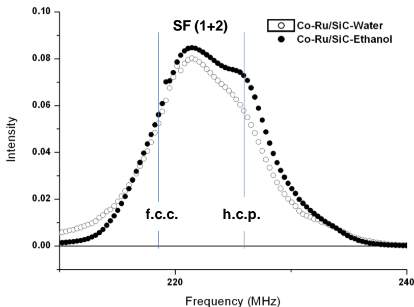
Figure 5. Spectres RMN 59 Co des catalyseurs Co-Ru/SiC-E et Co-Ru/SiC-W, enregistrés à 4.2 K, montrant la présence de plusieurs espèces de cobalt: Co (cfc), Co (hcp) ainsi que des fautes d'empilement (SF (1+2)) avec 56 \pm 1 % pour le Co-Ru/SiC-E et 52 \pm 1 % pour le Co-Ru/SiC-W.
