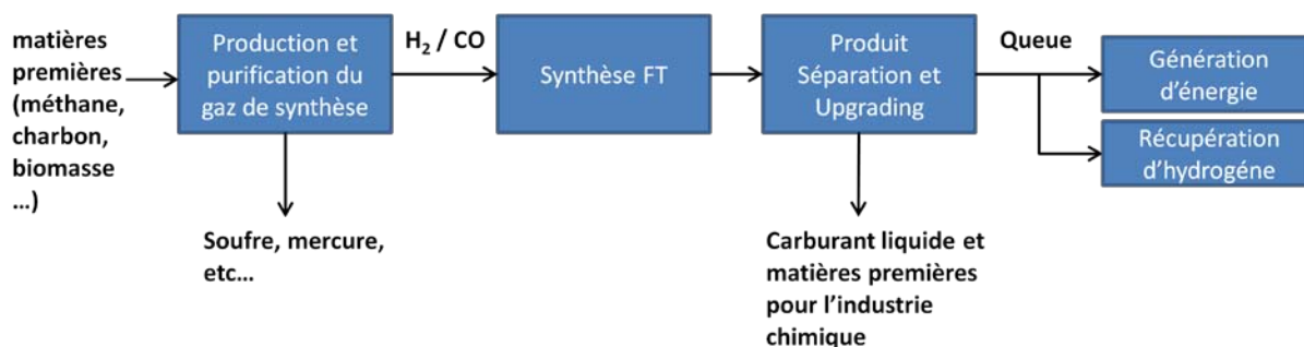
Figure 1. Schéma simplifié d'une unité XTL intégrant les différentes étapes du procédé
