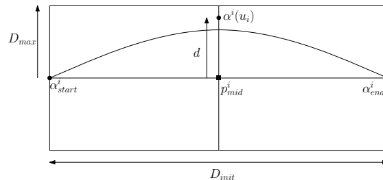
FIGURE 2.6 – Modélisation de trajectoire par approximation B-spline
