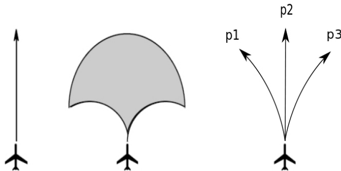
FIGURE 1.5 – Approches nominale, pire cas et probabiliste de la prédiction de trajectoire
