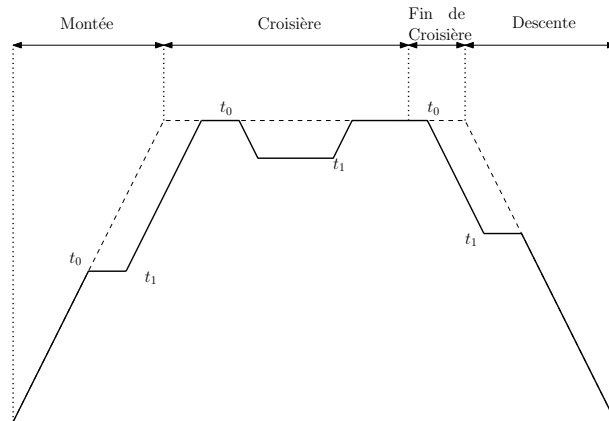
FIGURE 1.11 – Manœuvres utilisées dans le plan vertical
