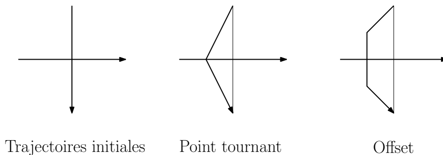
FIGURE 1.4 – Deux types de manœuvres horizontales
