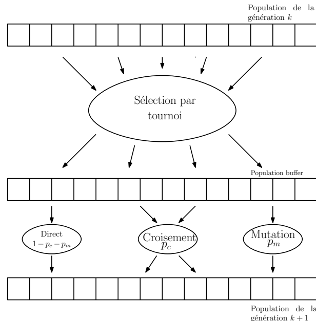
FIGURE 3.1 – Processus d'évolution de la génération k à la génération k + 1 durant l'AG
