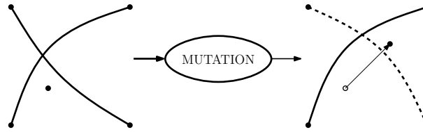
FIGURE 3.7 – Trajectoires correspondant à un chromosome avant et après mutation (déplacement du point de contrôle d'une des trajectoires)
