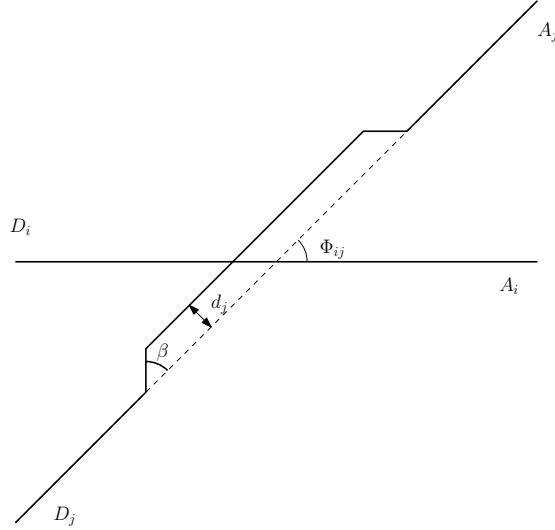
FIGURE 1.12 – Conflit à deux avions et manœuvres de résolution
