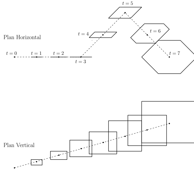
FIGURE 1.9 – Modélisation de l'incertitude sur la position de l'avion dans les plans horizontal et vertical
