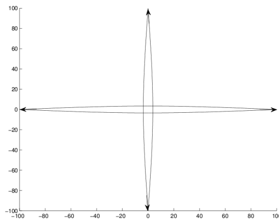
FIGURE 4.15 – Trajectoires obtenues par résolution par AG
