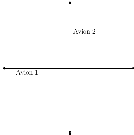
FIGURE 4.5 – Croisement de deux avions à 90^\circ
