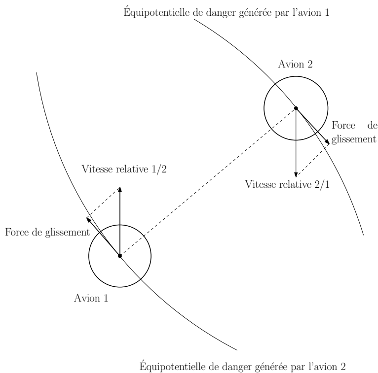
FIGURE 1.7 – Forces de glissement coordonnées entre deux avions
