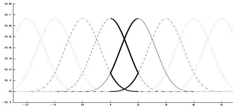
FIGURE 2.5 – Les 4 fonctions de base impliquées dans le calcul de l'approximation dans l'intervalle [1, 2]
