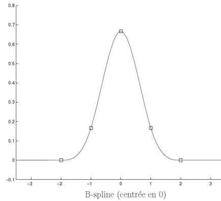
FIGURE 2.4 – Fonction de base B_0 centrée en le nœud 0
