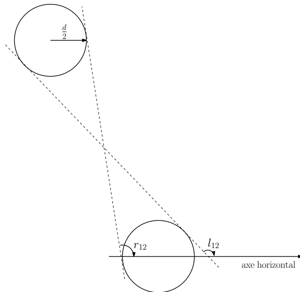
FIGURE 1.13 – Situation à deux avions et angles associés
