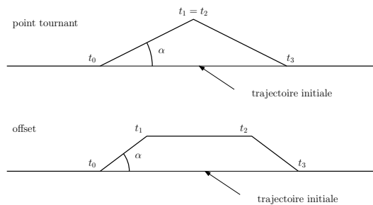
FIGURE 1.10 – Manœuvres utilisées dans le plan horizontal et variables d'optimisation
