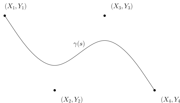
FIGURE 2.3 – Exemple d'approximation de 4 points de contrôles du plan par la B-spline \gamma paramétrée par s
