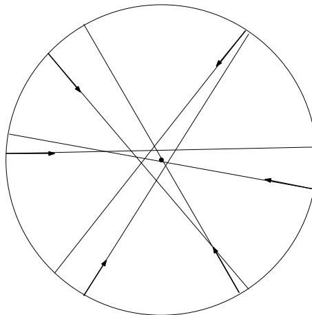
FIGURE 4.21 – Exemple de situation aléatoire pour N = 6 avion
