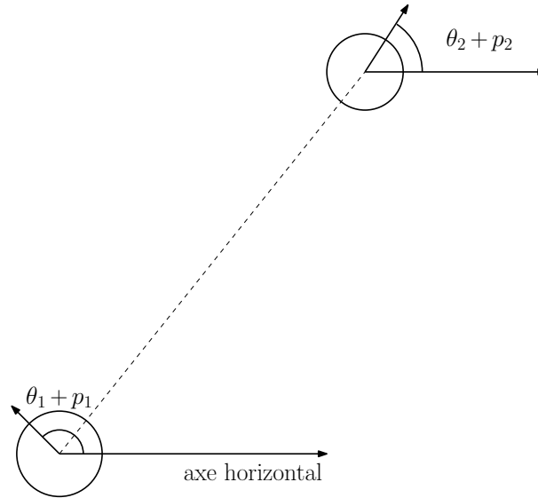
FIGURE 1.14 – Situation à deux avions et changements de direction associés
