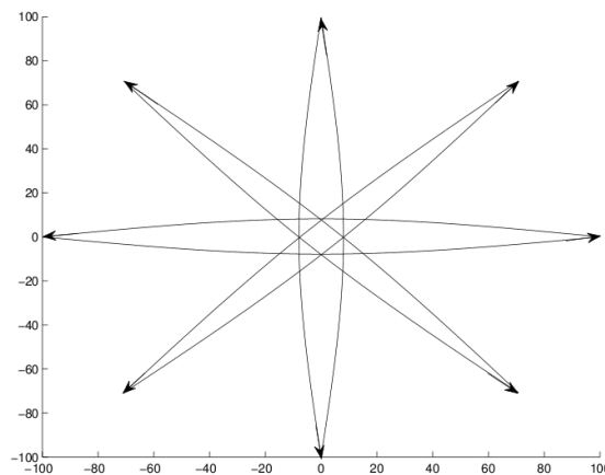
FIGURE 4.20 – Solution optimale obtenue par méthode de points intérieurs démarrant d'un bon point de départ
