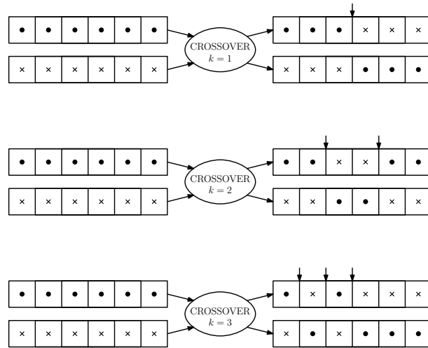
FIGURE 3.5 – Slicing crossover à k points, pour k = 1, 2, 3
