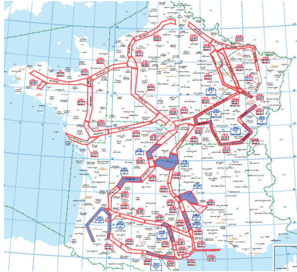
FIGURE 1.2 – Carte des routes aériennes sur la France
