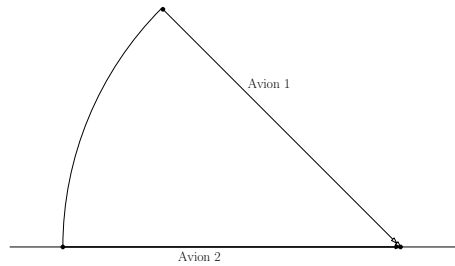
FIGURE 4.8 – Fusion des routes de deux avions
