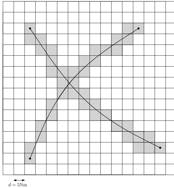
FIGURE 3.3 – Discretisation de l'espace pour une situation à 2 avions
