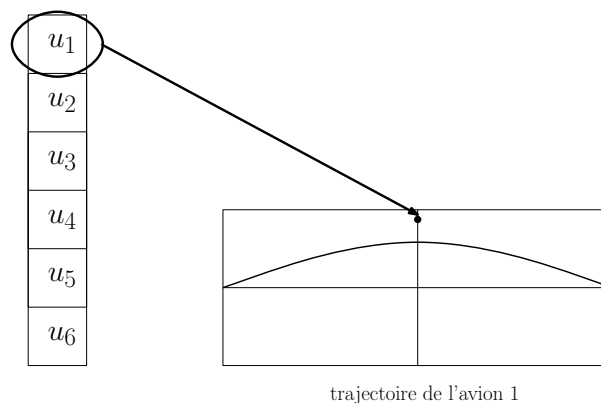
FIGURE 3.2 – Encodage d'un chromosome pour une situation à N = 6 avions
