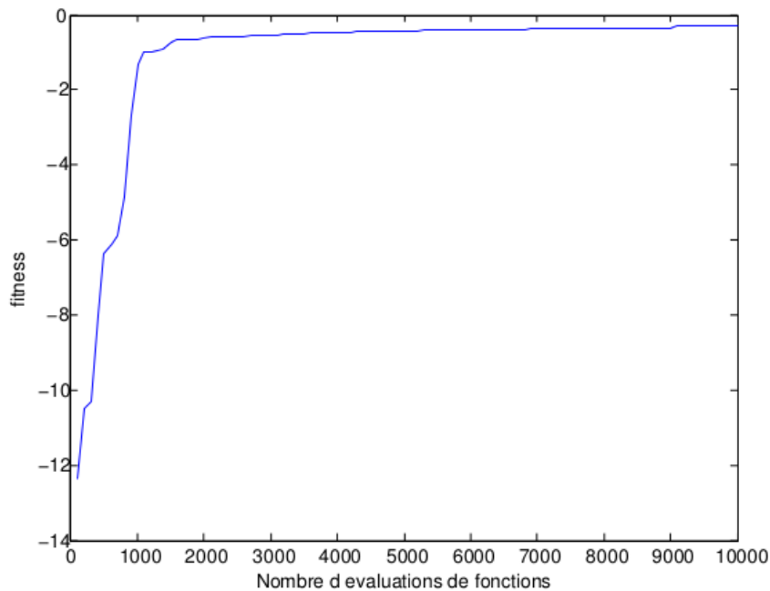
FIGURE 4.1 – Évolution de la fitness par rapport au nombre d'évaluations de fonctions pour le problème du rond-point à N = 8 avions
