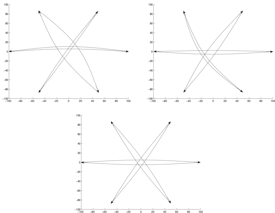
FIGURE 4.18 – Trajectoires obtenues par résolution par méthode locale des points intérieurs avec deux points de départ de la recherche différents
