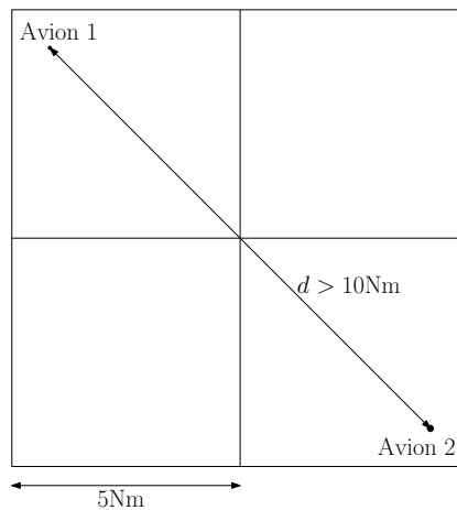
FIGURE 3.4 – Deux avions considérés à tort en conflit
