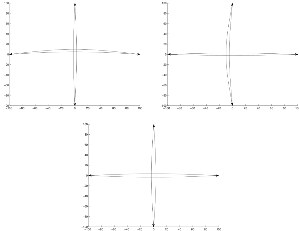
FIGURE 4.16 – Trajectoires obtenues par méthode locale des points intérieurs avec deux points de départ différents
