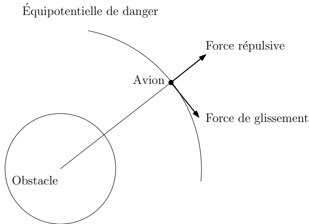
FIGURE 1.6 – Forces exercées par un obstacle sur un avion
