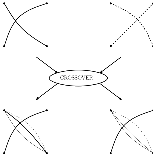
FIGURE 3.6 – Trajectoires correspondant aux parents (en haut) et aux enfants issus d'un croisement barycentrique (en bas)
