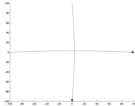
FIGURE 4.6 – Trajectoires obtenues par AG
