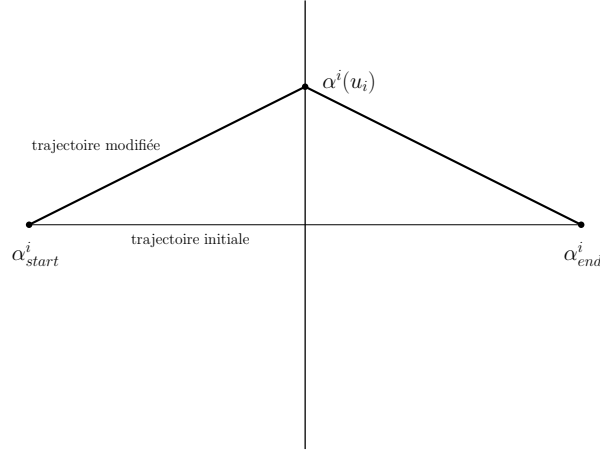
FIGURE 2.1 – Modélisation de trajectoire linéaire par morceaux avec point tournant
