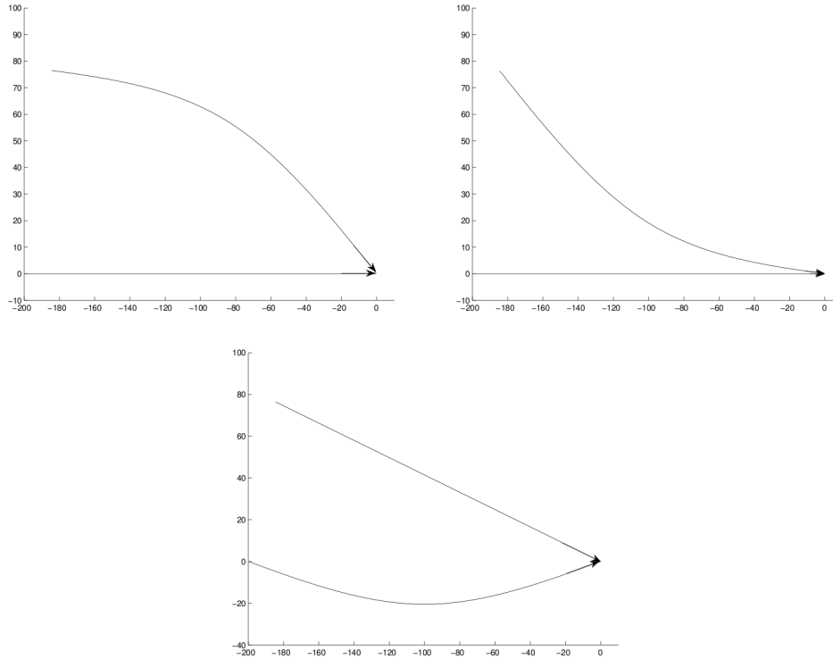
FIGURE 4.10 – Trajectoires obtenues par méthode locale de points intérieurs avec trois points de départ différents
