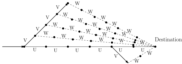
FIGURE 1.8 – Exemple de mouvements dans le graphe pour une trajectoire
