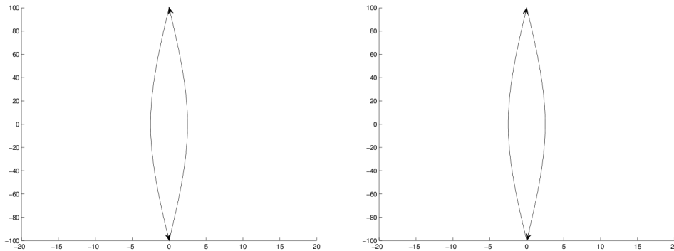
FIGURE 4.4 – Trajectoires obtenues par méthode locale des points intérieurs avec deux points de départ différents
