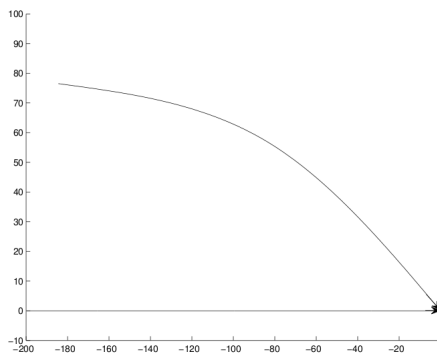
FIGURE 4.9 – Trajectoires obtenues par AG
