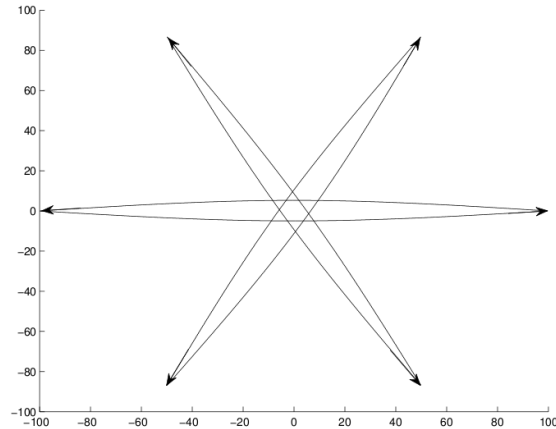
FIGURE 4.17 – Trajectoires obtenues par AG
