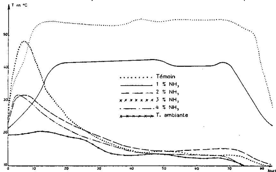
Figure 35 : Courbes de température des balles témoin et traitées (humidité =34 %)
