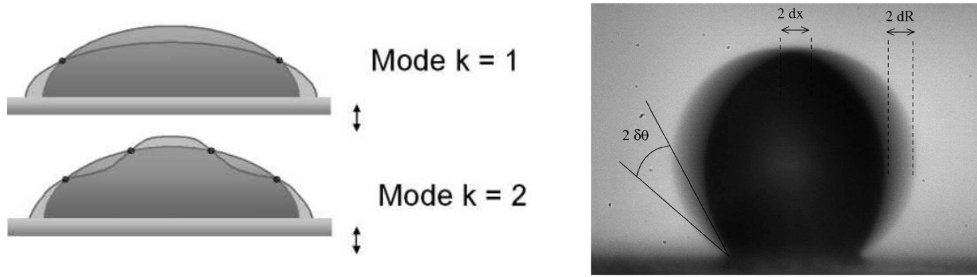
FIGURE I.8 – Gauche : mode "pumping", tiré de [36]. Droite : mode "rocking", tiré de [39]
