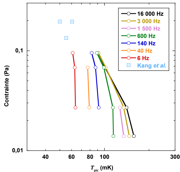
FIGURE 3.20 – La température de transition T_{pic} est donnée en fonction de la contrainte \sigma = \mu\varepsilon . La contrainte est calculée avec la valeur du module de cisaillement à la température T_{pic} , c'est à dire environ au milieu de la transition. Les trois points au-dessus de 0,1 Pa proviennent de Kang et al. [135] dans une région qu'ils considèrent comme une transition entre des dislocations totalement piégées et partiellement piégées.
