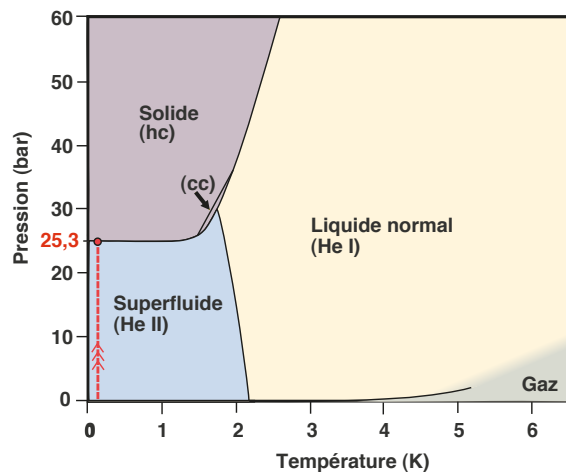
FIGURE 2.32 – Diagramme de phases ( P, T ) de {}^4\text{He} . La ligne rouge représente le chemin suivi pour la croissance de cristaux de "type 1". Le point rouge correspond au point où la mesure est réalisée.
