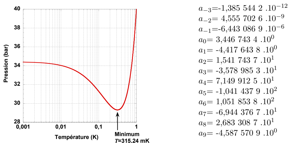
FIGURE 2.8 – À gauche, la courbe de fusion de ^3\text{He} selon l'équation de la PLTS-2000 dont les coefficients sont donnés à droite
