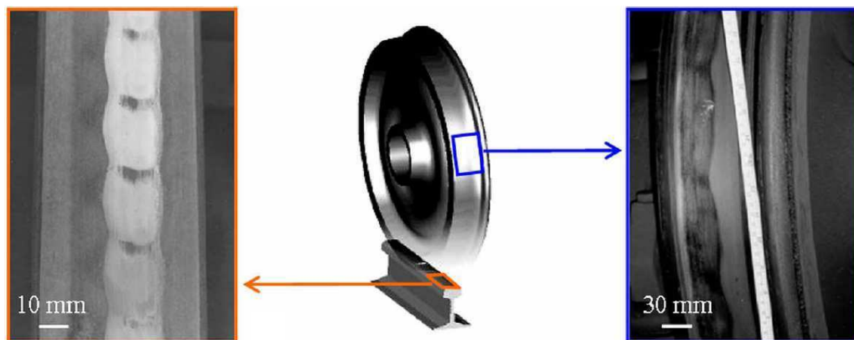
FIGURE 3.1 – Roue et rail déformés par usure ondulatoire. À gauche, photographie d'un rail de train sur lequel on aperçoit le motif créé par l'usure ondulatoire, à droite, photographie de la roue usée par le rail déformé. D'après (Saulot [2006]).
