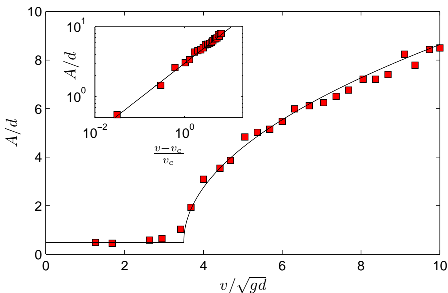
FIGURE 2.13 – Diagramme de bifurcation dans les simulations numériques. On observe ici aussi une bifurcation semblable à une bifurcation super-critique. Le graphe dans l'encadré, correspond à l'amplitude des rides en fonction de l'écart au seuil en échelle logarithmique, cette amplitude peut être modélisée par une droite de pente 1/2 symbolisée par la courbe en trait noir.
