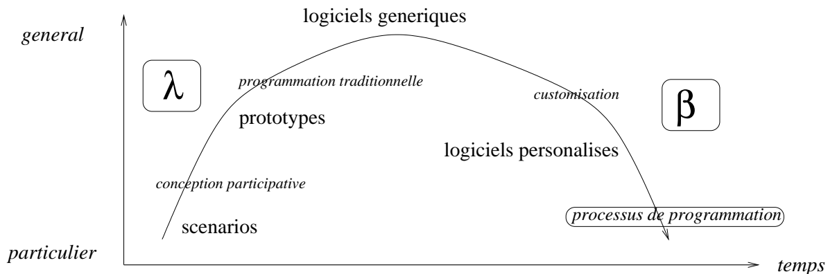
FIG. 1.6 – Généralisation/spécialisation.
