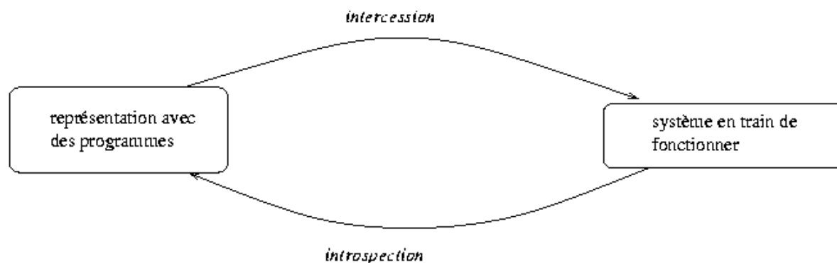
FIG. 3.3 – Causalité.
