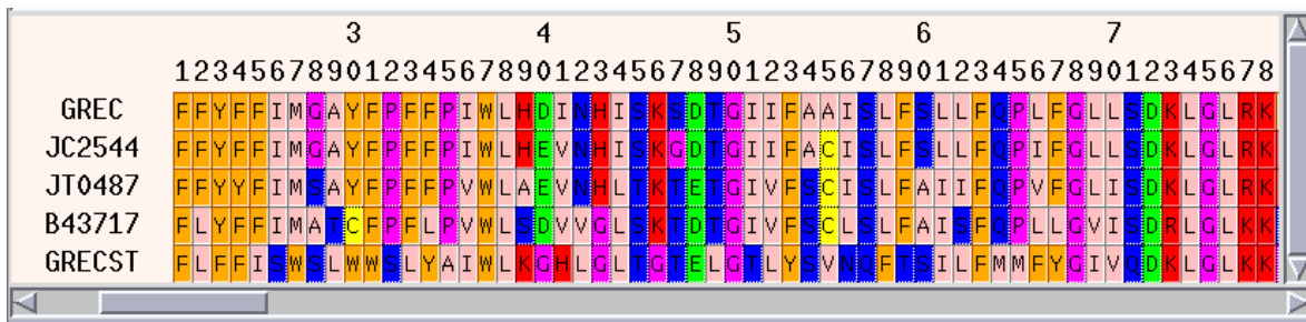
FIG. 5.7 – Éditeur d'alignement.
