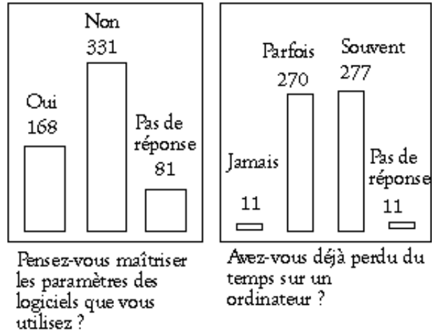
FIG. 2.6 – Les problèmes
