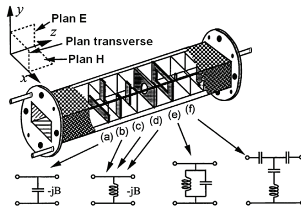
Figure 4-8 : Différentes formes d'iris dans un guide d'ondes rectangulaire et leurs circuits équivalents respectifs
