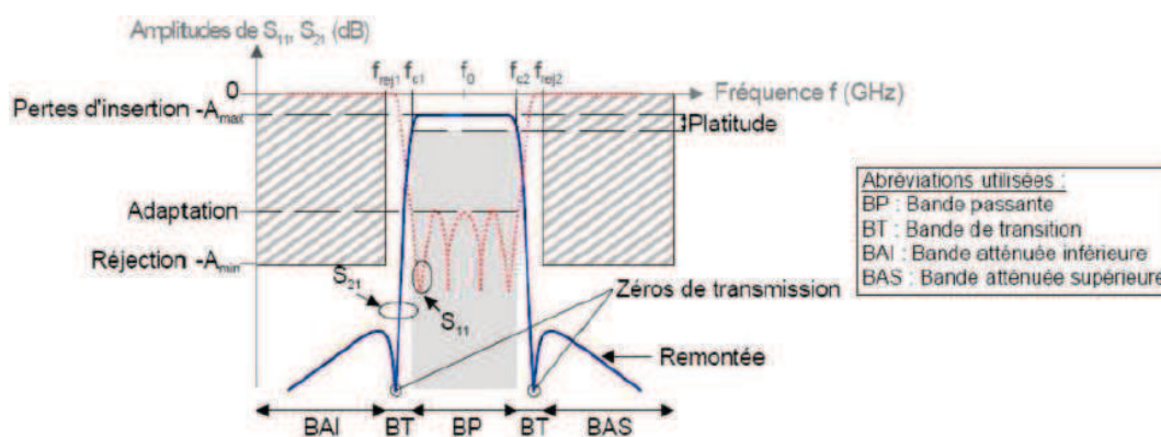
Figure 1-2: Gabarit et réponse électrique d'un filtre passe-bande
