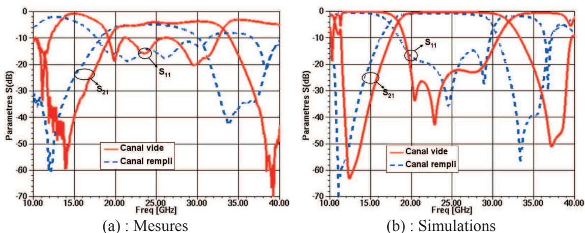
Figure 3-18 : Performances mesurées (a) et simulées (b) du filtre (premier wafer)
