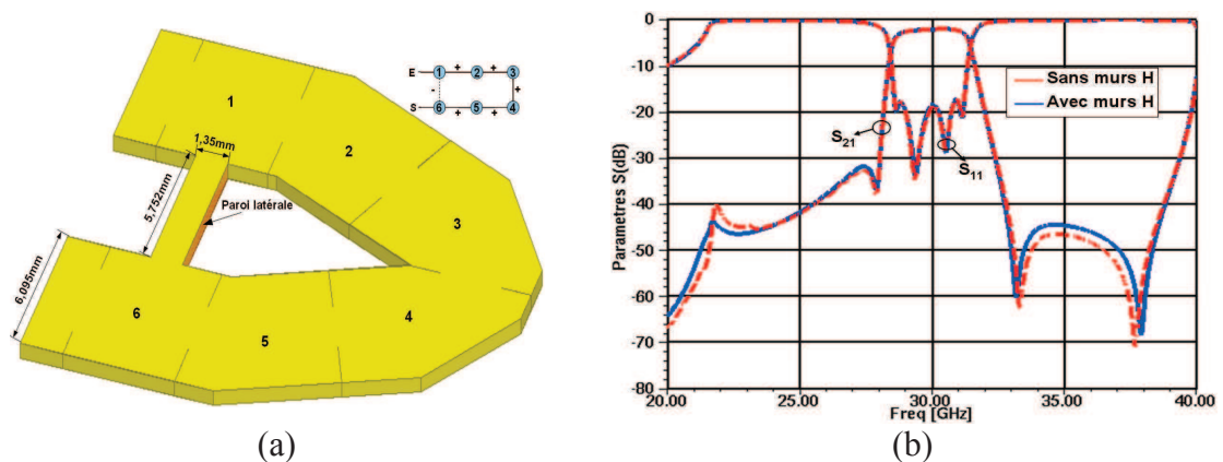
Figure 4-31 : (a) Filtre SIW à iris d'ordre 6 replié et (b) performances électriques simulées avec couplage par guide
