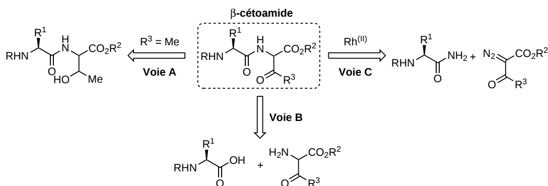
SCHÉMA 1.7 – Synthèse des précurseurs \beta -cétoamide et \beta -cétothioamide
