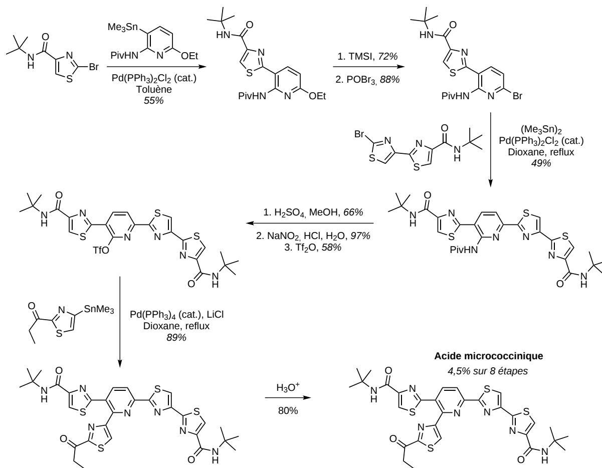
SCHÉMA 1.32 – Aménagement pas-à-pas d'un précurseur pyridinique pour la synthèse de l'acide micrococcinique
