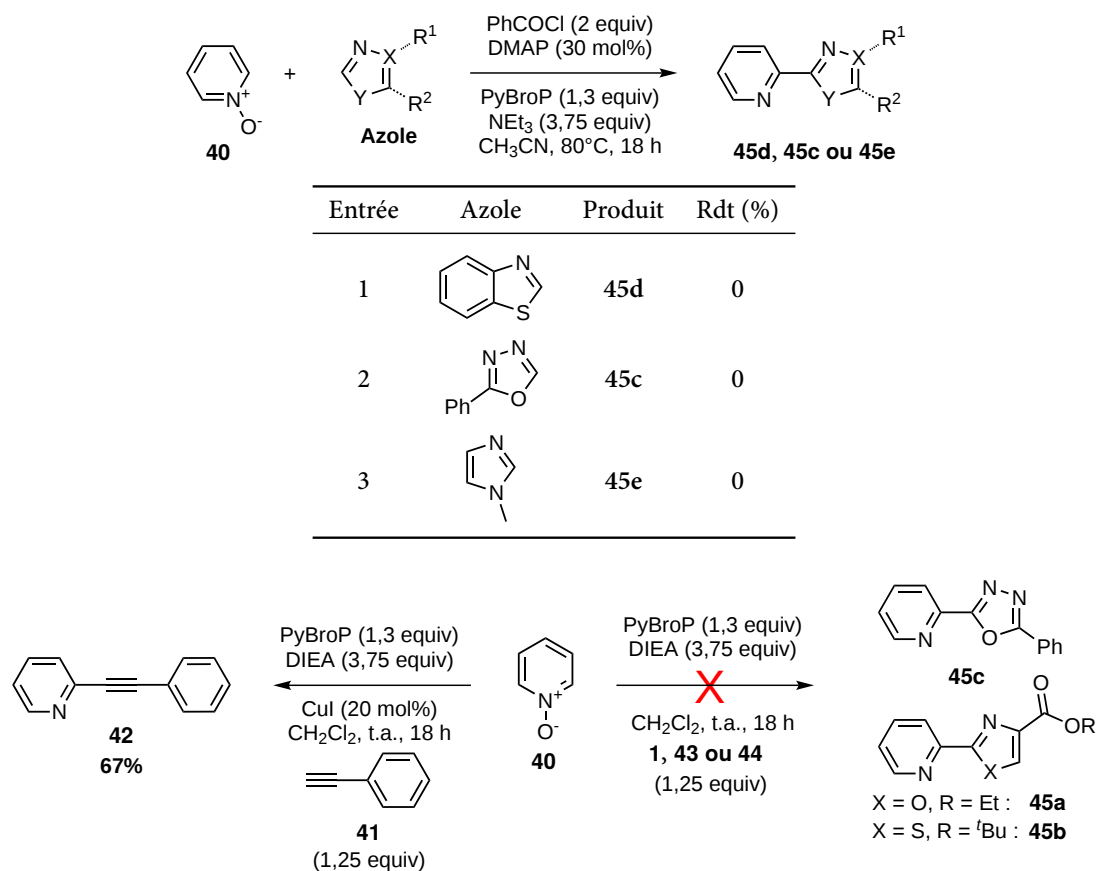
SCHEMA 3.17 – Addition du phénylacétylène en position C 2 de la pyridine N -oxyde activée par le PyBroP, et premiers essais d'introduction directe de 1,3-diazoles sur la pyridine N -oxyde activée par le PyBroP
