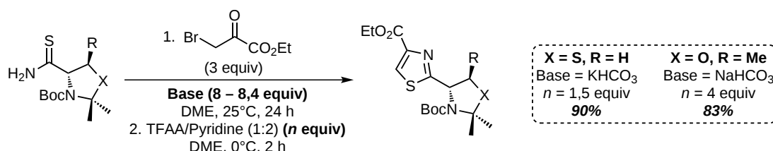
SCHÉMA 1.14 – Modification de la méthode de HOLZAPFEL proposée par NICOLAOU au cours de la synthèse du thiostrepton
