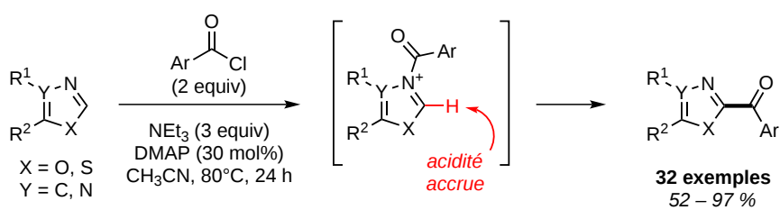
SCHÉMA 3.18 – Développement d'une méthodologie générale d'arylation en séries (benz)oxazole, (benzo)thiazole et 1,3,4-oxadiazole
