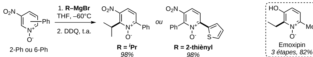
(b) Réactivité des 3-nitropyridines
