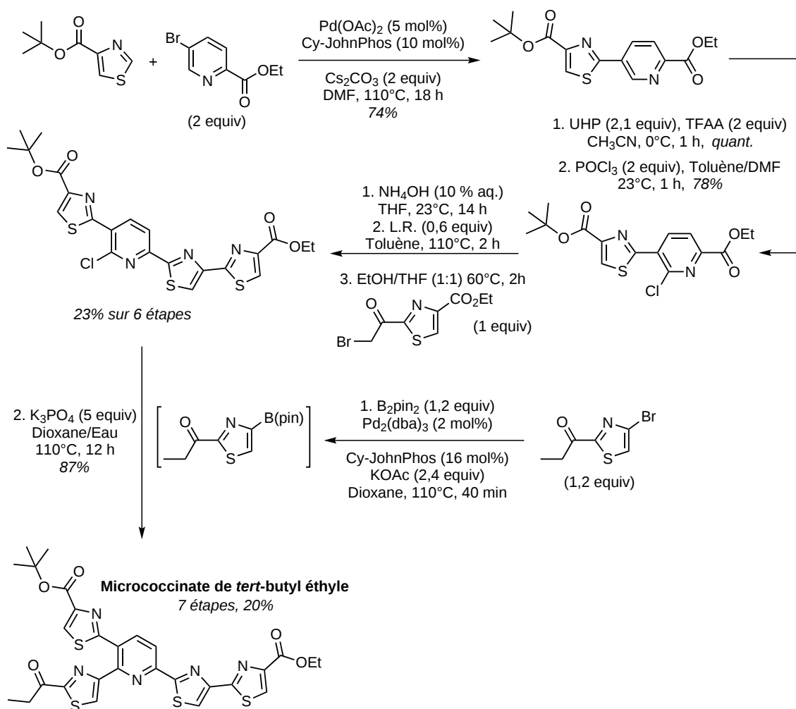
SCHÉMA 1.43 – Application de la méthodologie BSC à la préparation du micrococcinate de tert -butyl éthyle
