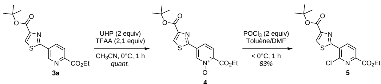
SCHÉMA 2.3 – Synthèse du 6-chloro-5-thiazolylpicolinate d'éthyle 5
