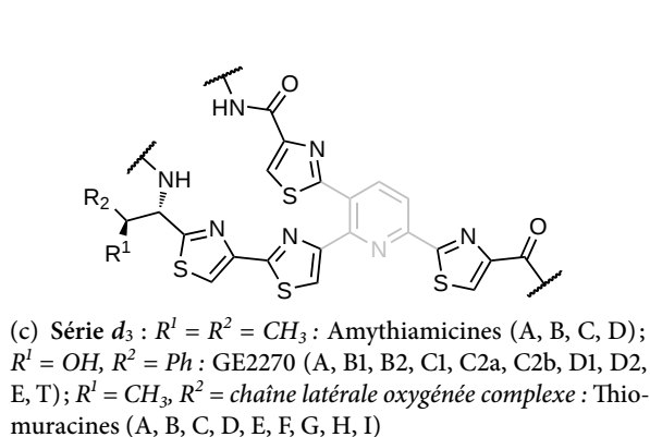
FIGURE 1.5 – Structures des cœurs des thiopeptides de la série d
