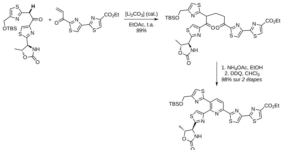
SCHÉMA 1.22 – Première synthèse du cœur de la micrococcine P1 par condensation, proposée par CIUFOLINI et son équipe
