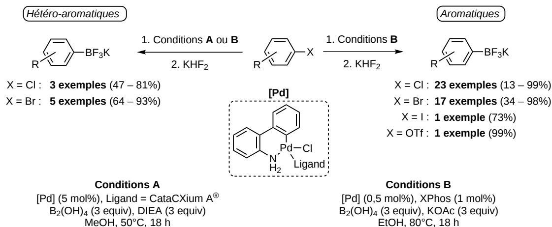
SCHÉMA 2.15 – Généralisation de l'utilisation de (tétrahydroxy)diborane et première application aux hétéroaromatiques
