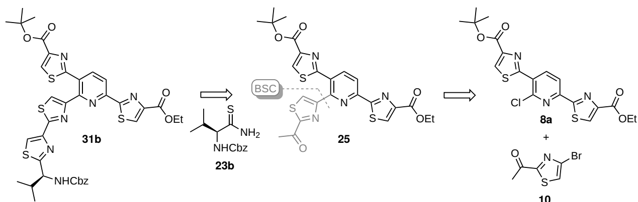
SCHÉMA 2.26 – Rétrosynthèse envisagée pour l'accès à la trithiazolypyridine 25
