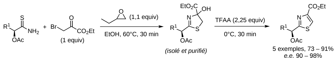
SCHÉMA 1.12 – Préparation des α-hydroxyméthyle-thiazoles proposée par SCHMIDT
