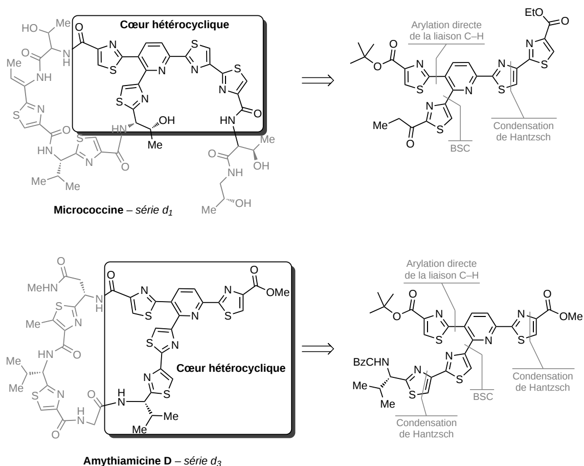
SCHÉMA 4.1 – Déconnexions clés employées lors de la synthèse du micrococcinate de tert -butyl éthyle (série d 1 ), étendues à la préparation des cœurs de type d 3
