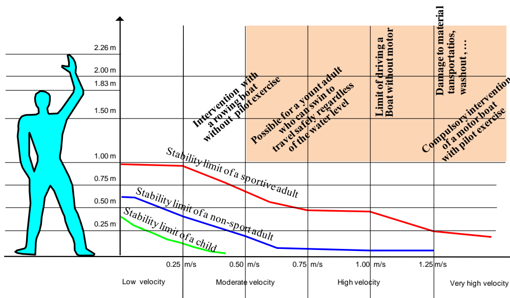
Figure III-19 Stability limits in water according to Direction départementale de l'équipement (DDE) du Vaucluse/DDE94 (Source : P.R.R.I.-Val-de-Marne, 2007, p23)
