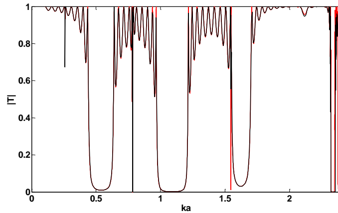
Figure 6-19 : coefficients de transmission par 10 réseaux linéaires identiques obtenus avec avec la méthode de diffusion multiple, les calculs numériques étant effectués sous FORTRAN (tracé rouge) et avec COMSOL (tracé noir)
