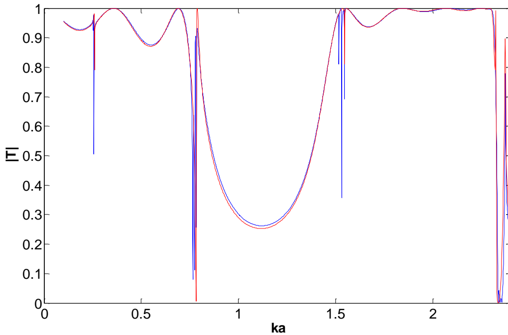
Figure 4-11: Coefficients de transmission d'une SP2D de 3 réseaux identiques dont tous les tubes ont la même masse volumique \rho = 7900\text{kg/m}^3 (rouge) et d'une SP2D de 3 réseaux linéaires dont les masses volumiques varient de l'un à l'autre \rho = 7900, 7500, 7100\text{kg/m}^3 (bleu),
