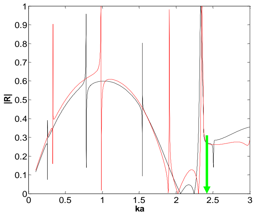
Figure 4-1 : Coefficients de réflexion d'un seul réseau de tubes b/a = 75/85 (noir), b/a = 73/85 (rouge). Ordre de diffraction 0.
