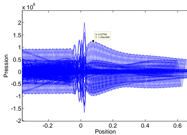
Figure 6-29 : pression de l'onde incidente, diffractée dans le réseau et diffusée en fonction de la variable Y. Le carreau indique la position de la tâche de focalisation
