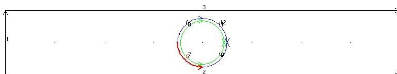
Figure 6-9 : réglages des conditions de frontière dans le sous-domaine solide
