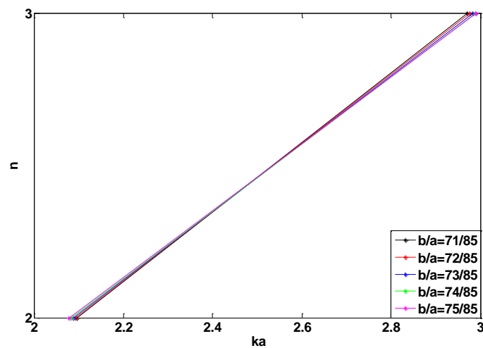
Figure 1-16 : trajectoire de Regge de la série l = 1 pour b/a variant de 71/85 à 75/85. Zoom de la figure précédente entre n = 2 et n = 3 .
