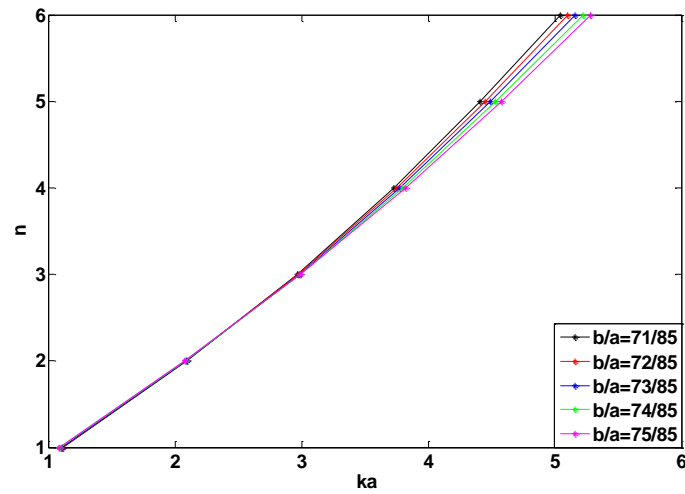
Figure 1-15 : trajectoire de Regge de la série l = 1 du tube en polyéthylène pour b/a variant de 71/85 à 75/85.
